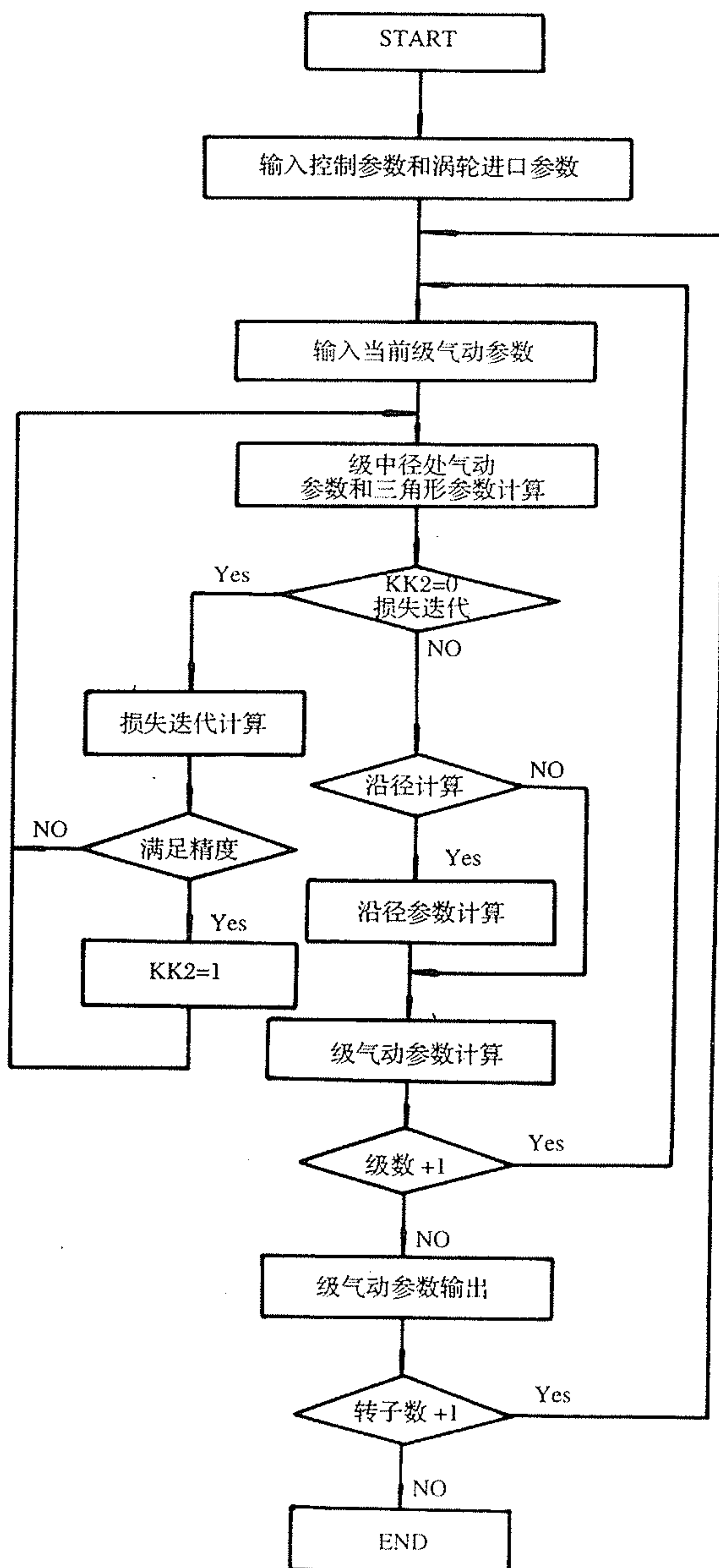
图 2-17 一维多方案设计计算流程图
