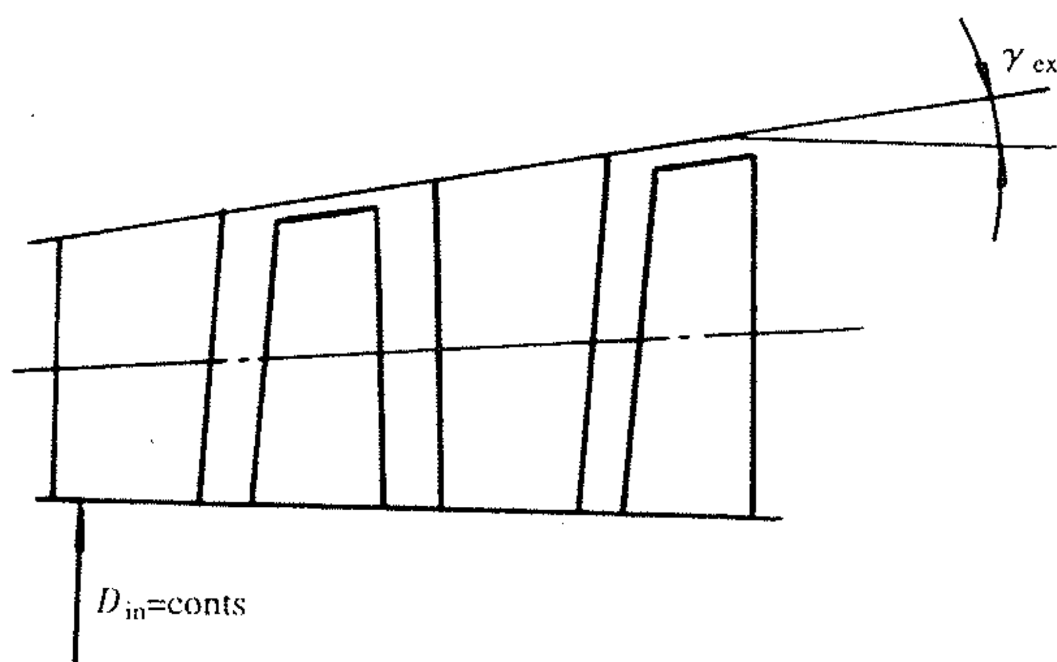
图 3-12 等内径流道
