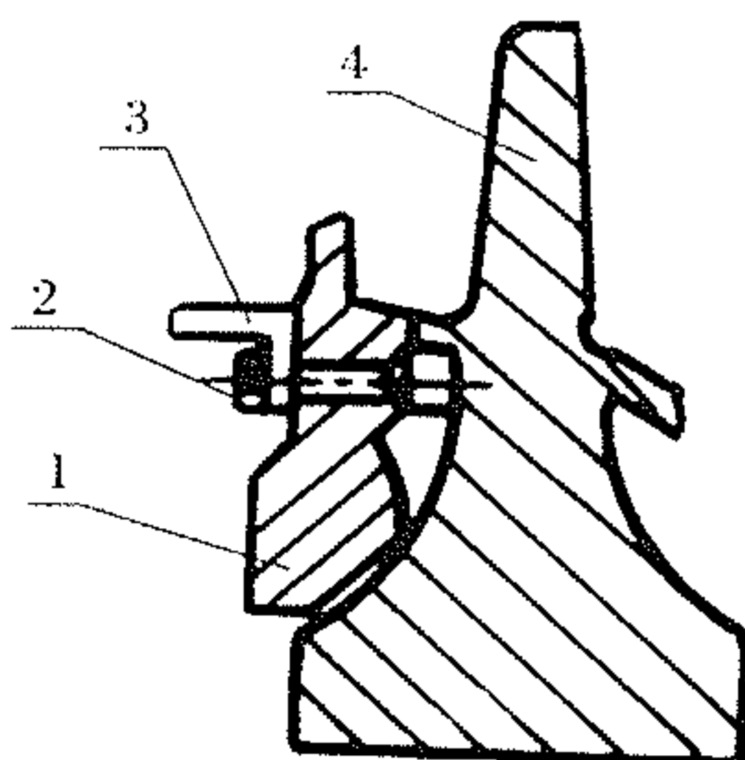
图 10-4 CFM56-5 高压涡轮转子
