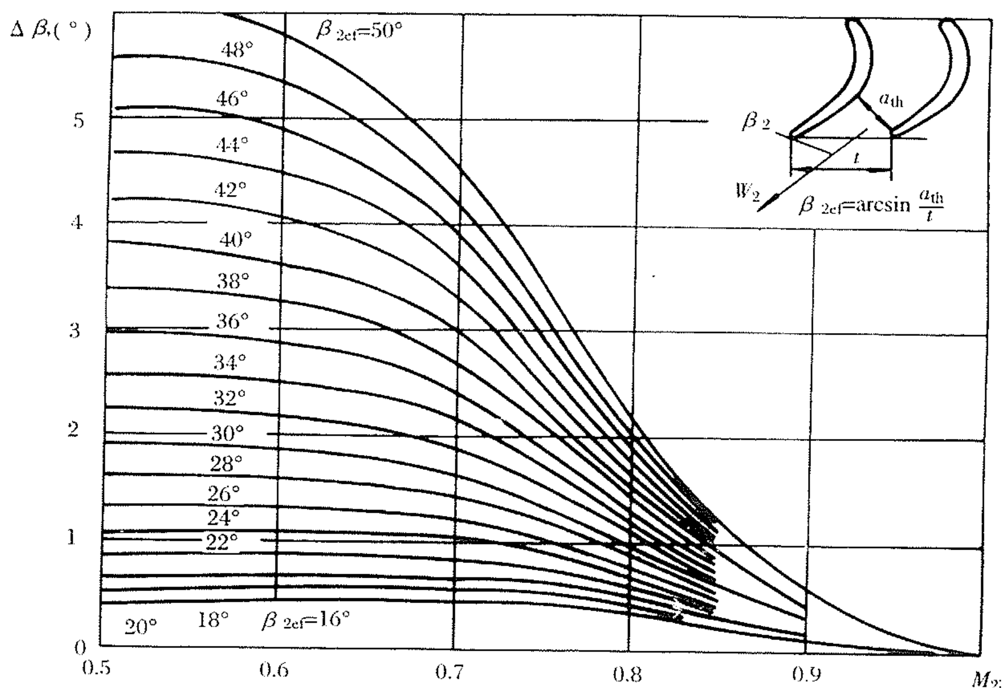
图 3-30 落后角曲线
