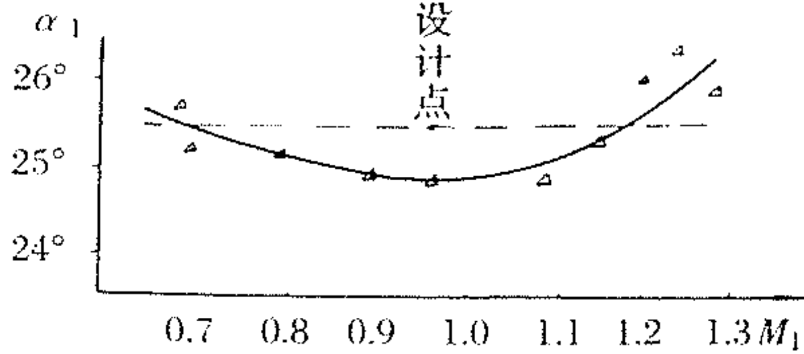
图 13-3 平面叶栅 \alpha_1 = f(M_1) 曲线
