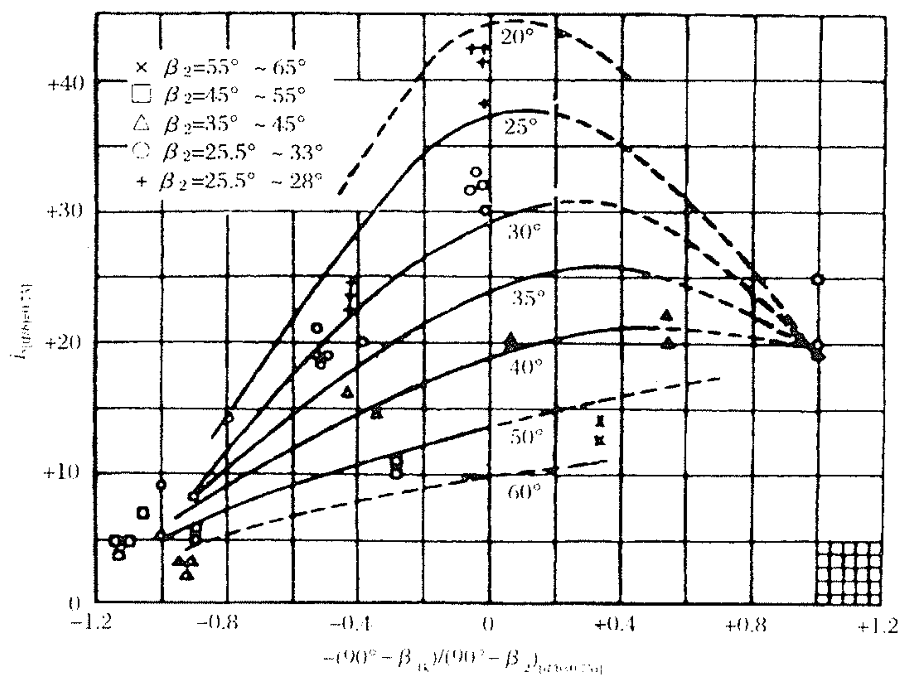
图 3-25 失速攻角 i_{s[(t/b)=0.75]} 随相对栅距的变化
