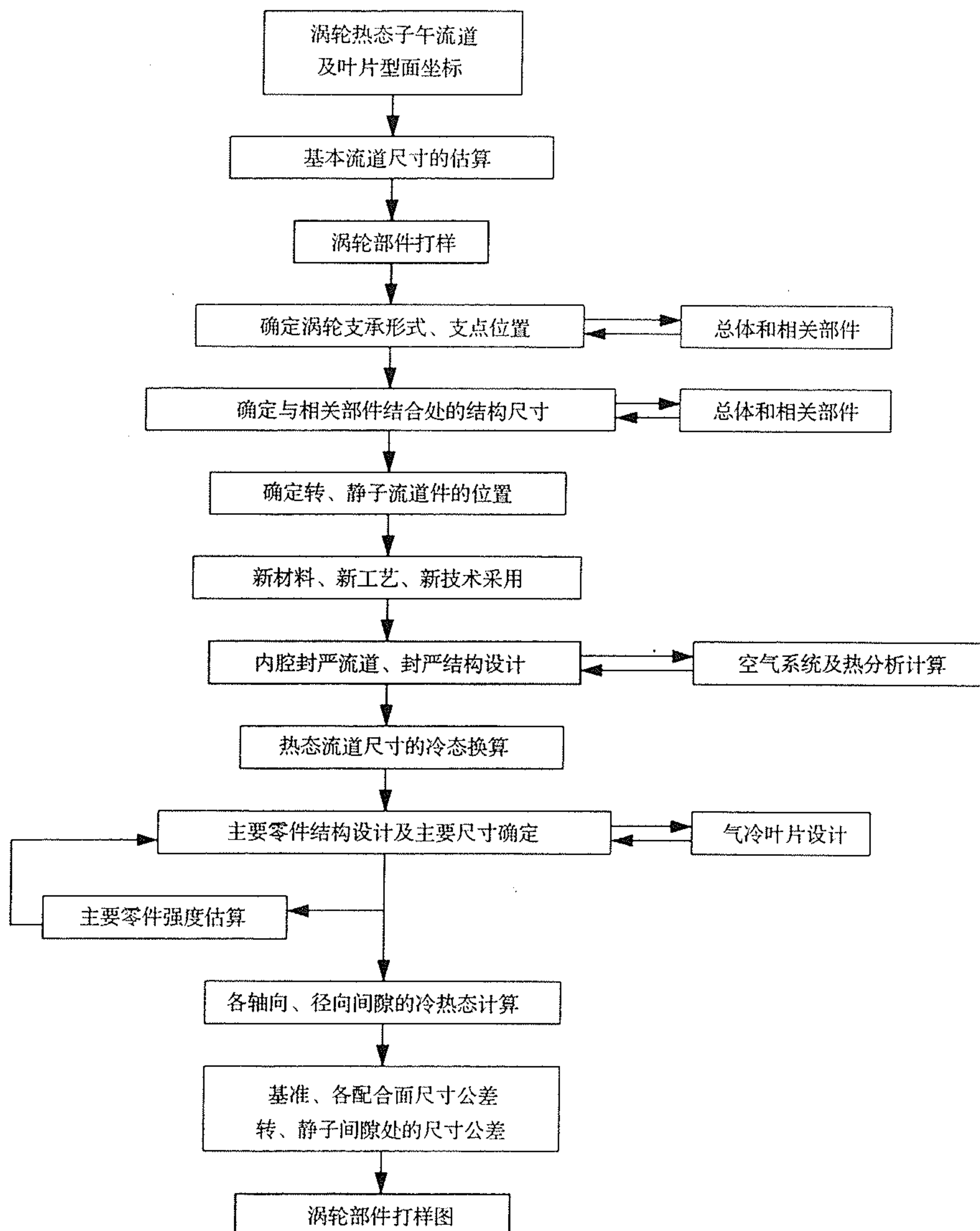
图 1-6 涡轮结构设计流程
