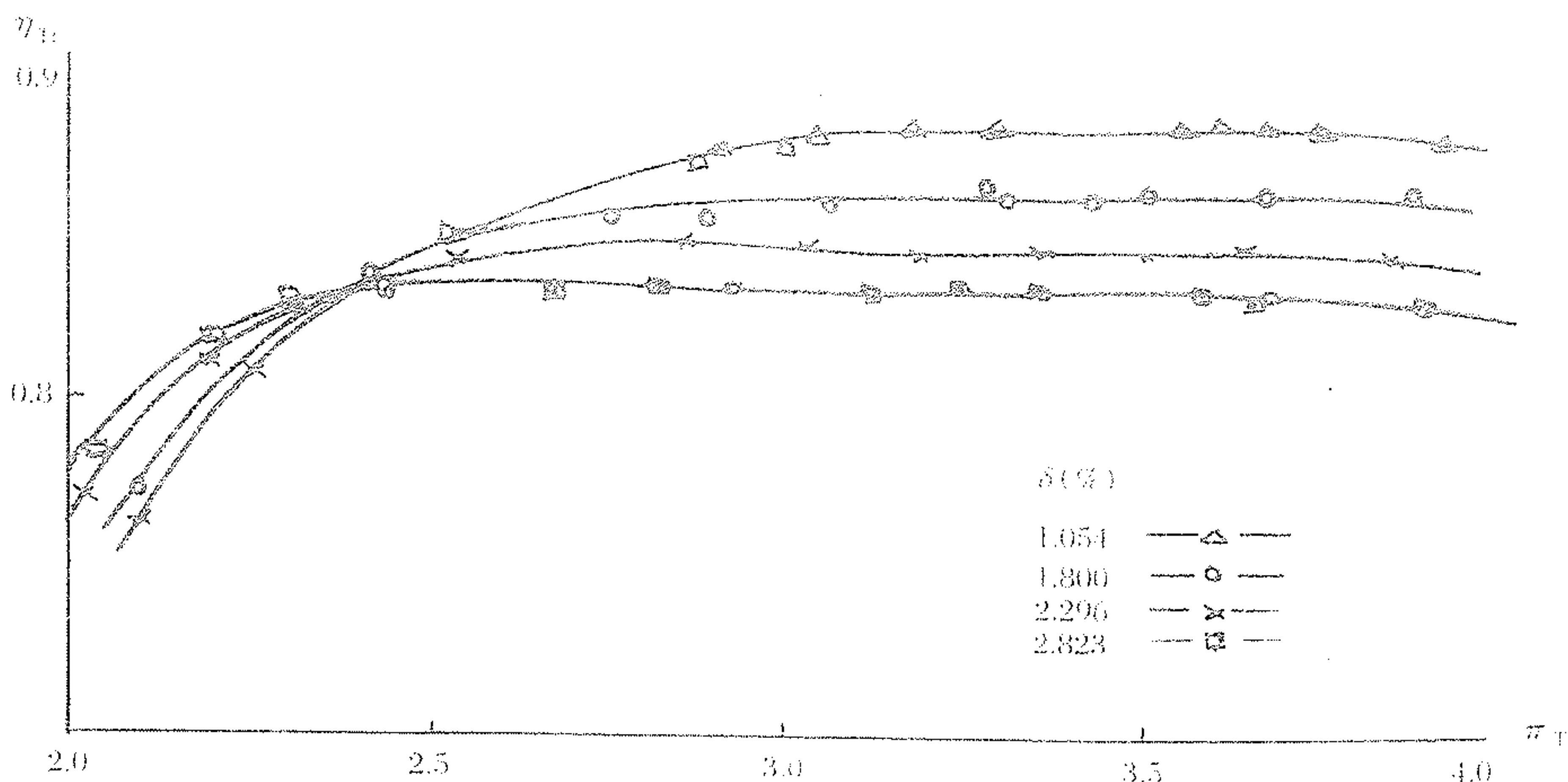
图 13-20 效率随 \bar{\delta} 的变化曲线
