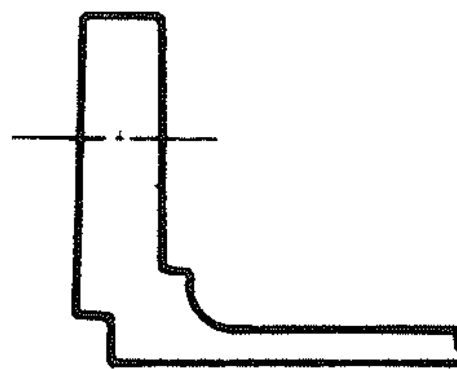
图 11-28 “危险”截面处加厚
