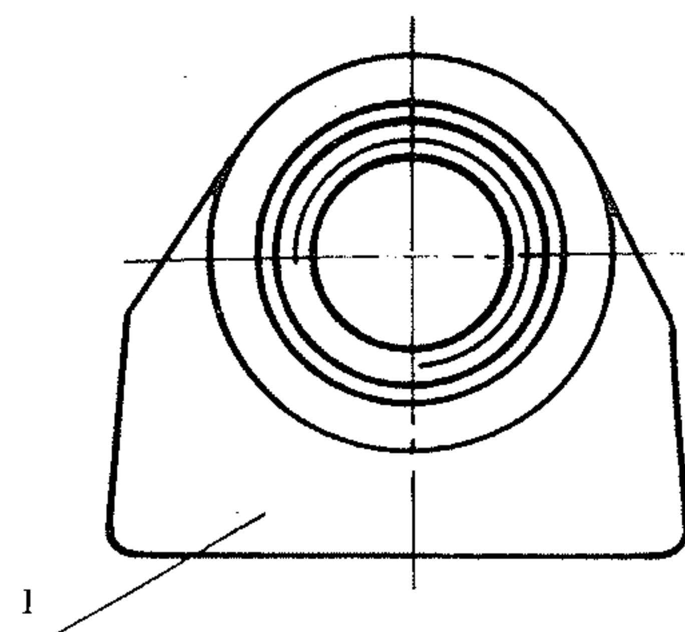
图 10-10 托板自锁铆轴螺母 1—托板;2—螺母;3—铆轴
