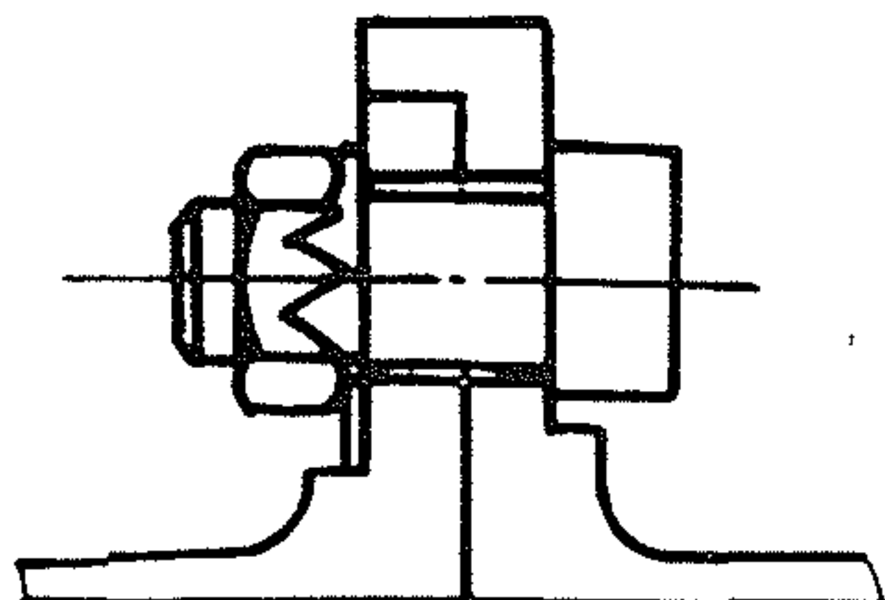
图 11-36 外止口结构示意图
