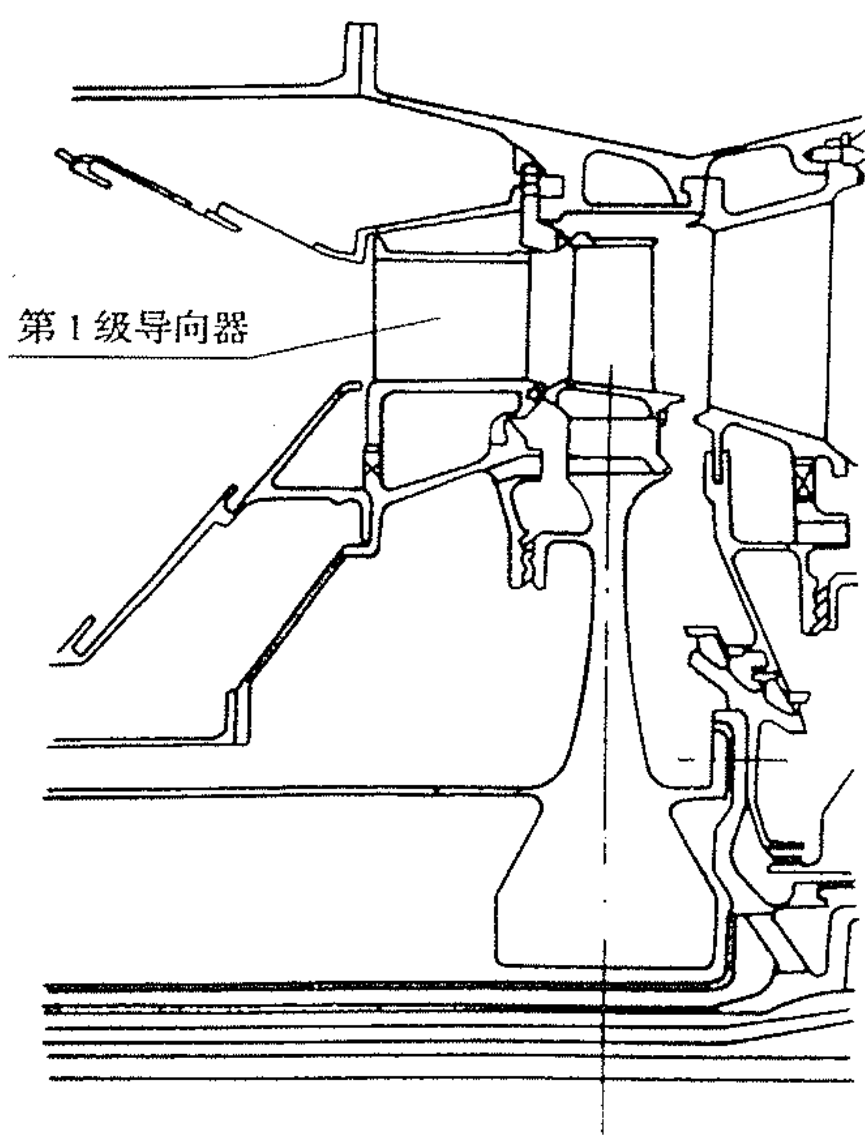
图 11-6 RB199 高压涡轮第 1 级导向器
