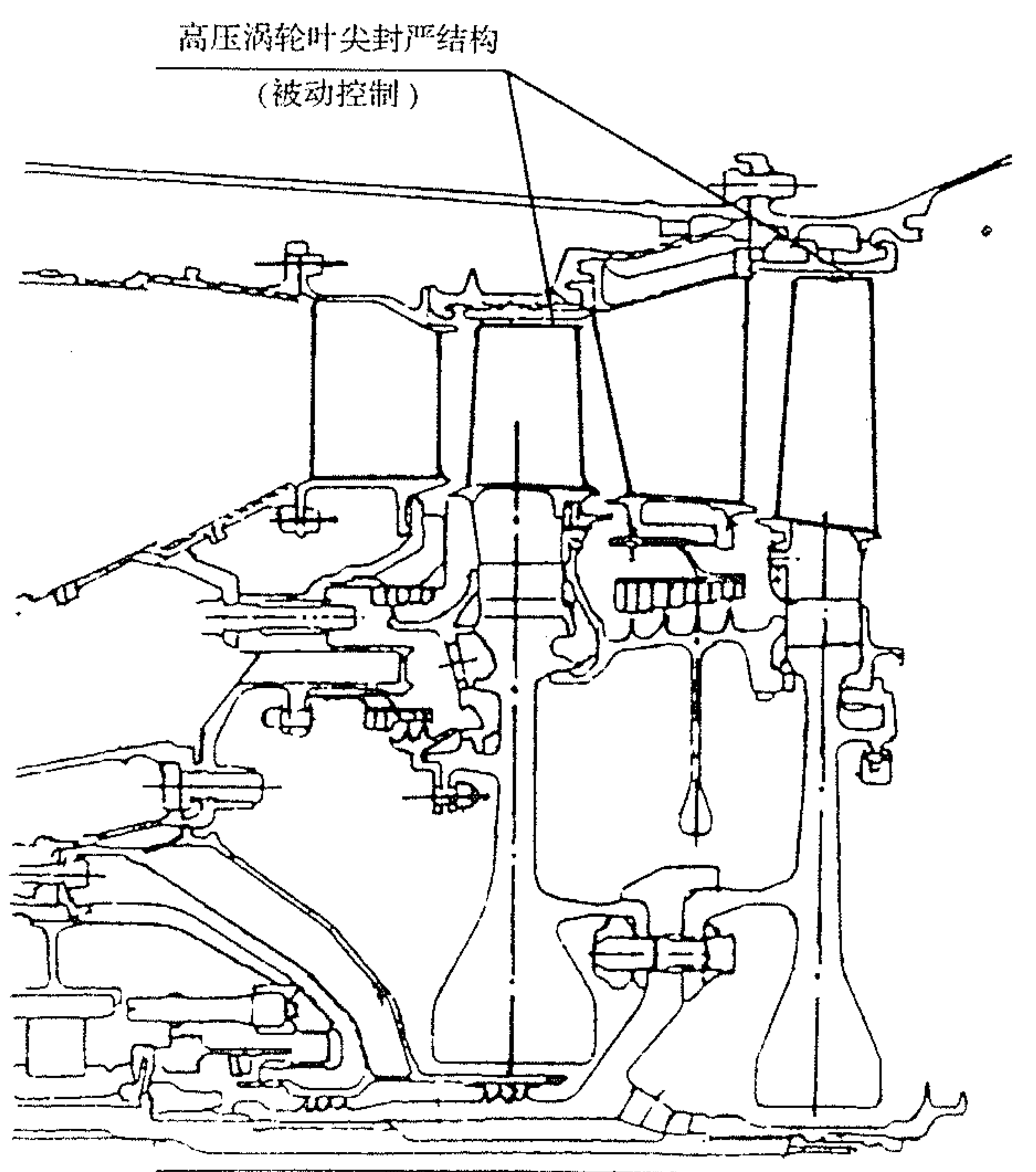
图 12-49 F100 发动机高压涡轮结构
