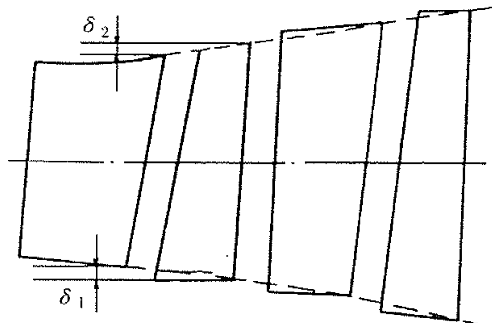
图 3-17 流道中的阶差
