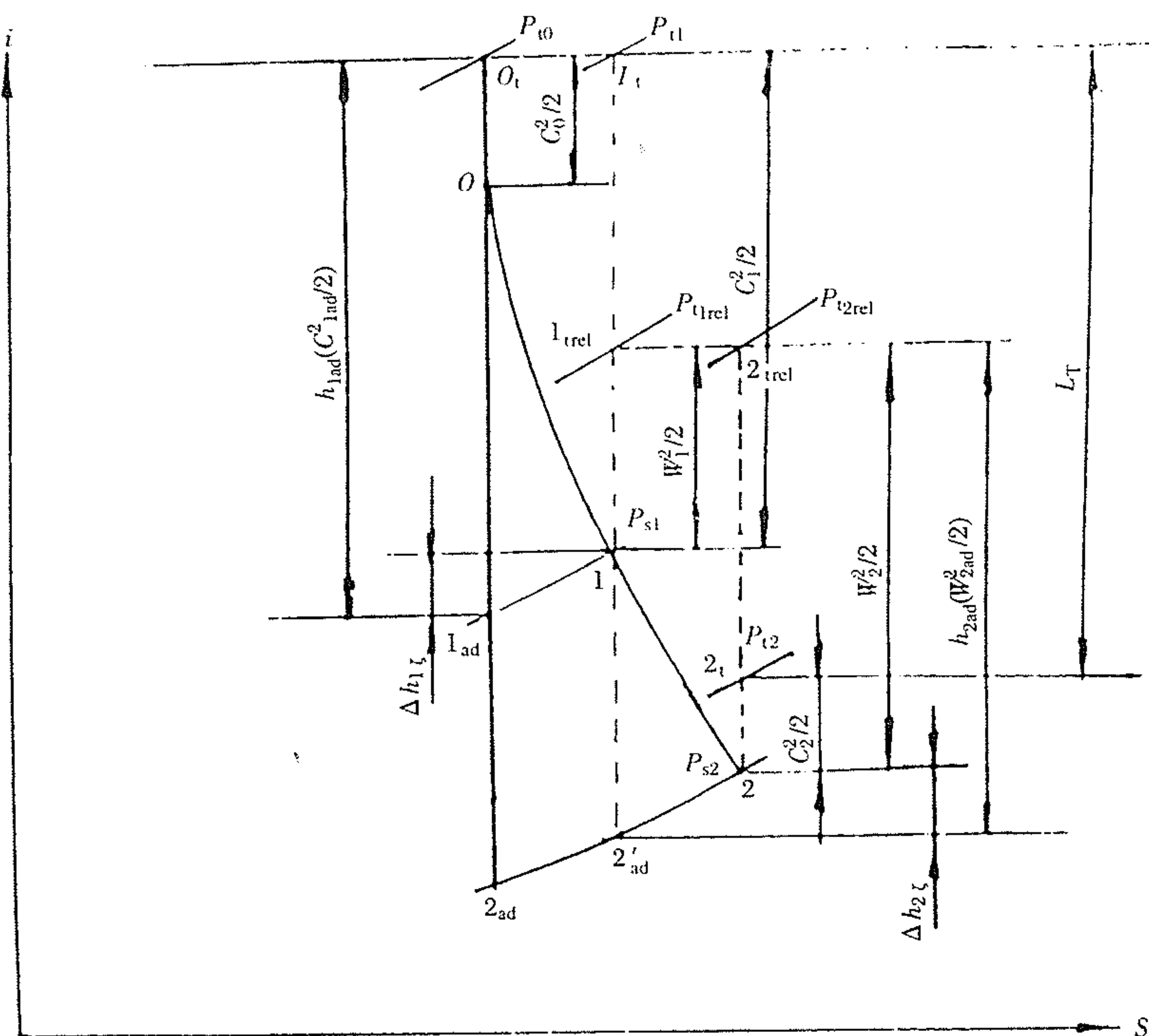
图 3-20 涡轮级焓熵图
