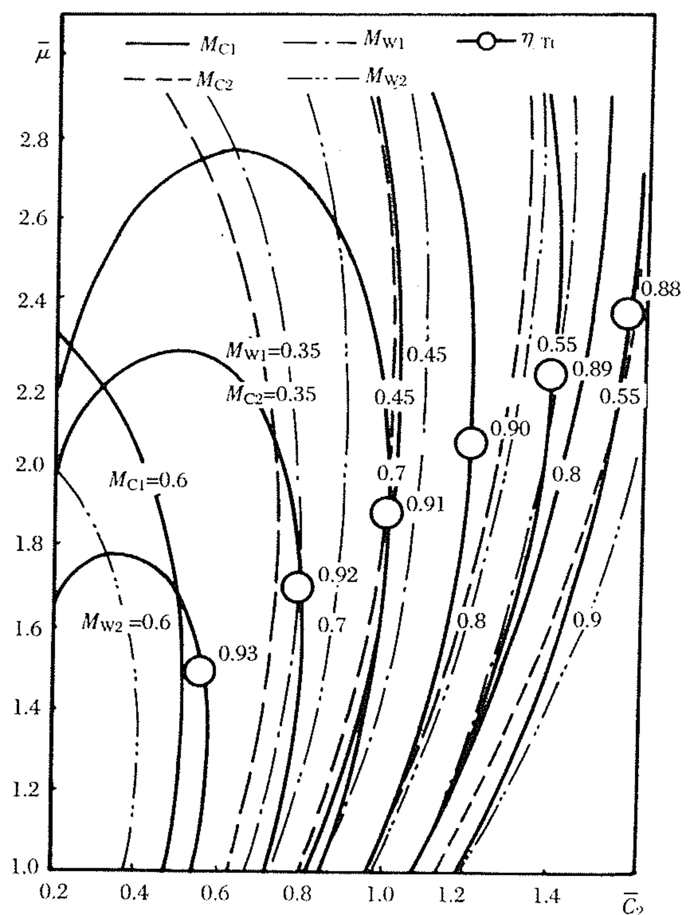
图 2-12 涡轮级参数关系图
