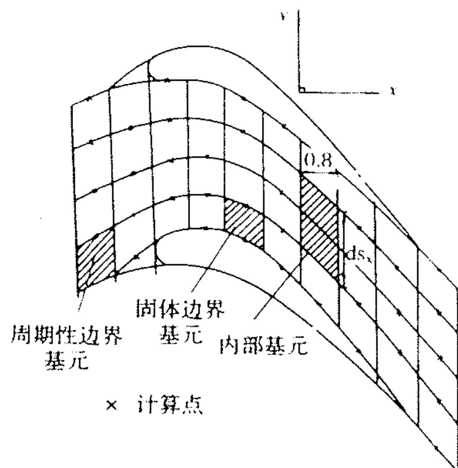
图 5-15 平面叶栅求解流场
