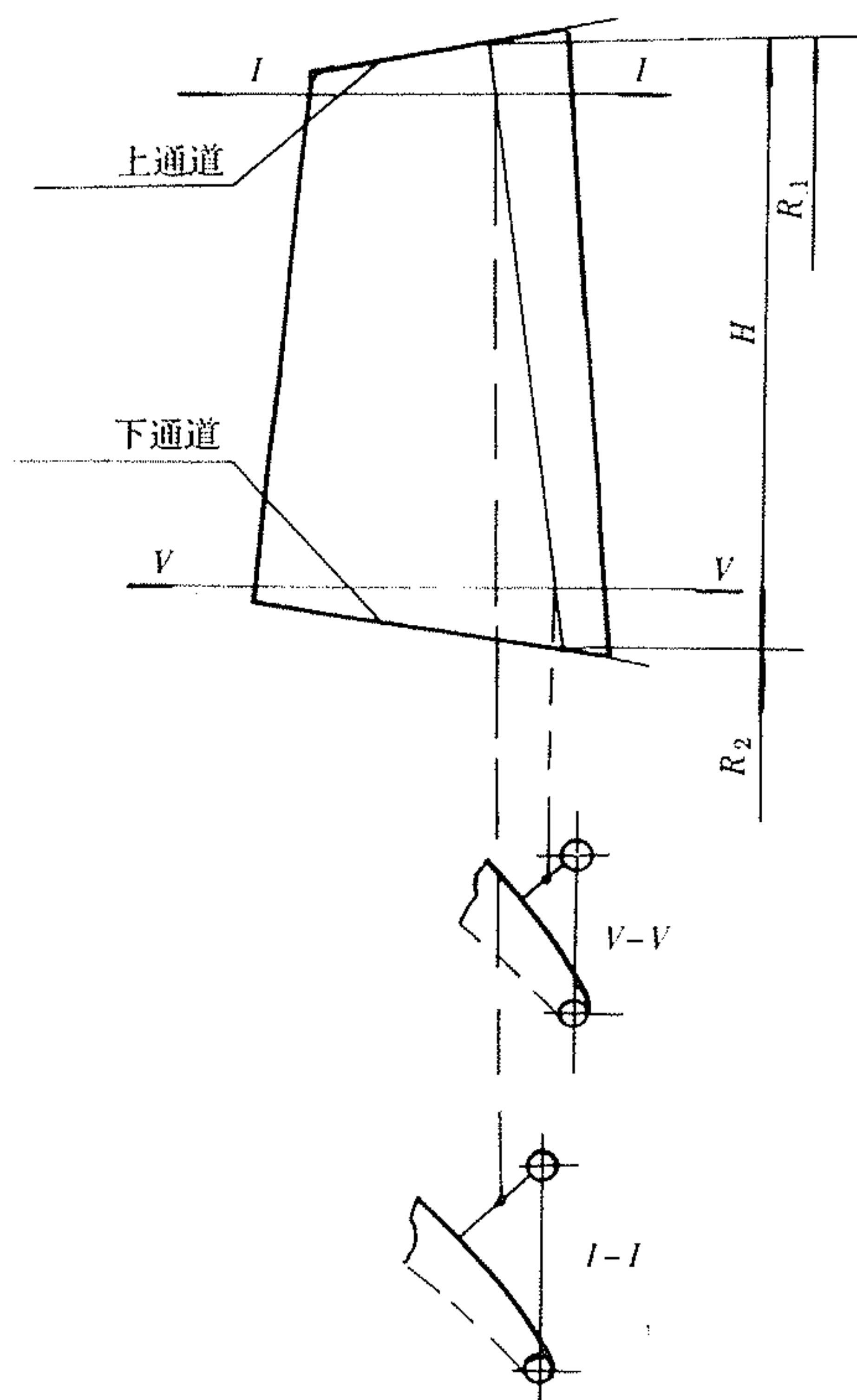
图 4-3 确定排气面积示意图
