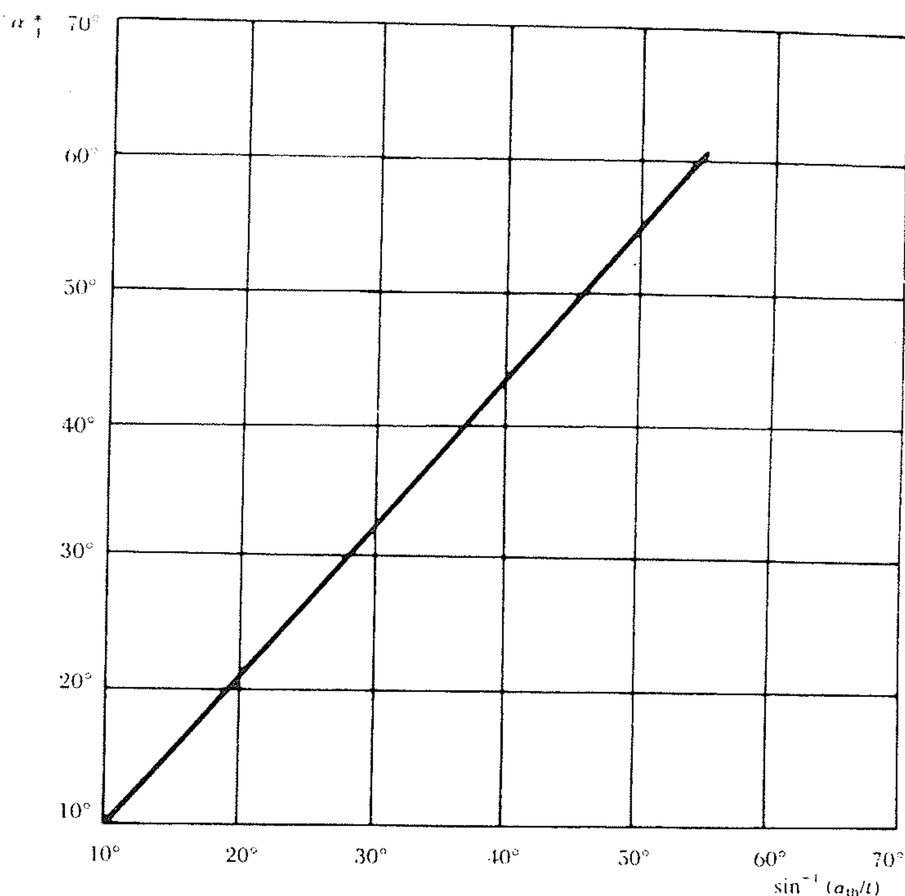
图 3-34 叶片出口气流角与 \sin^{-1}(a_{th}/t) 的关系曲线
