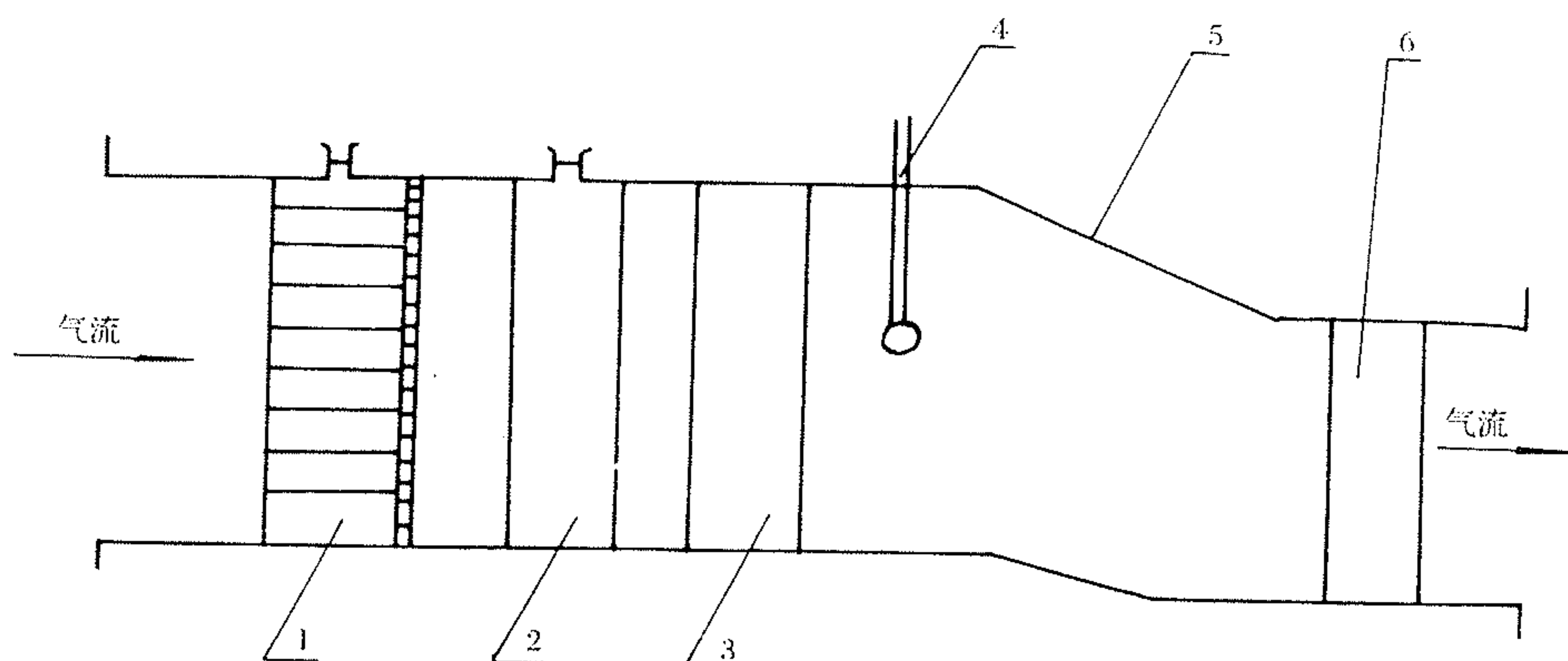
图 13-13 环形叶栅试验流道示意图
