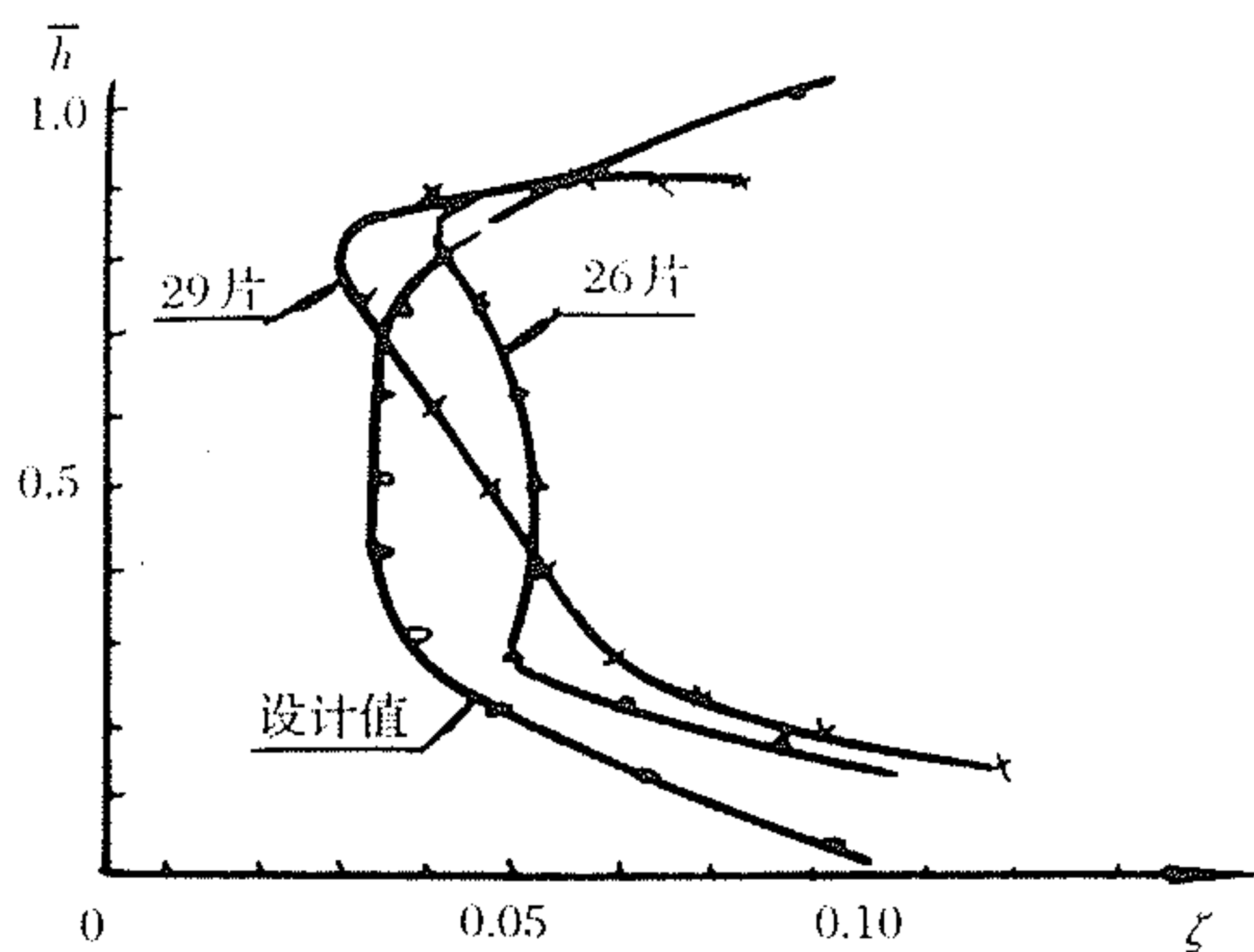
图 13-11 某跨声速涡轮环形叶栅 \bar{\zeta} = f(\bar{h}) 曲线
