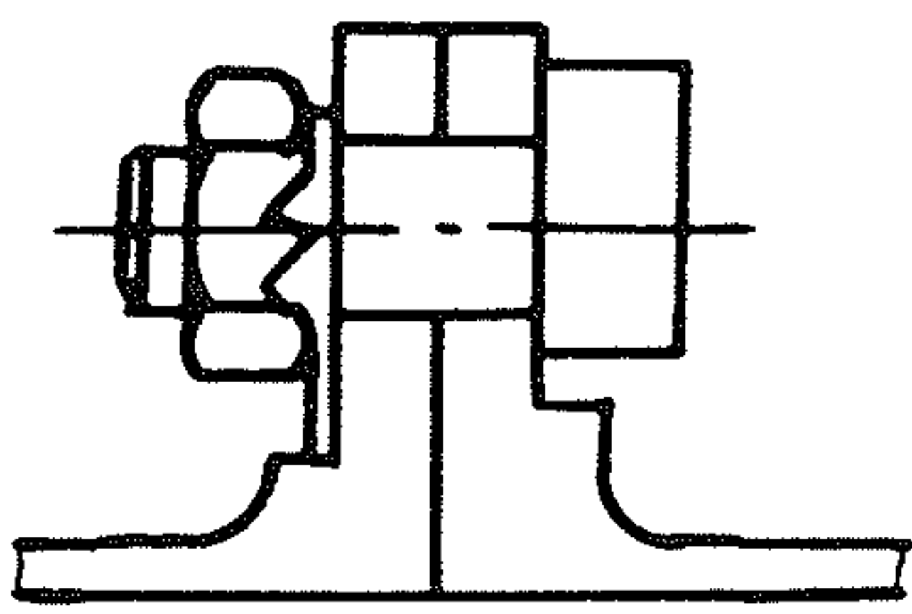
图 11-35 精密螺栓结构示意图
