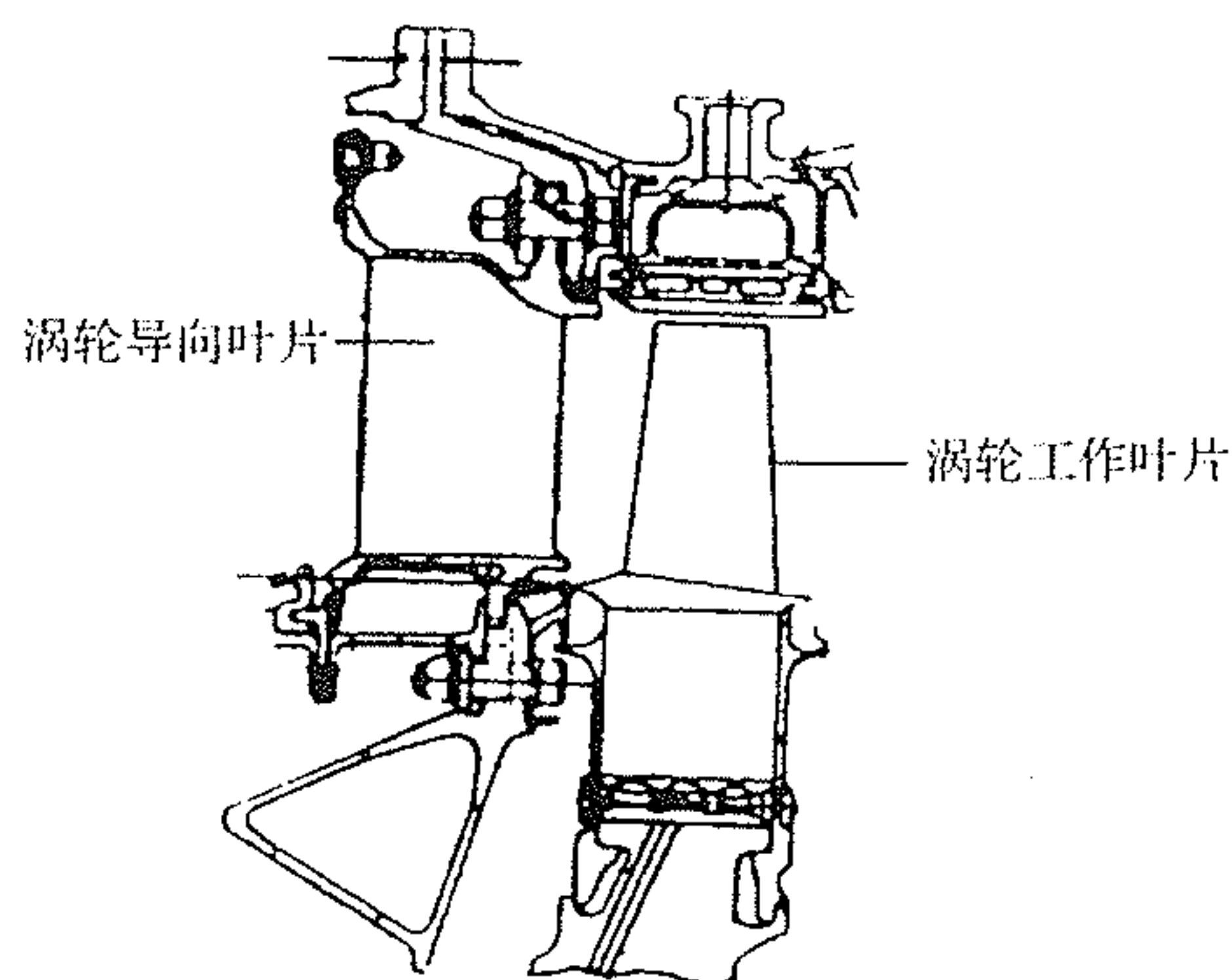
图 12-34 E 3 高压涡轮叶尖主动间隙控制结构示意图
