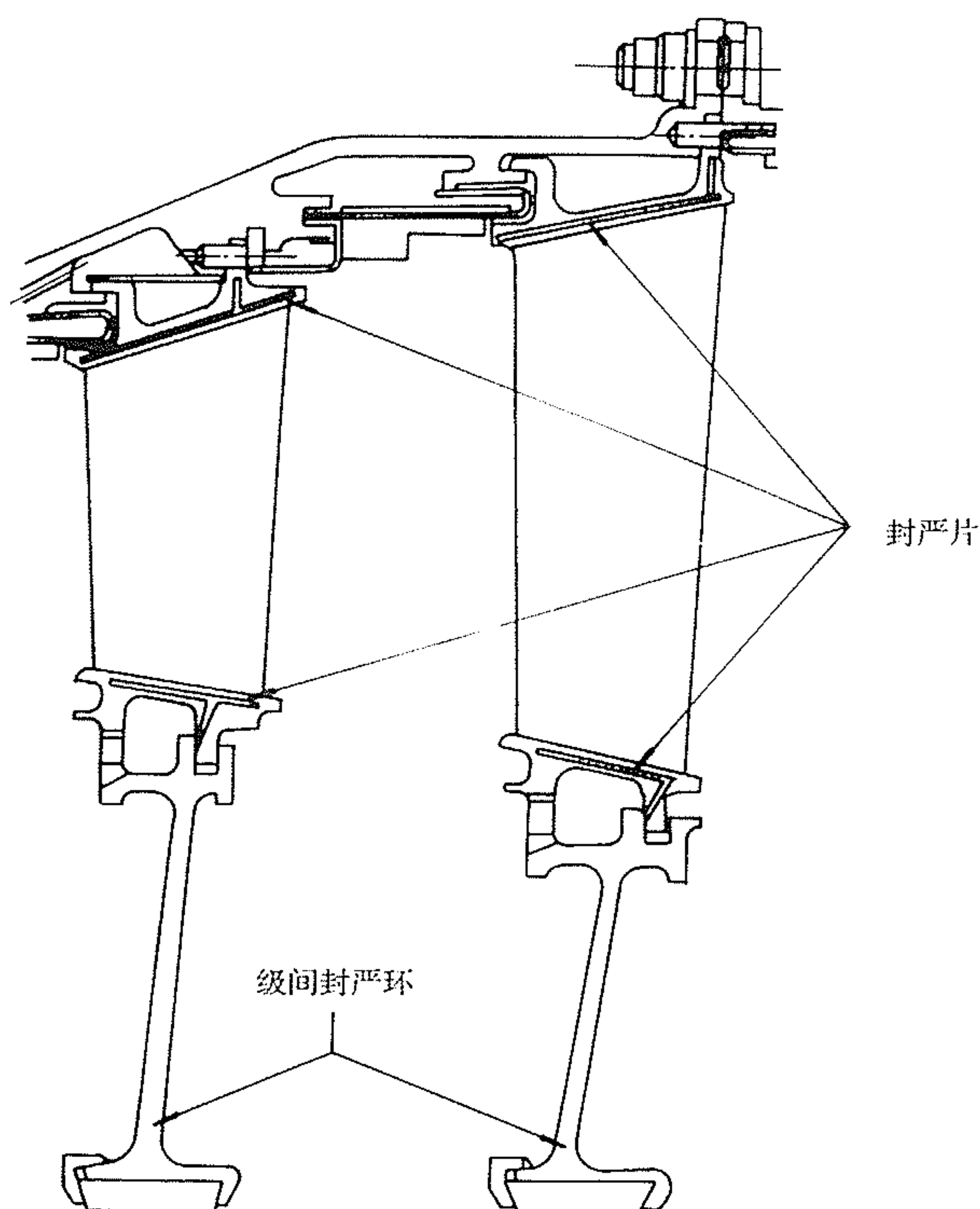
图 12-28 WJ5A1 发动机涡轮导向叶片间封严片示意图
