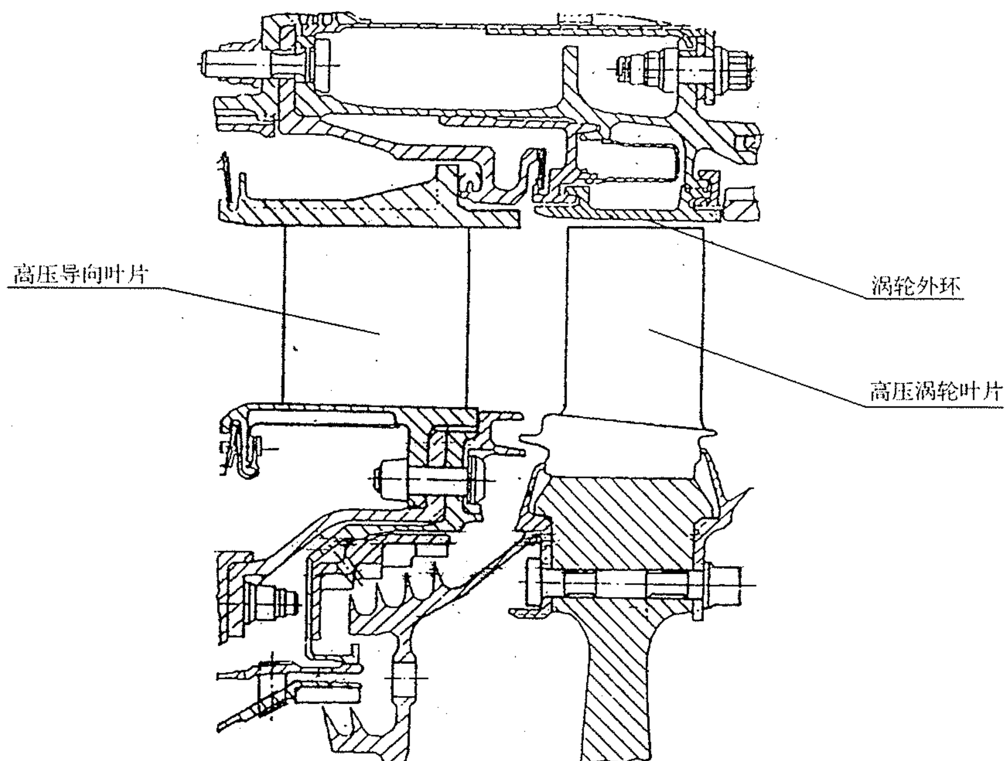
图 12-35 CFM56-3 发动机高压涡轮叶尖主动间隙控制结构示意图
