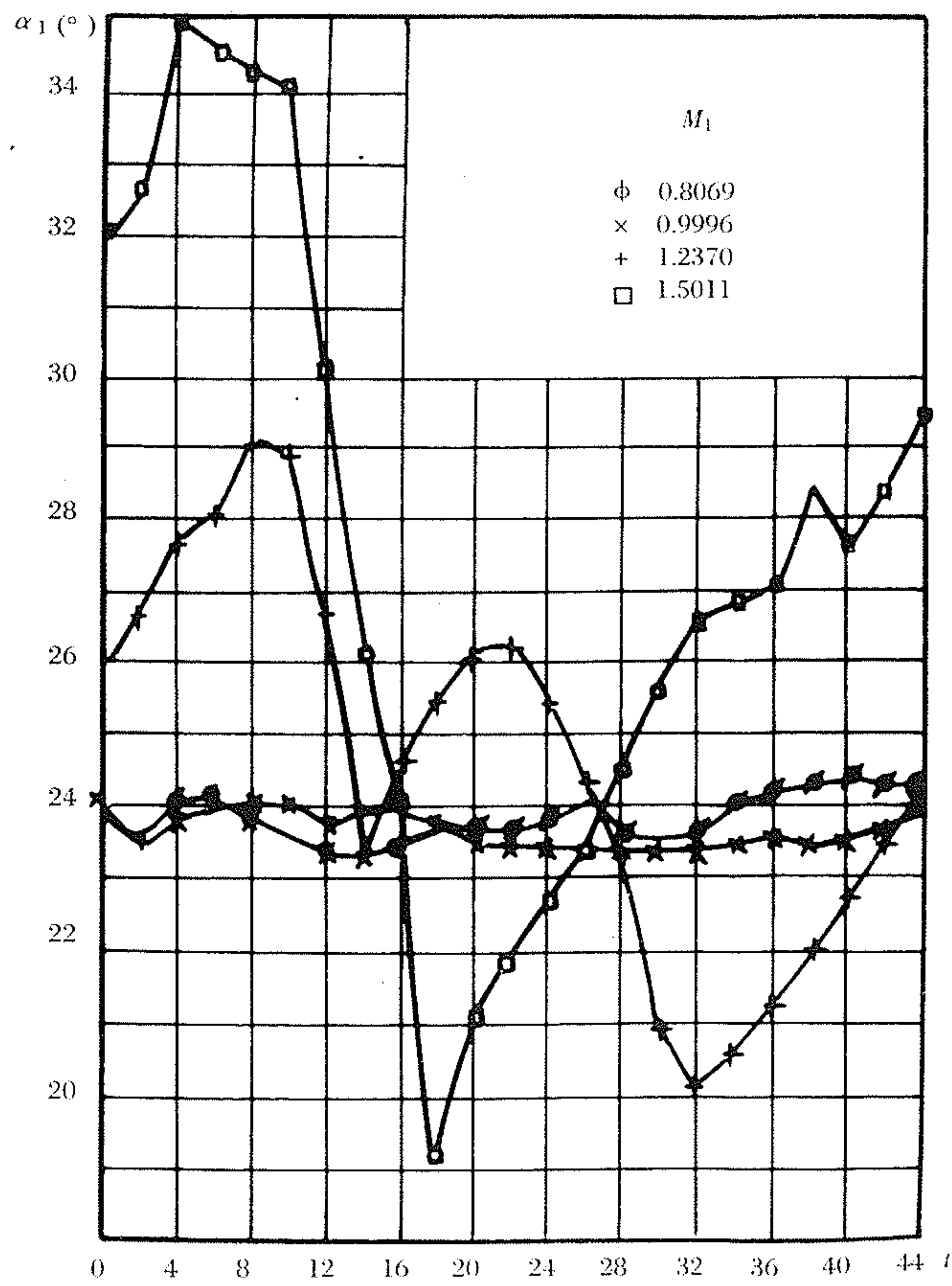
图 13-9 平面叶栅 \alpha_1 = f(t) 曲线
