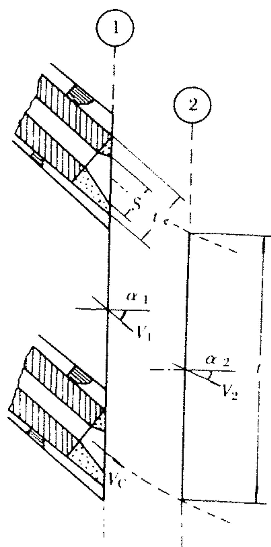
图 5-22 TOTLOS 方法尾缘混合 控制体示意图
