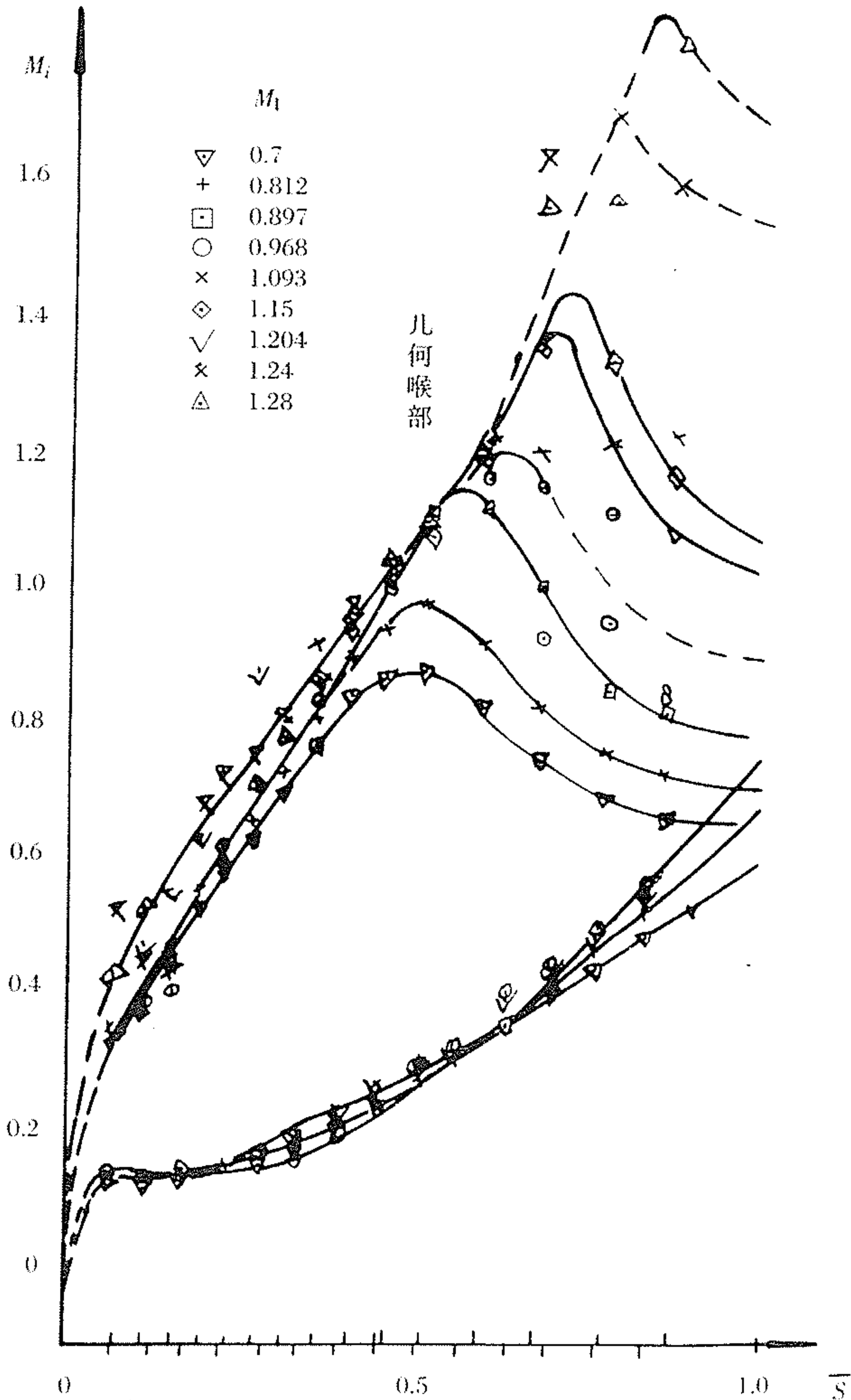
图 13-4 平面叶栅 M_i = f(M_1) 曲线
