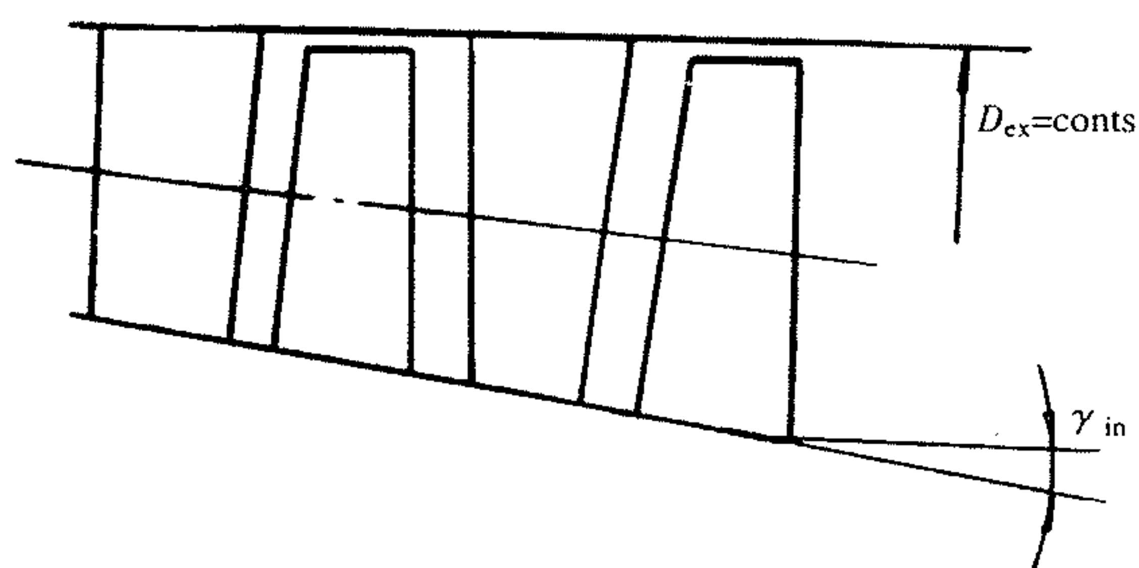
图 3-13 等外径流道
