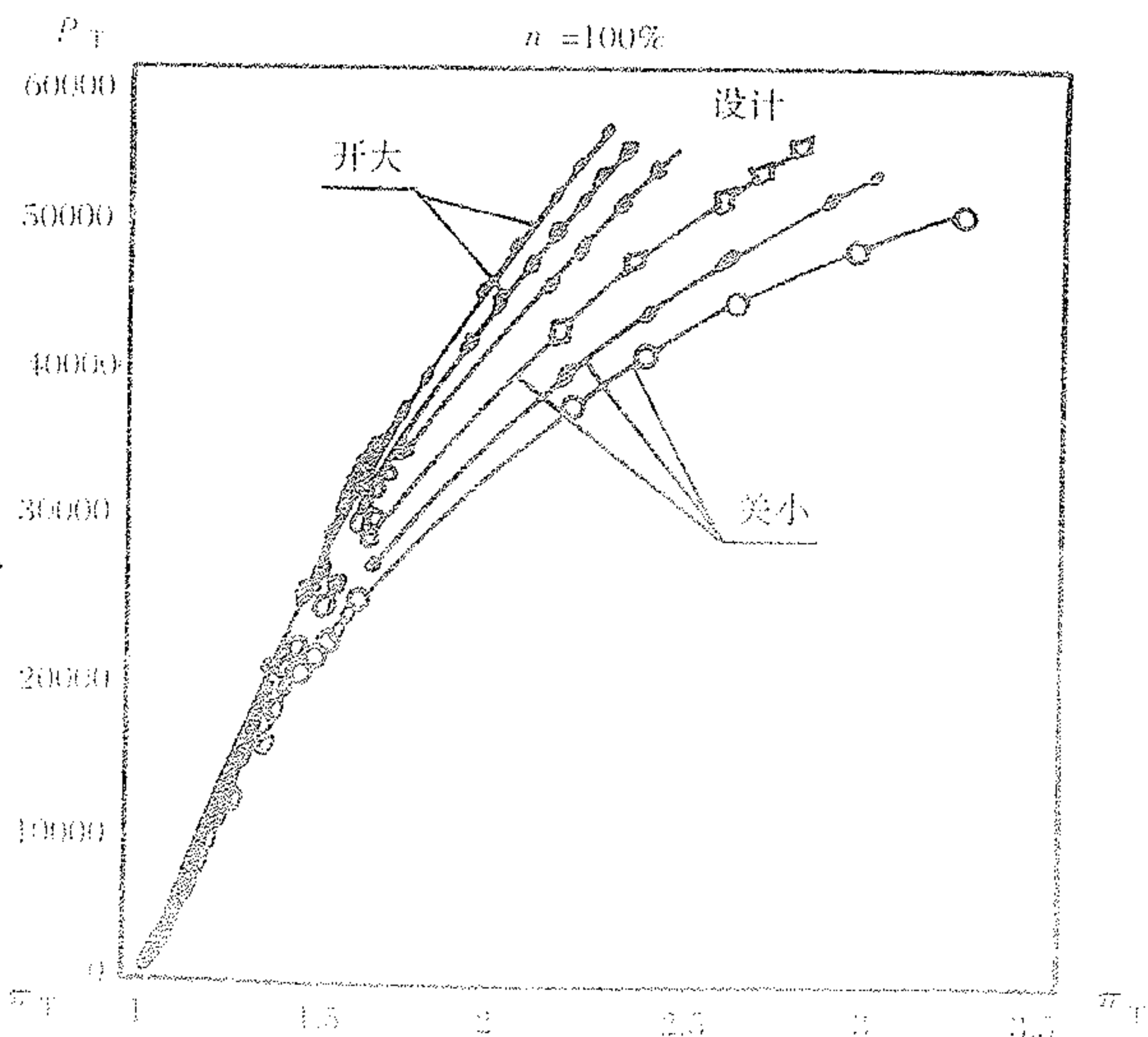
图 13-22 变几何涡轮功率特性
