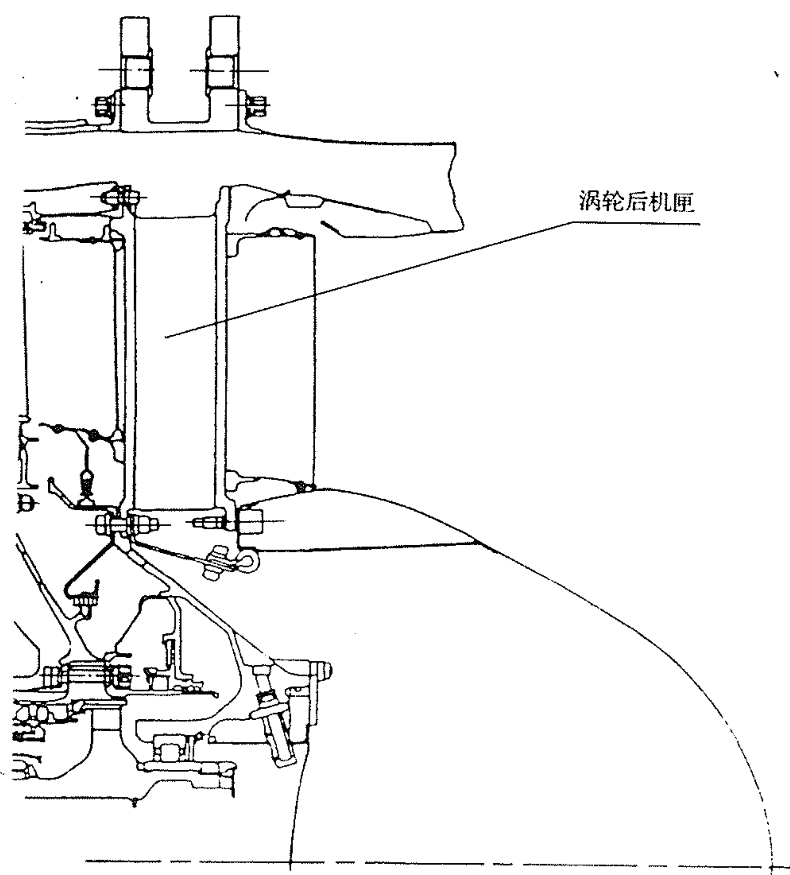
图 11-53 V2500 涡轮后机匣
