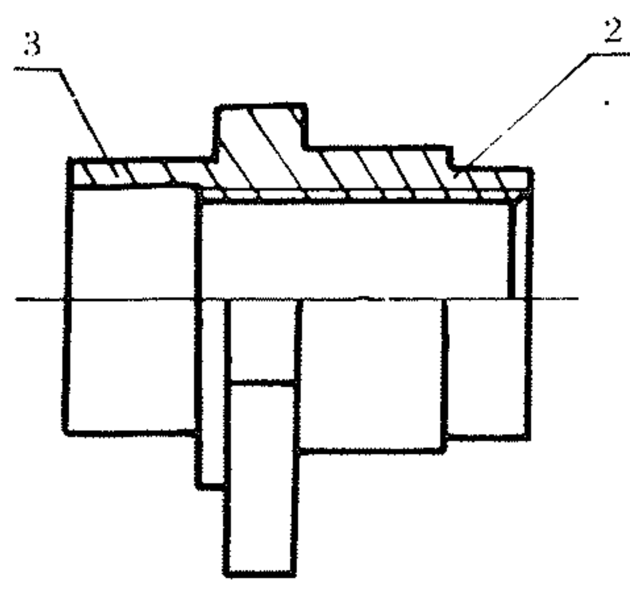
图 10-10 托板自锁铆轴螺母 1—托板;2—螺母;3—铆轴
