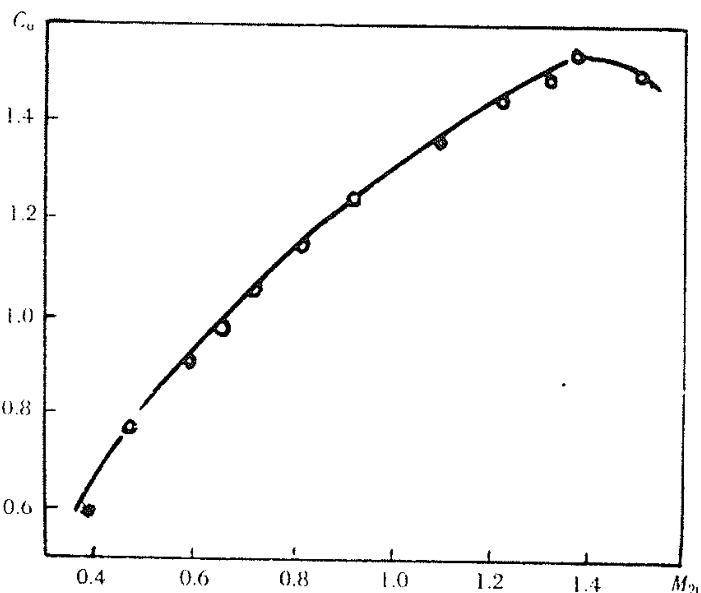
图 5-11 负荷系数随出口状态变化曲线
