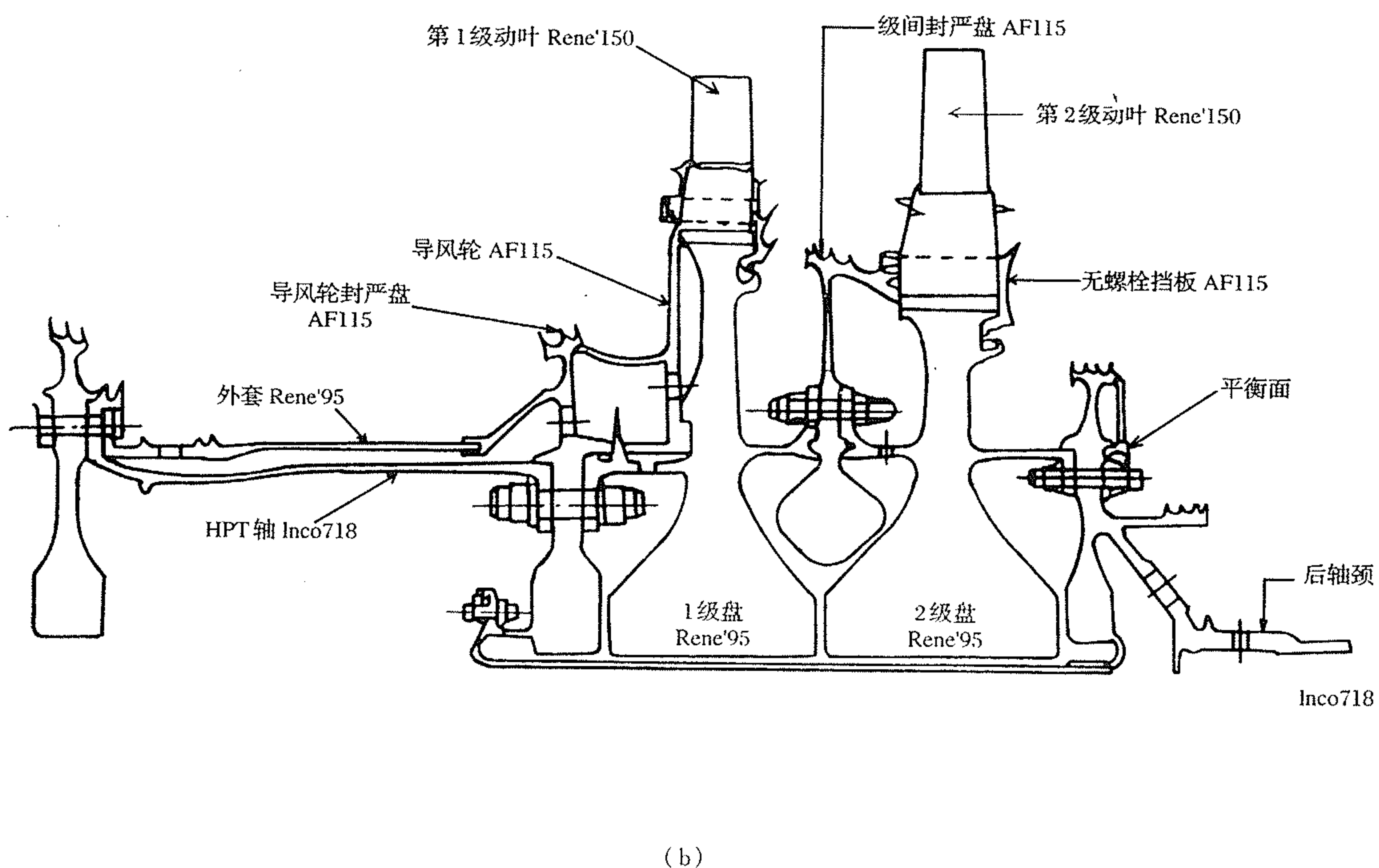
图 8-24 涡轮结构选材示例图
