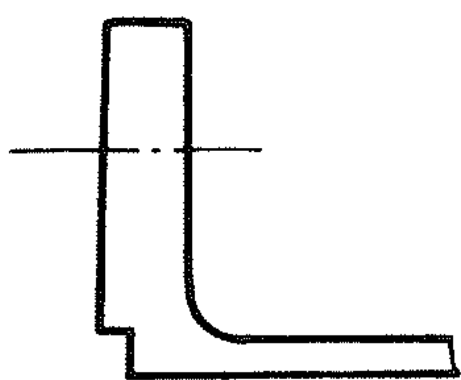
图 11-27 机匣安装边转接处为“危险”截面
