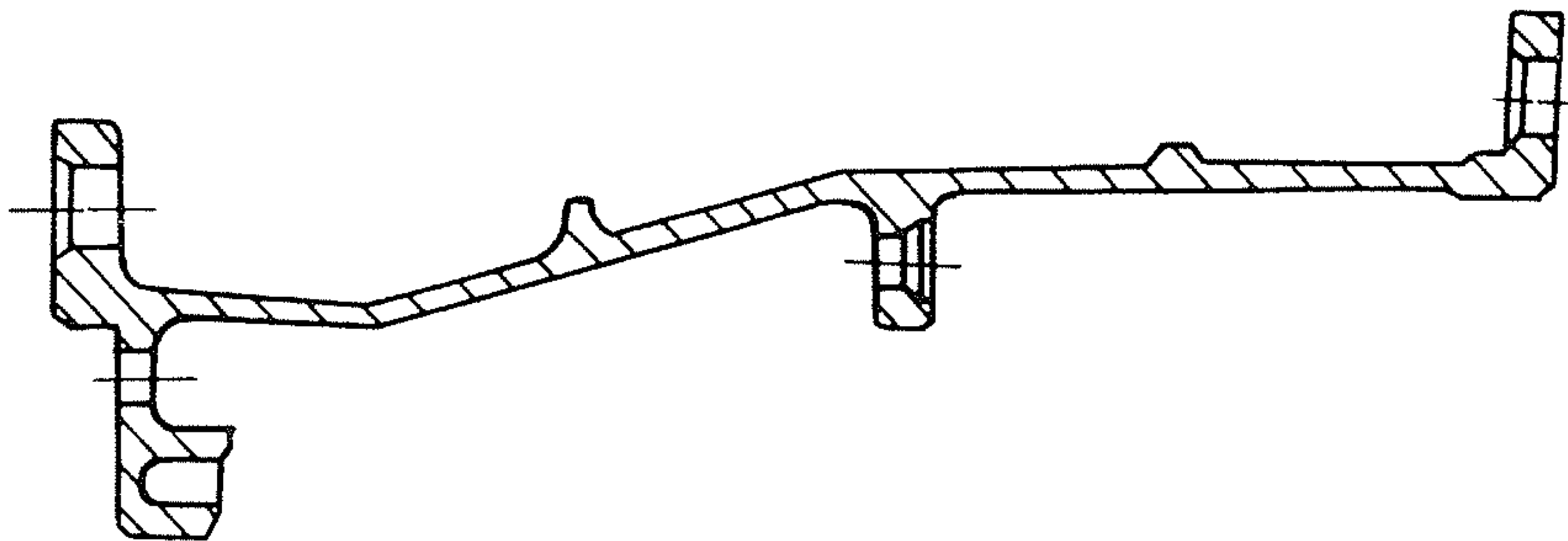
图 11-33 某型发动机低压涡轮机匣示意图
