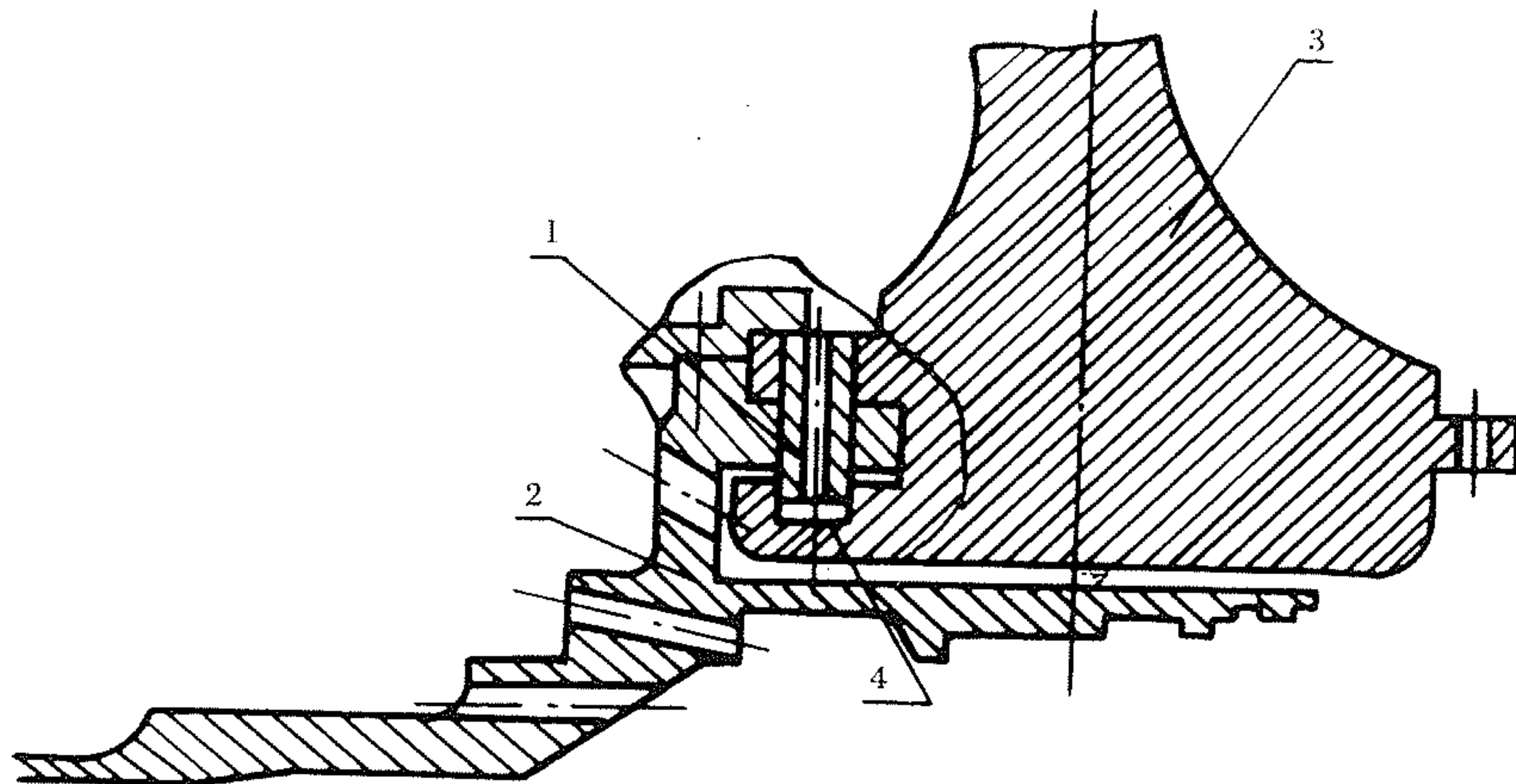
图 10-16 叉形安装边销子连接的涡轮盘轴
