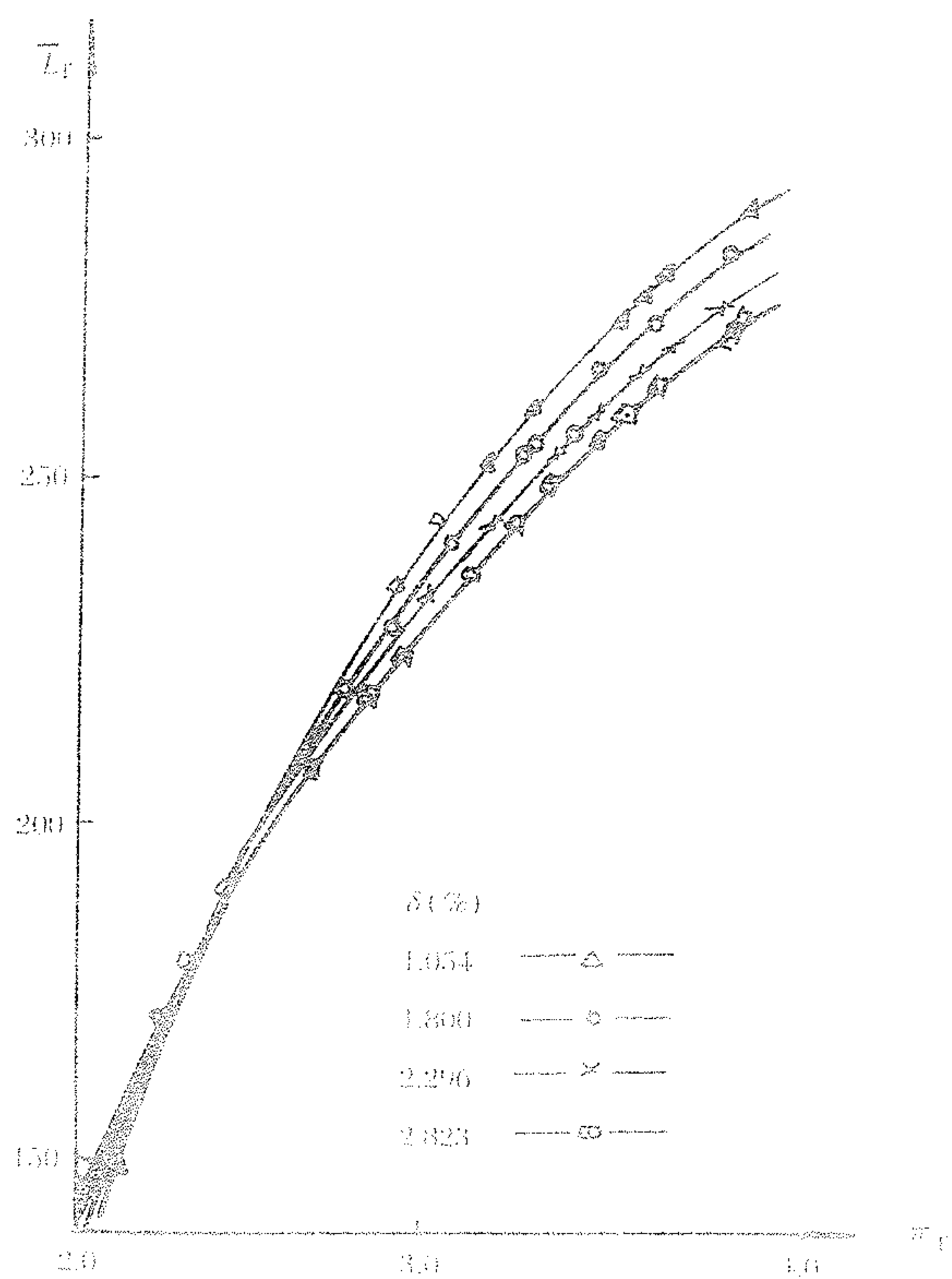
图 13-19 功量随 \delta 的变化曲线
