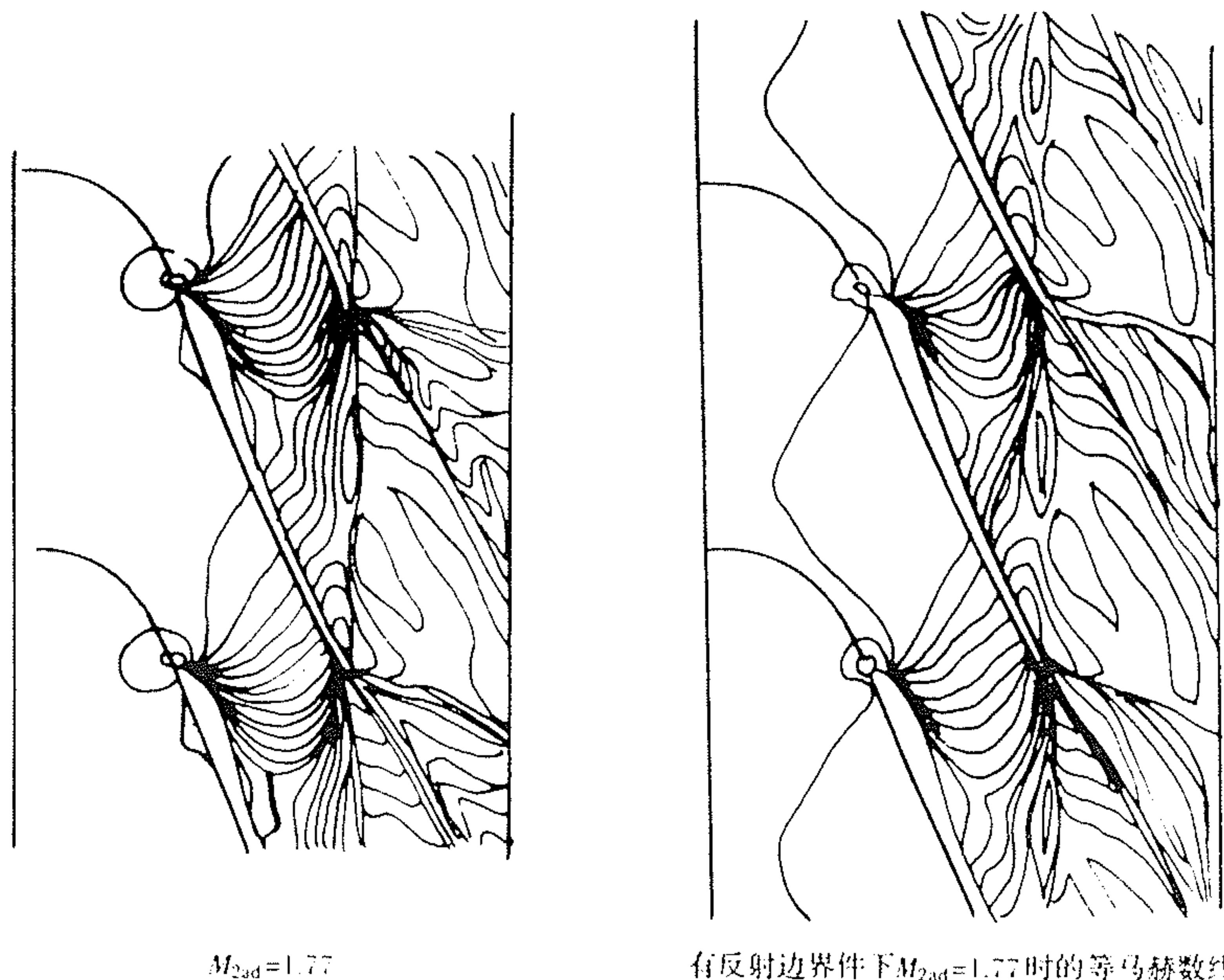
图 5-17 有、无反射边界条件等马赫线的对比
