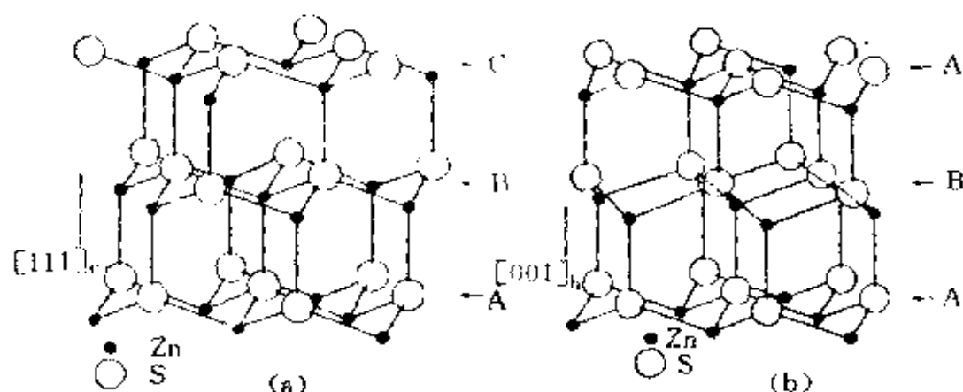
图 9.4 ZnS 的结构
