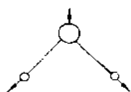
对称伸缩
