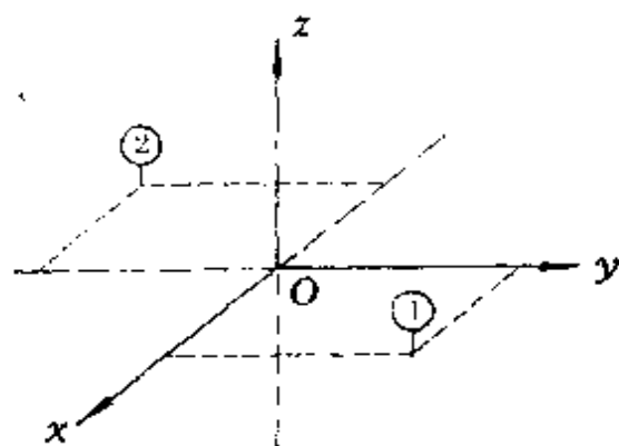
图 4.1 C_2 的对称操作
