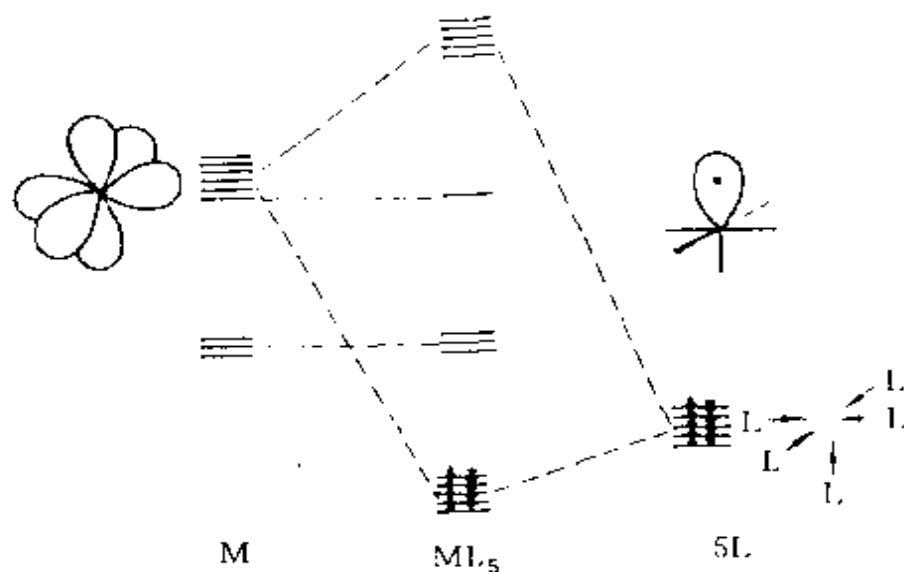
图 6.18 ML_5 分子轨道能级图
