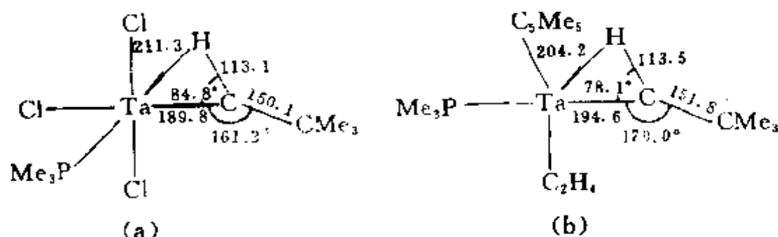
图 10.11 和 C—H→M 键有关的一些结构参数
