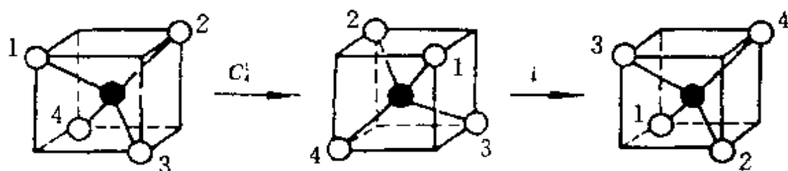
图 4.4 具有 I_4 轴分子经过 I_4 操作的情况
