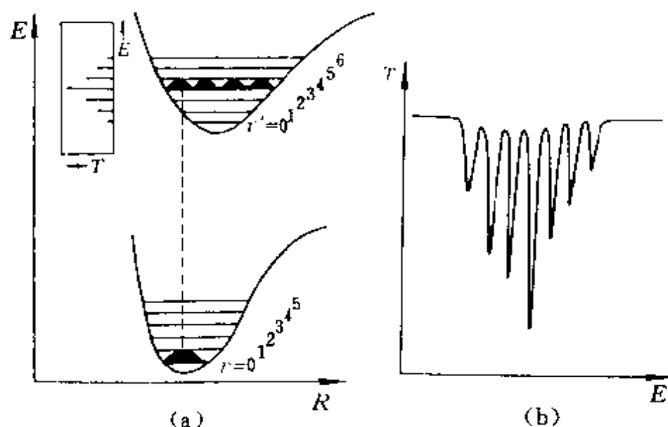
图 3.24 \text{H}_2 分子由 \sigma^2_{1s} \rightarrow \sigma^1_{1s} \cdot \pi^2_{3p} (a) 跃迁的能级示意图 (b) 光谱示意图
