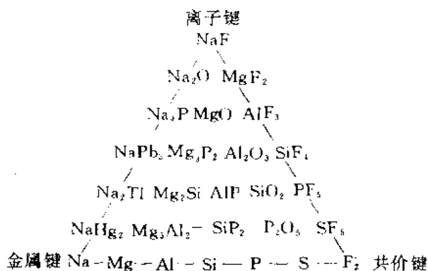
图 9.9 若干化合物的键型
