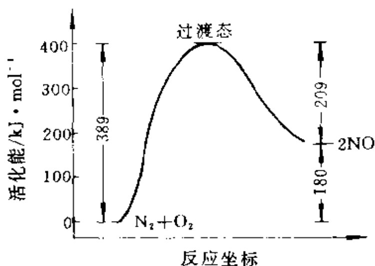
图 5.13 \text{N}_2 + \text{O}_2 \longrightarrow 2\text{NO} 的反应过程
