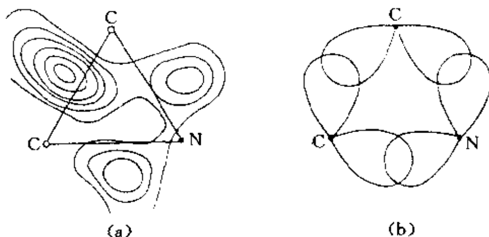
图 5.3 -\text{NC}_2\text{H}_4 三元环中的弯键
