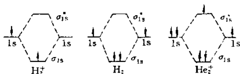
图 3.9 H_2^+ , H_2 和 He_2^+ 的电子排布图
