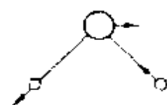
不对称伸缩
