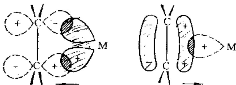
图 6.15 过渡金属(M)和烯烃 \begin{pmatrix} \diagup & \diagdown \\ \text{C} & = & \text{C} \\ \diagdown & \diagup \end{pmatrix} 间形成 \sigma - \pi 配键的情况
