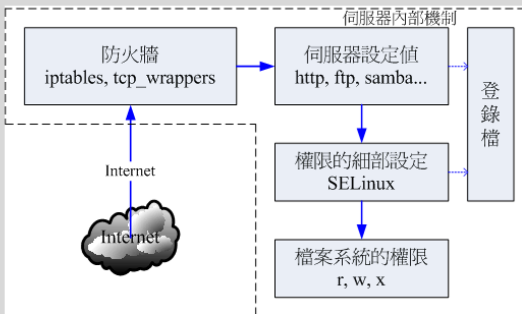
图 7.1-1、网络封包进入主机的流程
