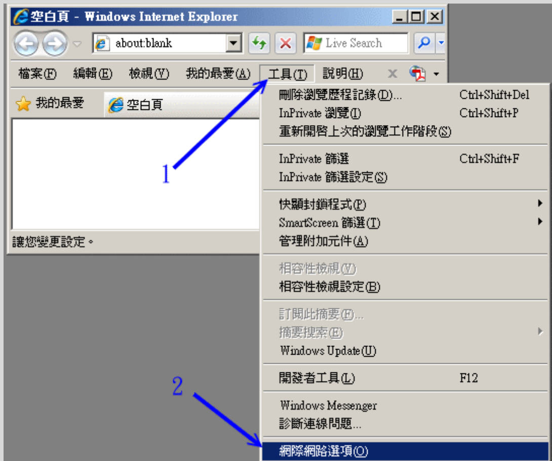
图 17.3-4、在 IE 上设定 proxy 的流程
