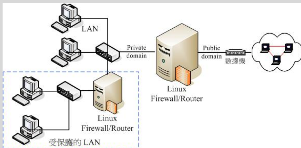
图 9.1-3、内部网络包含需要更安全的子网防火墙
