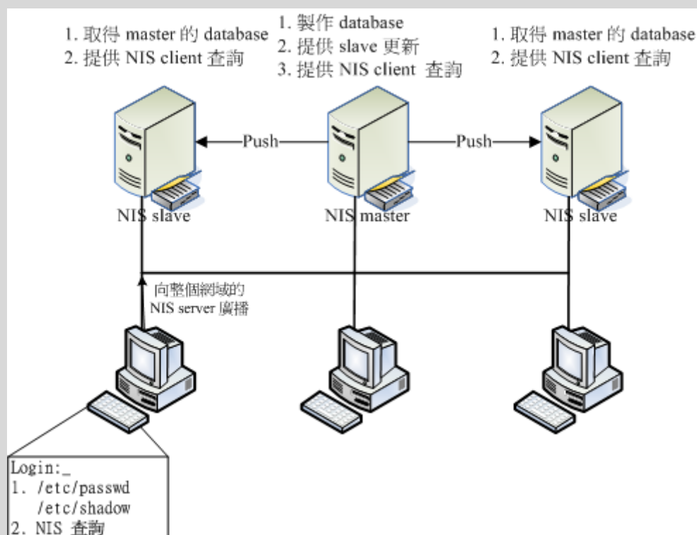
图 14.1-1、NIS 服务器与客户端的运作与查询方式示意图
