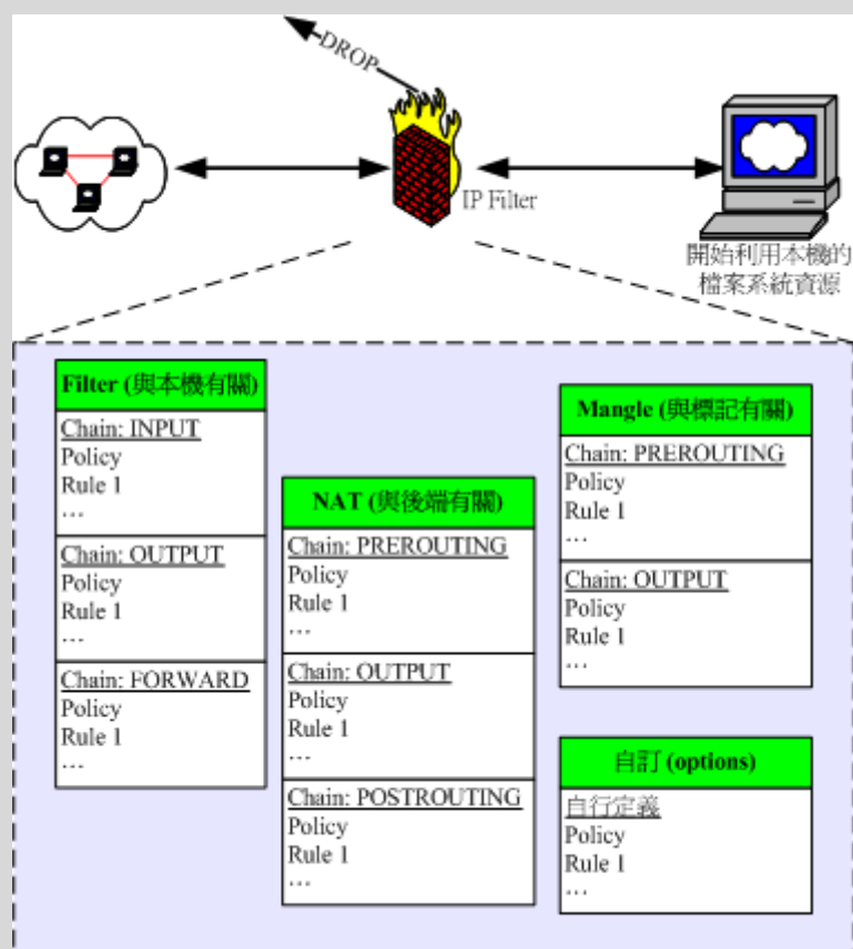
图 9.3-2、iptables 的表格与相关链示意图
