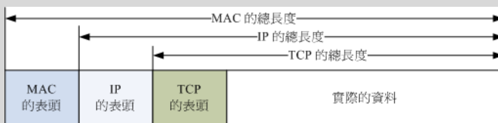
图 2.4-1、各封包之间的相关性
