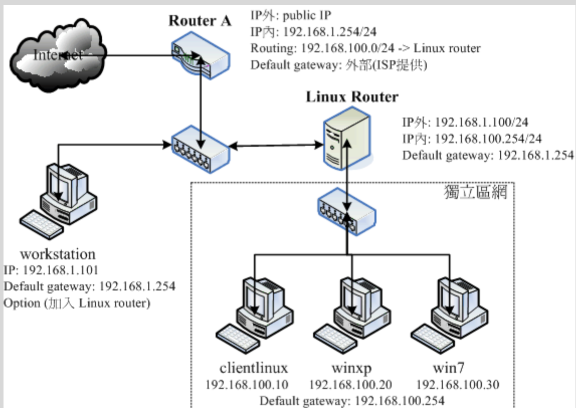
图 8.2-1、静态路由之路由器架构示意图
