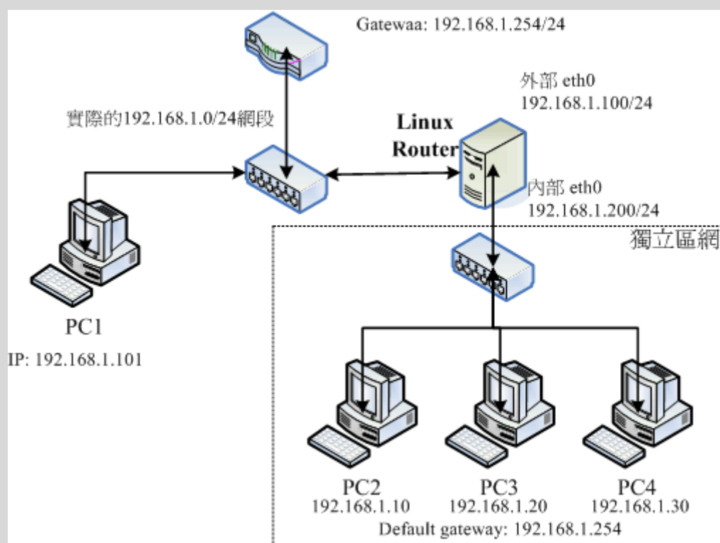
图 8.4-1、在路由器两个界面两边的 IP 是在同一个网段的设定情况
