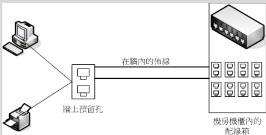
图 2.2-6、结构化布线简易图标
