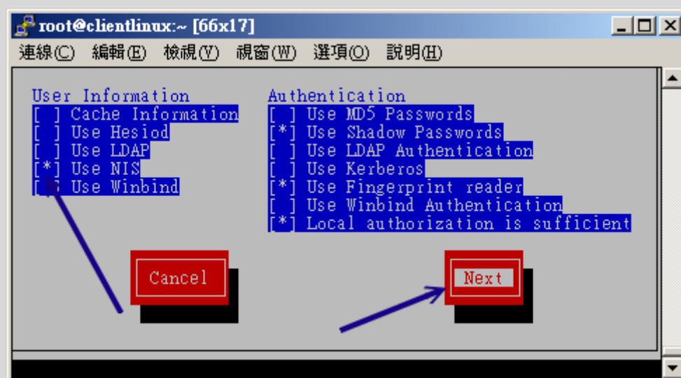
图 14.3-2、进入 authconfig 之后，选择 NIS 项目
