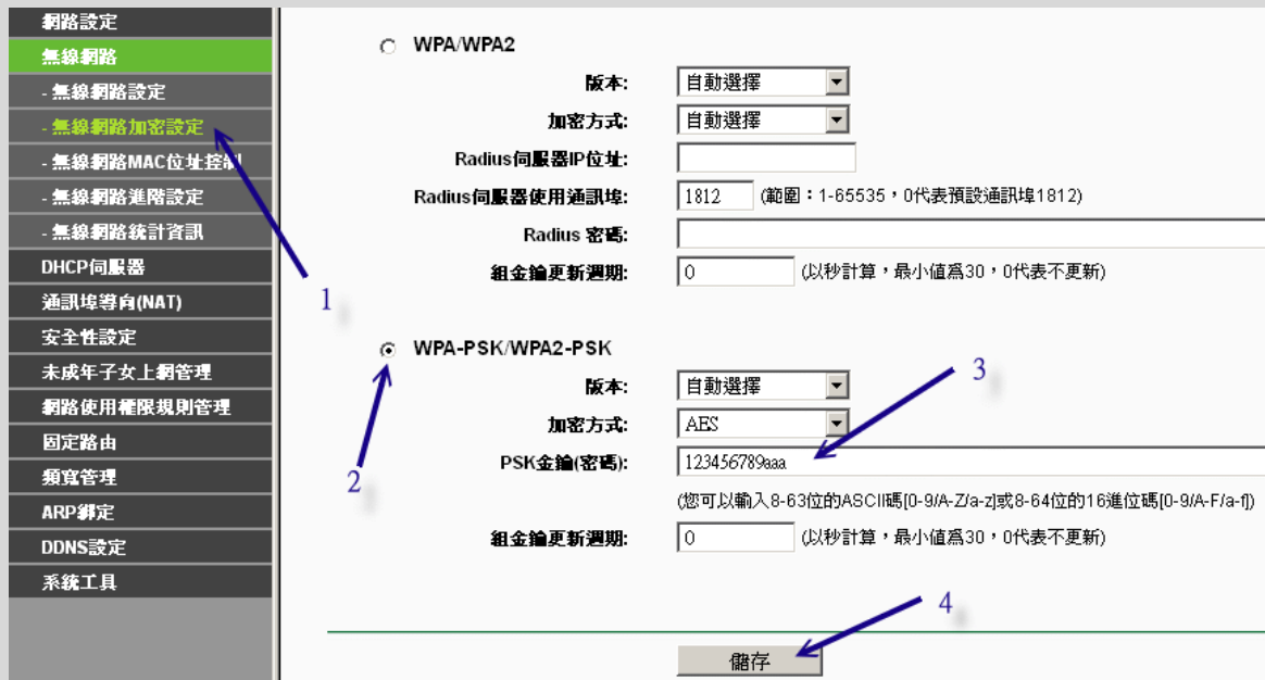
图 4.3-3、无线网络 AP 的密钥设定项目
