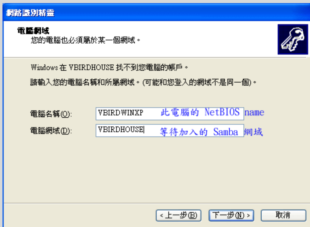
图 16.4-4、Windows 客户端连上 PDC 的方式流程示意图
