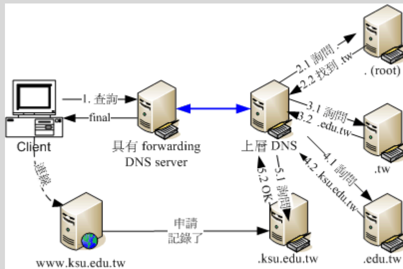
图 19.3-1、具有 forwarding 功能的 DNS 服务器查询方式
