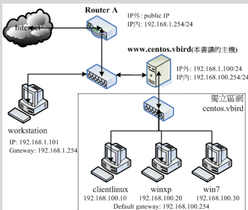
图 3.2-1、本书所使用的区网环境与参数设定
