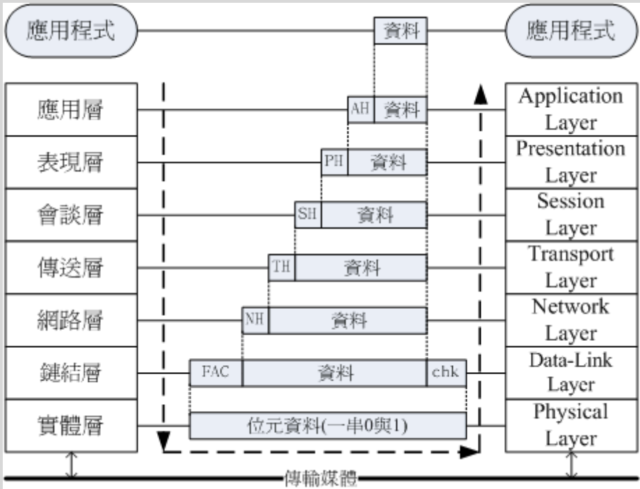
图 2.1-3、OSI 七层协议数据的传递方式
