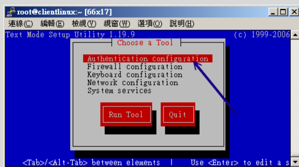
图 14.3-1、利用 setup 进入 authconfig 认证项目
