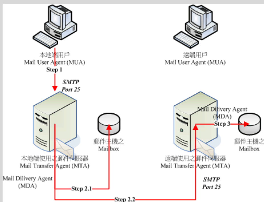
图 22.1-1、电子邮件的『传送』过程示意图
