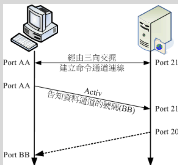
图 21.1-1、FTP 服务器的主动式联机示意图
