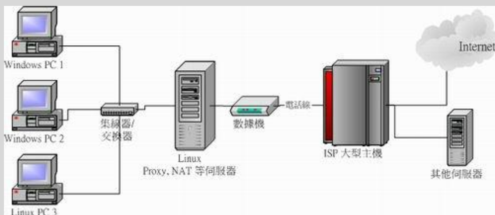
图 6.1-1、局域网的联机状态示意图
