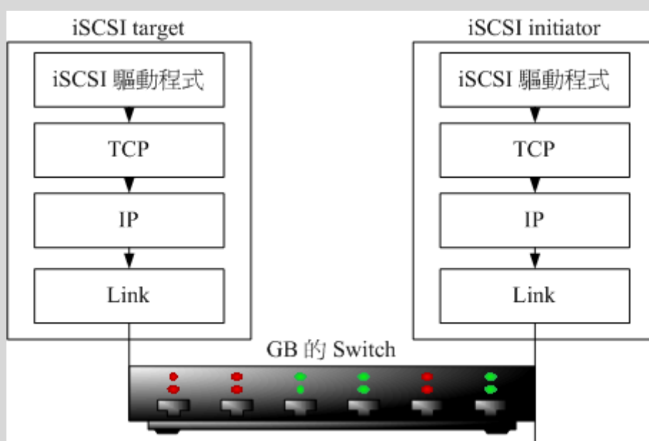
图 18.1-1、iSCSI 与 TCP/IP 相关性
