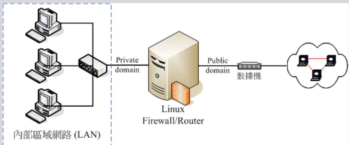
图 9.1-2、单一网域，仅有一个路由器的环境示意图
