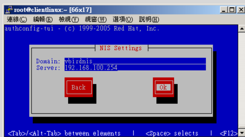
图 14.3-3、填写 NIS 领域以及 NIS 服务器的 IP 即可
