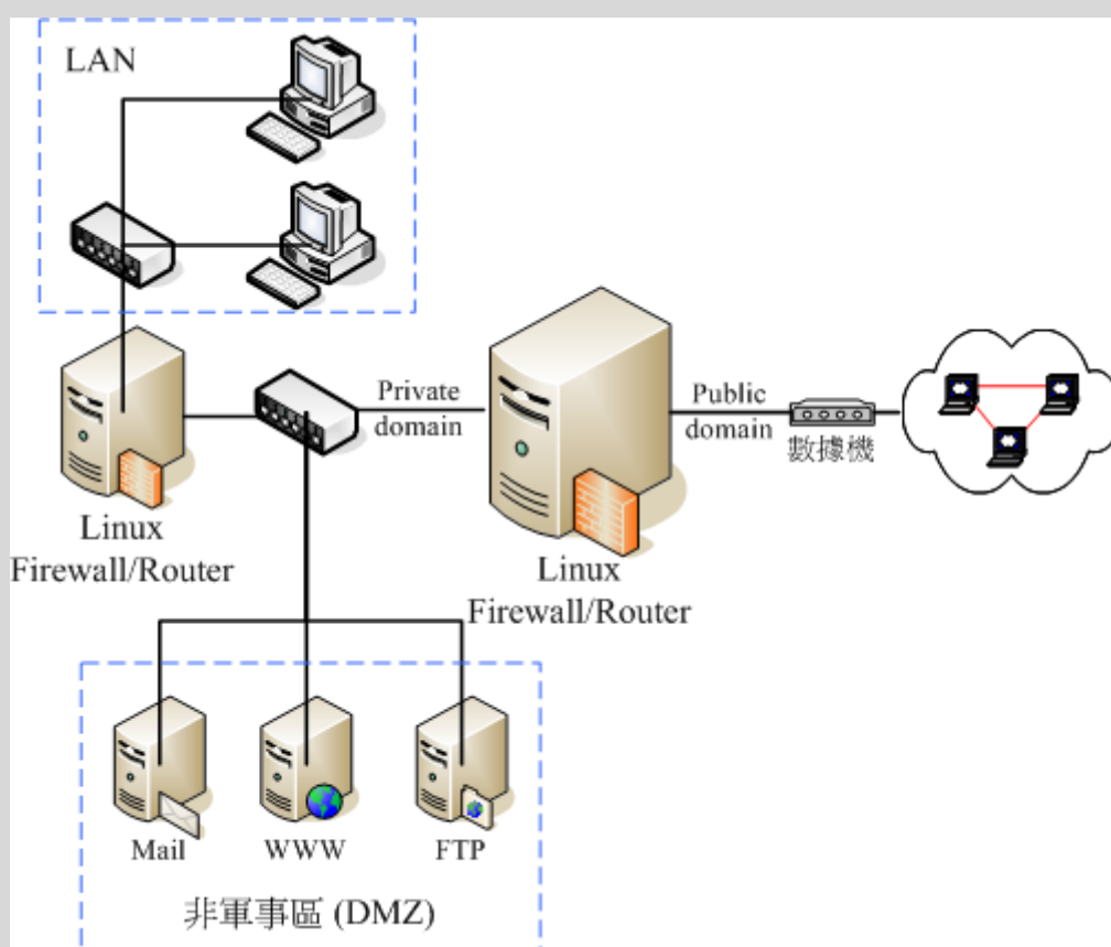
图 9.1-4、架设在防火墙后端的网络服务器环境示意图
