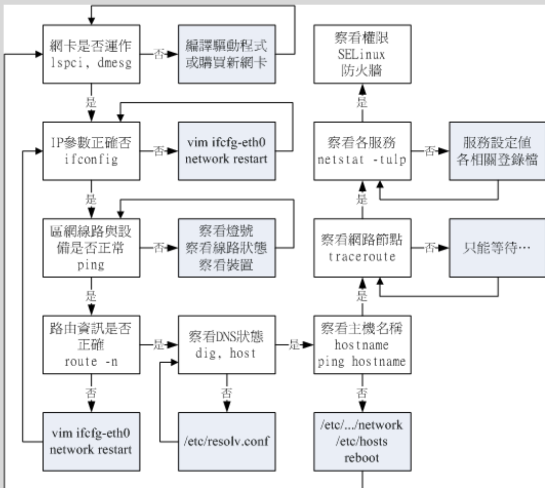
图 6.2-1、网络问题解决流程图
