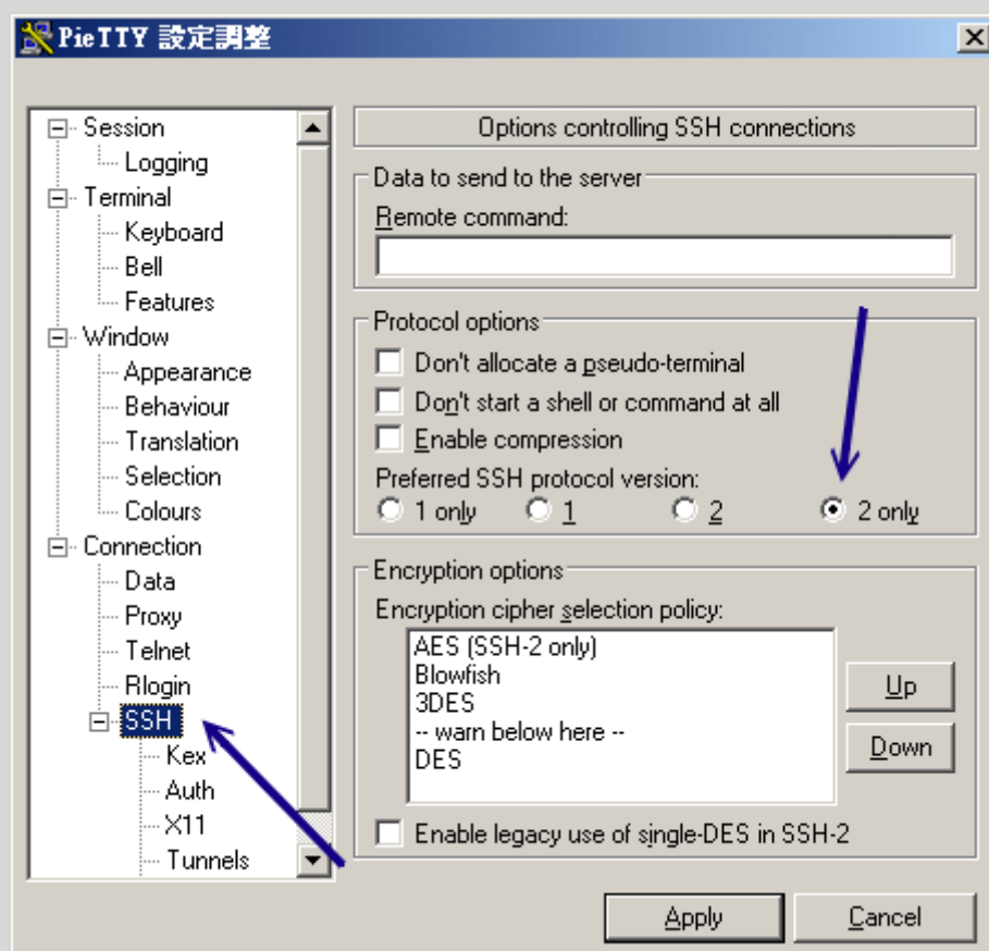
图 11.2-8、设定登入服务器时使用的 ssh 算法版本
