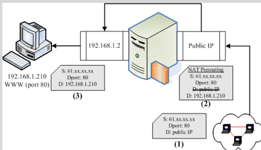
图 9.5-3、DNAT 的封包传送示意图
