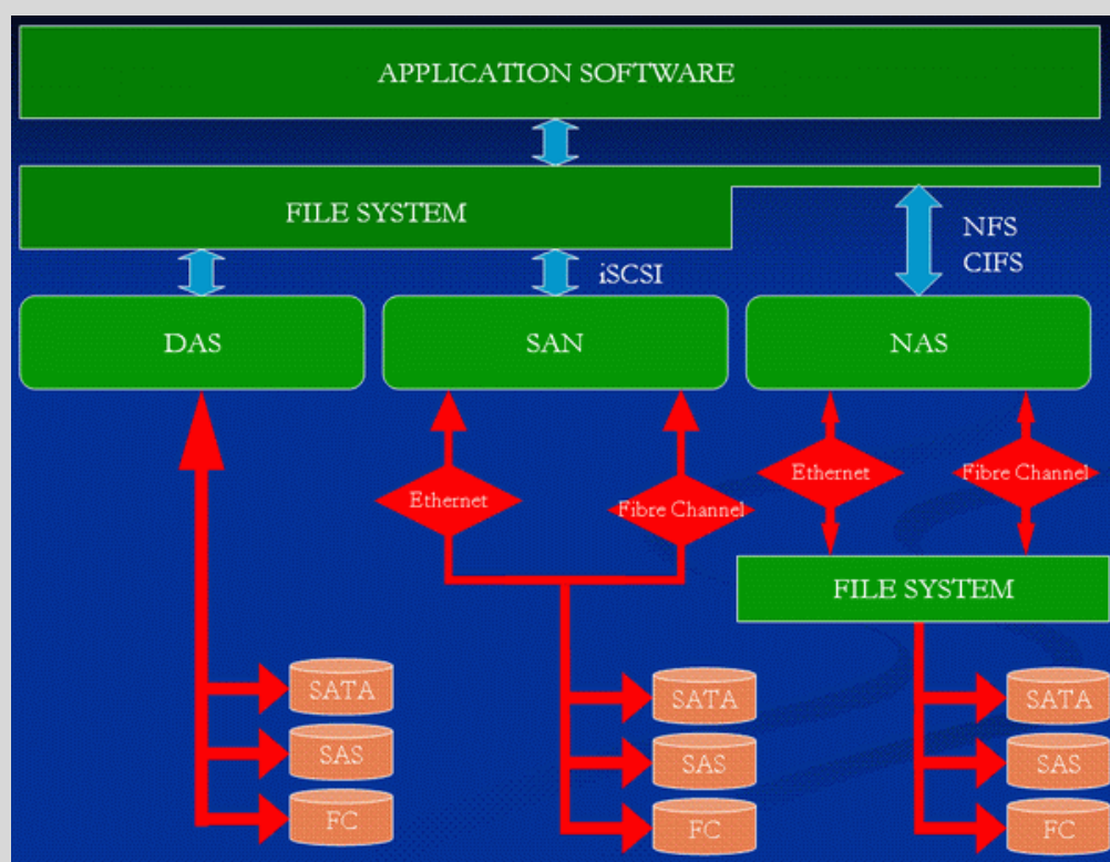
图 18.1-2、服务器取得文件系统的三个来源（数据源为 注 1 ）
