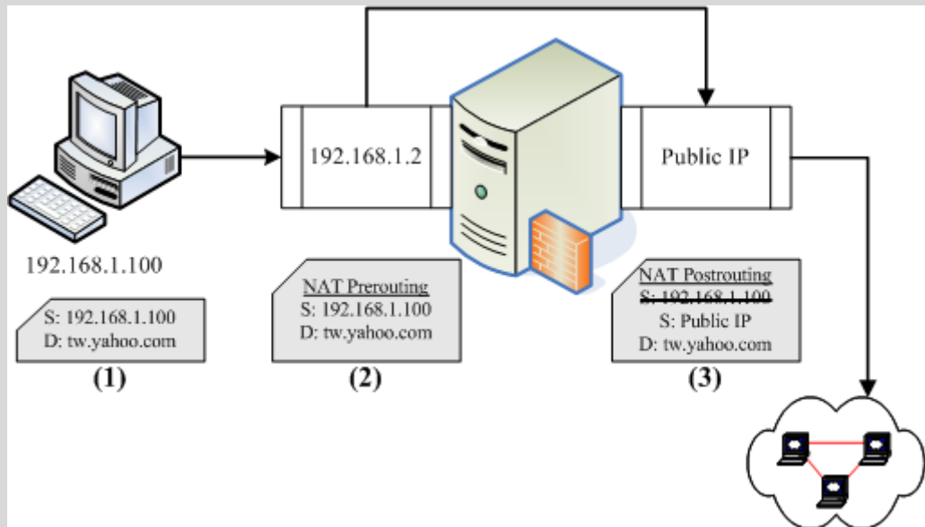
图 9.5-1、SNAT 封包传送出去的示意图
