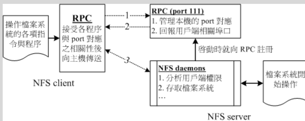
图 13.1-2、NFS 与 RPC 服务及文件系统操作的相关性
