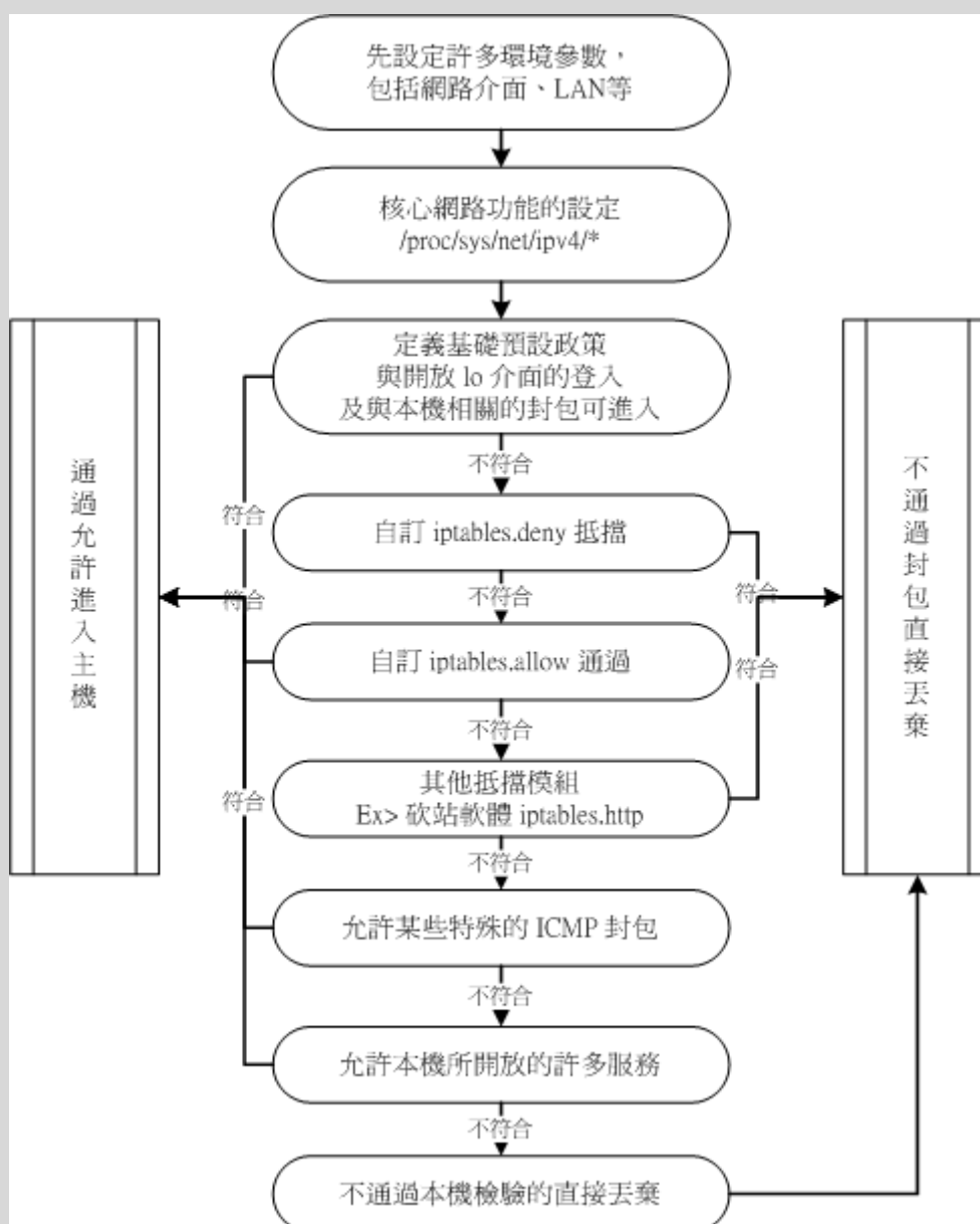
图 9.4-2、本机的防火墙规则流程示意图
