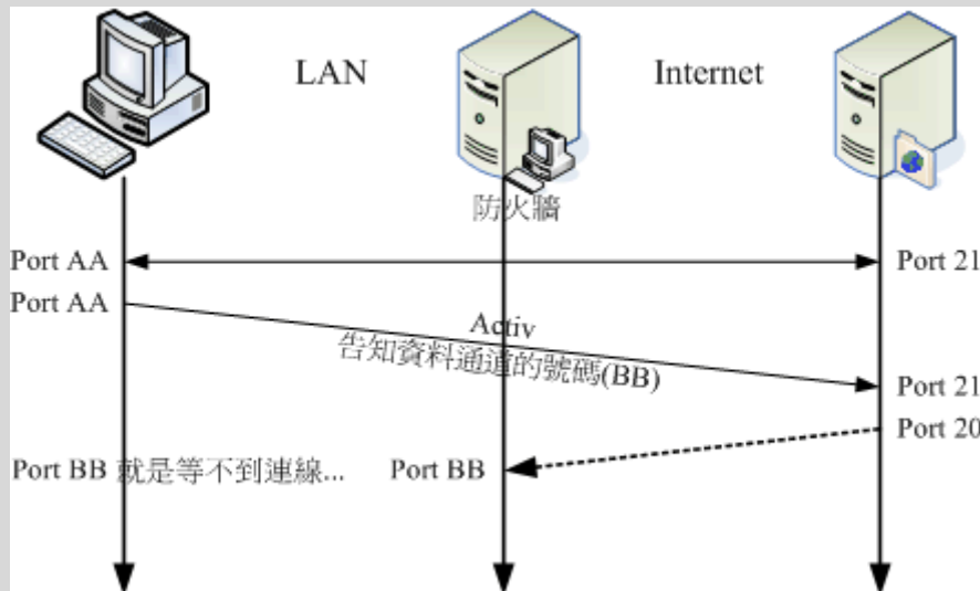
图 21.1-2、FTP 客户端与服务器端联机中间具有防火墙的联机状态
