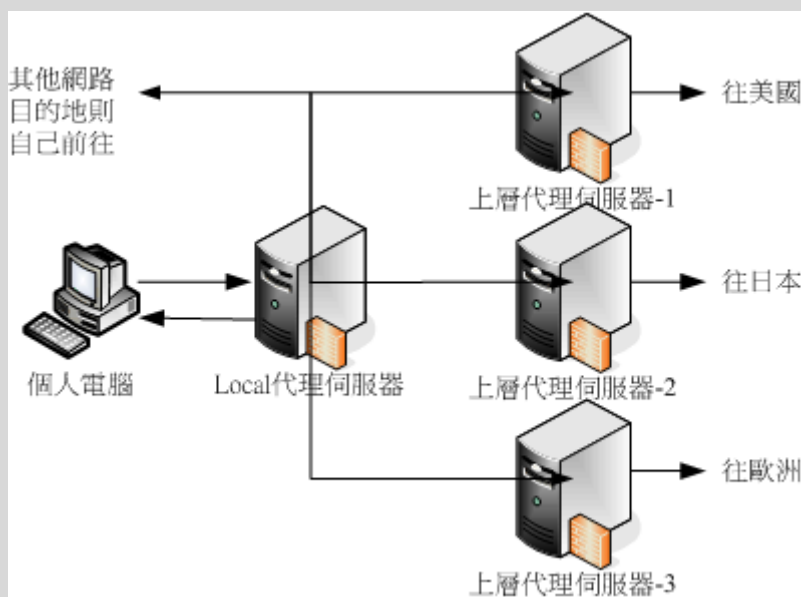
图 17.1-4、以多部上层代理服务器达到分流的效果示意图
