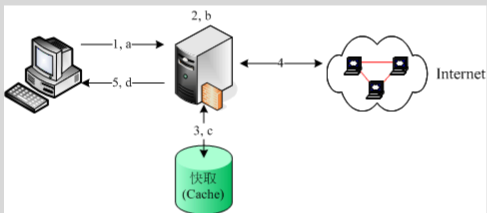
图 17.1-2、代理服务器的运作流程图：快取数据与客户端
