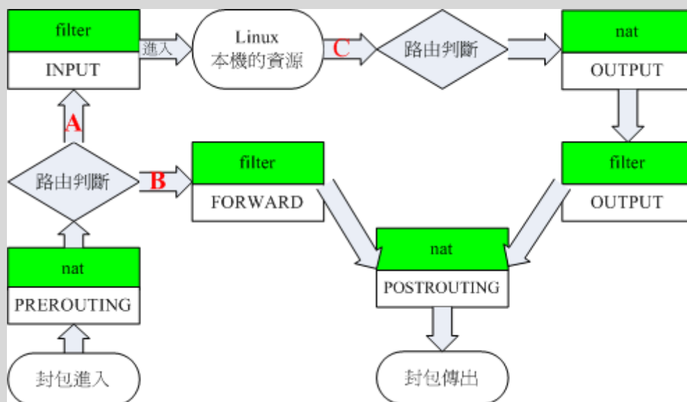
图 9.3-4、iptables 内建各表格与链的相关性(简图)
