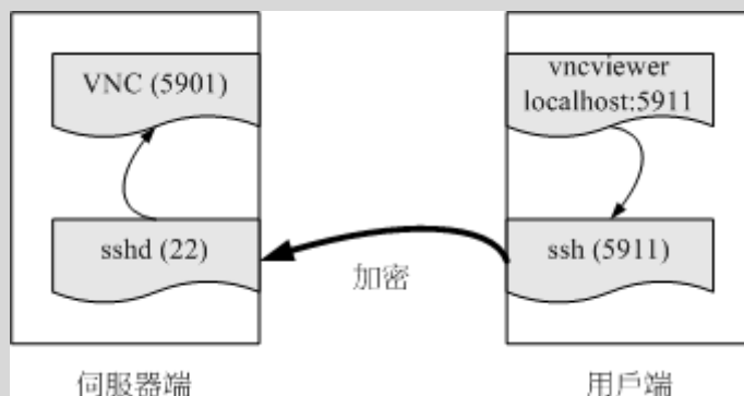
图 11.6-1、透过本地端的 ssh 加密联机到远程的服务器示意图
