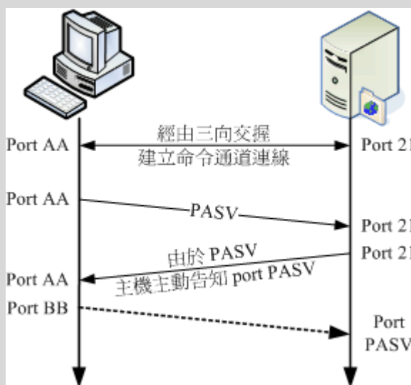
图 21.1-3、FTP 的被动式数据流联机流程
