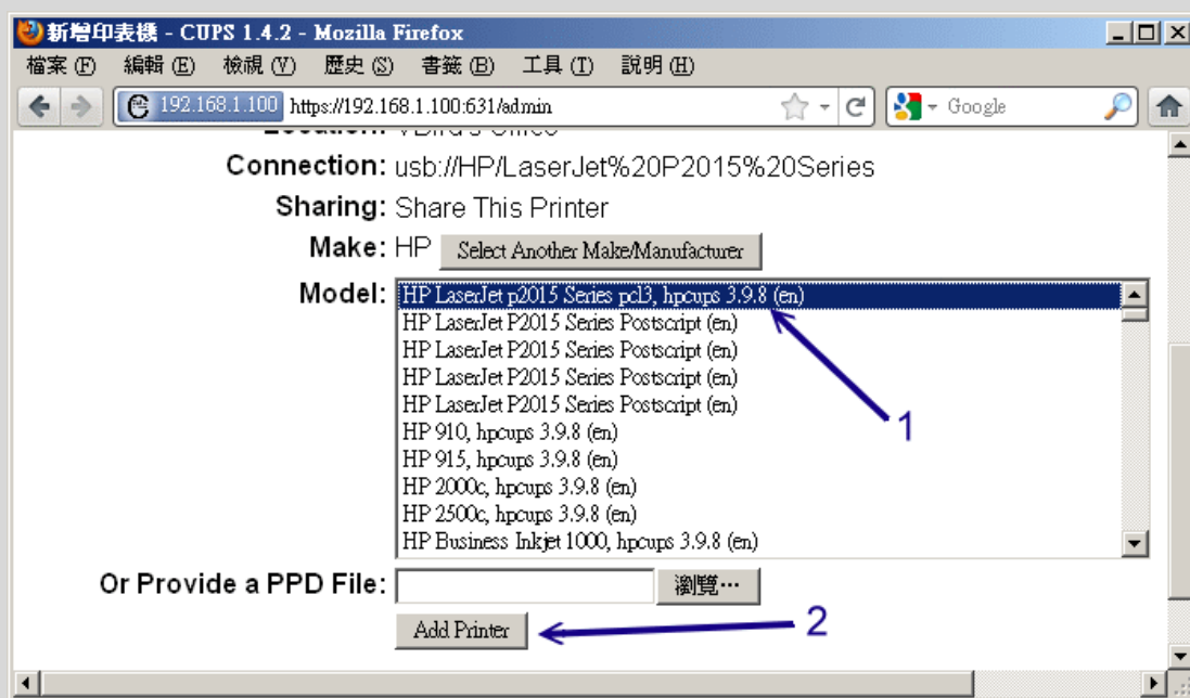
图 16.2-7、用 CUPS 设定 USB 打印机
