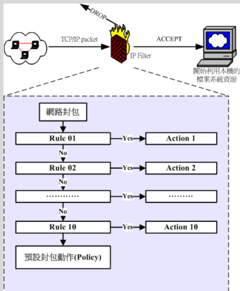
图 9.3-1、封包过滤的规则动作及分析流程
