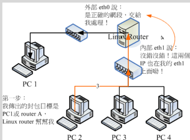
图 8.4-3、内部计算机想要传送到正常网域时的封包流向
