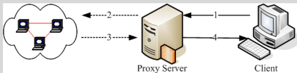
图 9.1-1、Proxy Server 的运作原理简介
