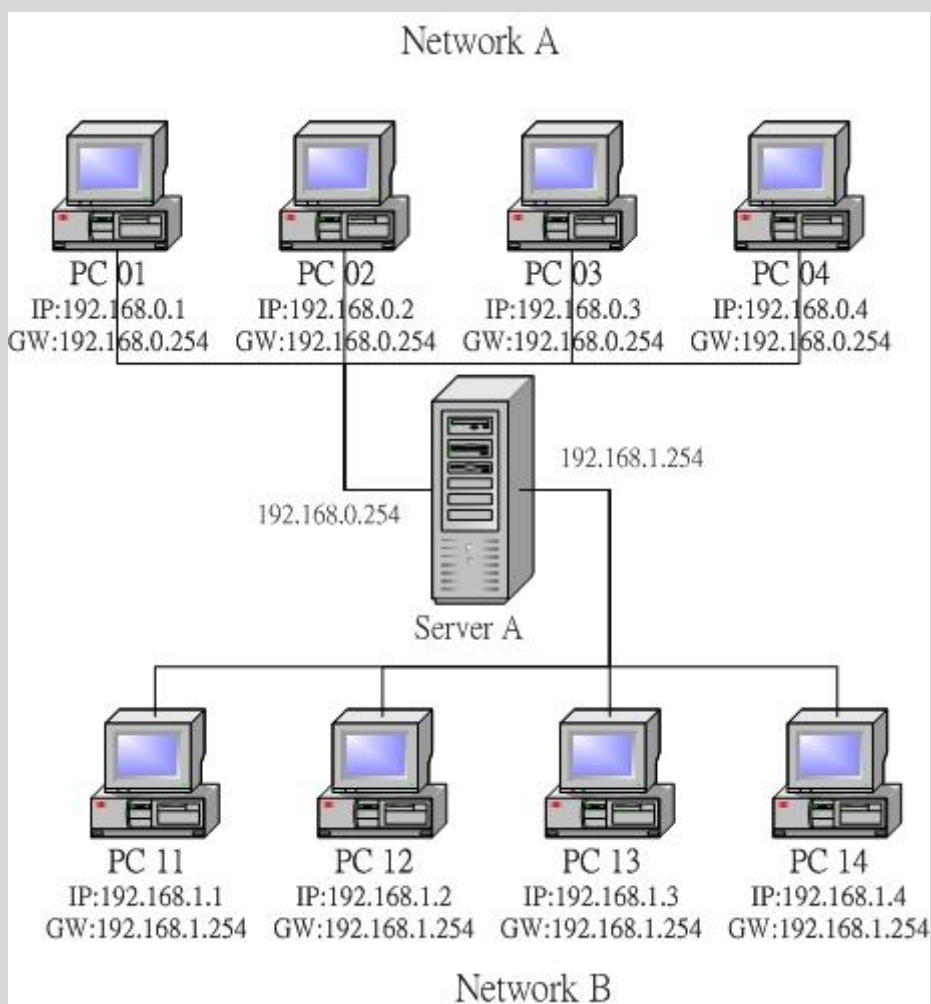
图 2.3-2、简易的路由示意图
