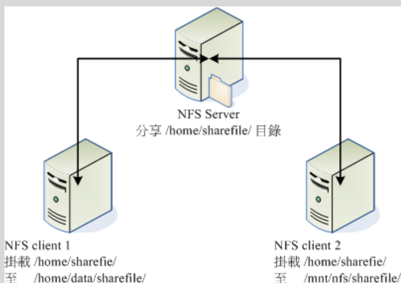
图 13.1-1、NFS 服务器分享目录与 Client 挂载示意图
