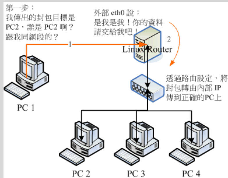
图 8.4-2、正常的网段想要传送到内部计算机去的封包流向
