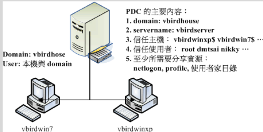
图 16.4-1、一个简易的 PDC 实作案例相关参数示意图
