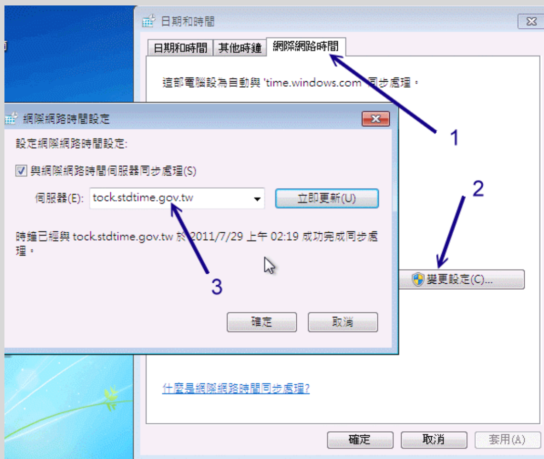
图 15.3-2、Windows 7 提供的网络校时功能
