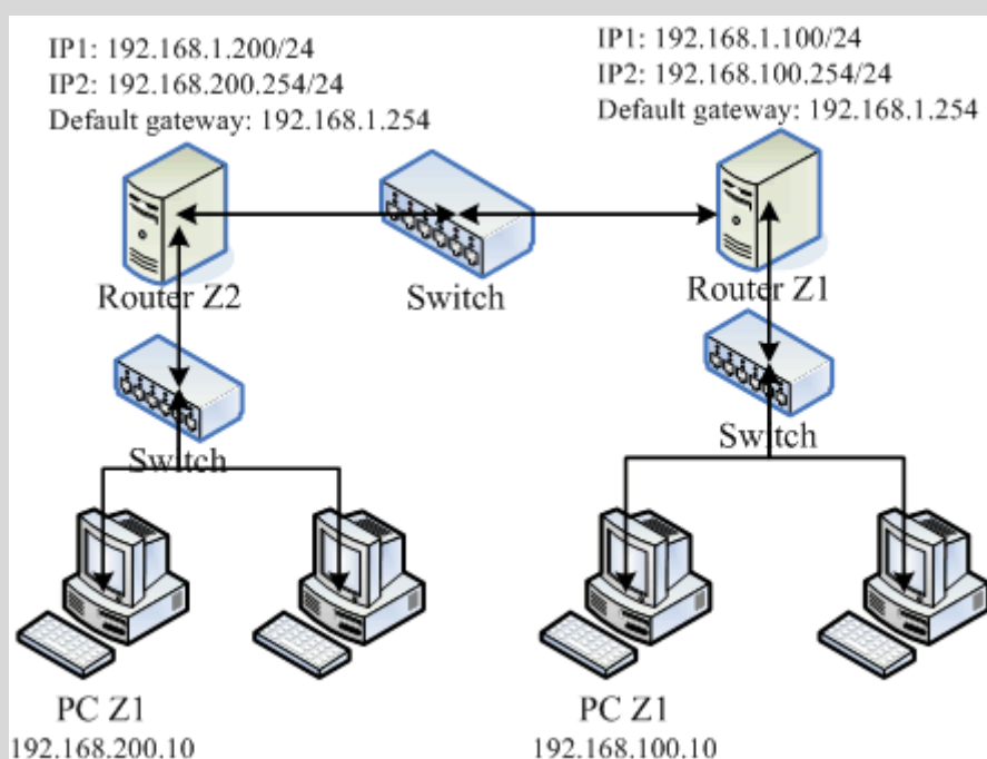
图 8.3-1、练习动态路由所设定的网络联机示意图
