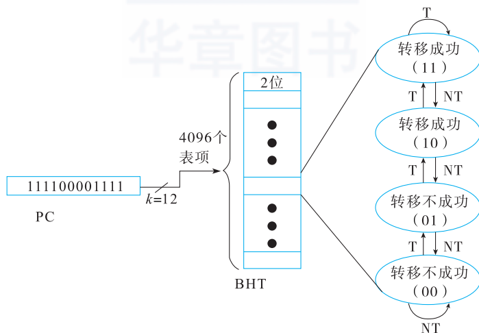
图 9.22 2 位 PHT 原理
