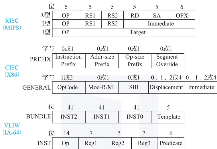
图 2.2 RISC、CISC、VLIW 指令编码特点
