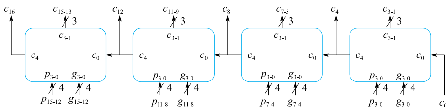
图 8.20 块内并行、块间串行的 16 位先行进位加法器的进位逻辑
