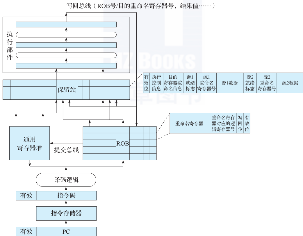
图 9.19 动态调度流水线结构示意图
