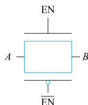
图 8.14 CMOS 电路：传输门
