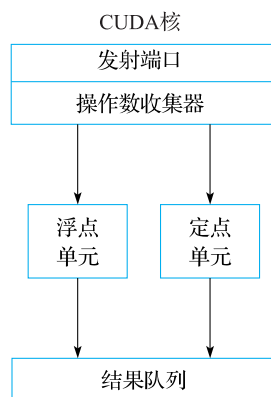
图 11.22 CUDA 核结构
