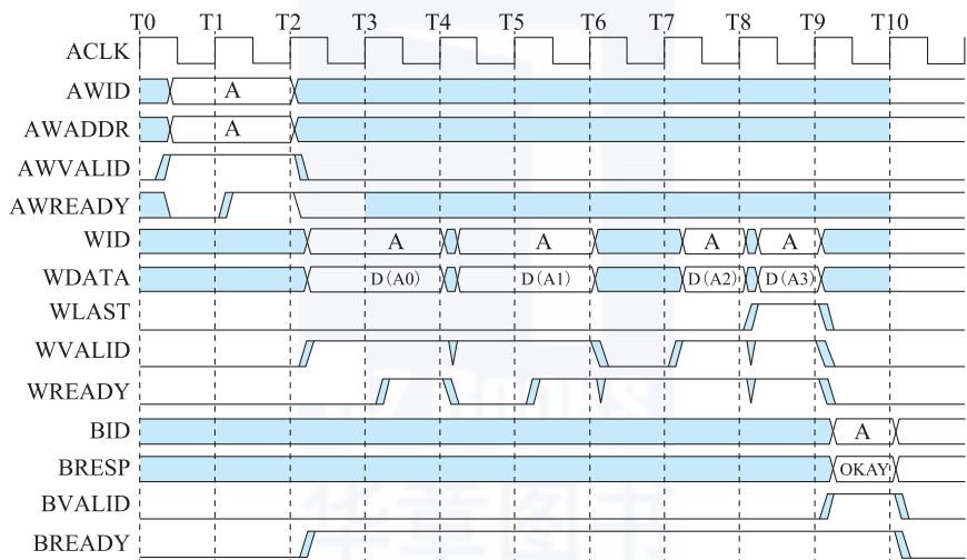
图 6.7 写事务
