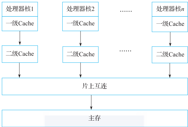
a) 私有Cache结构示意图
