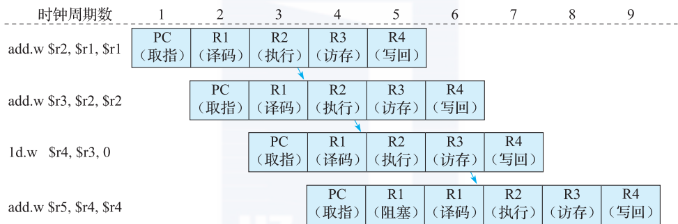
图 9.12 加入前递的数据相关时空图
