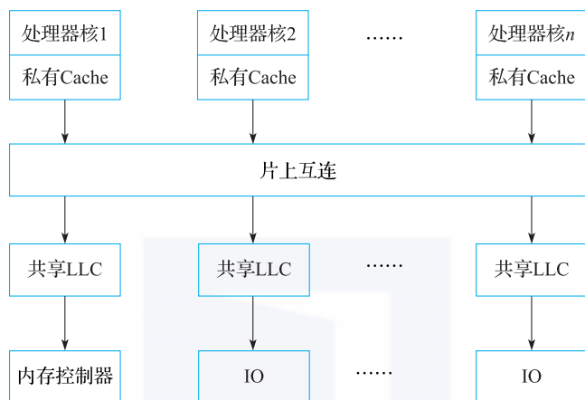
图 11.6 NUCA 架构多核处理器的片上互连
