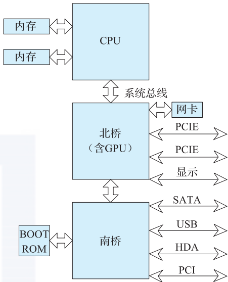
图 5.8 CPU-弱北桥-南桥结构
