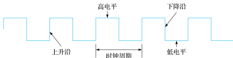
图 8.7 时钟信号
