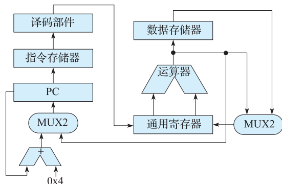
图 9.1 简单 CPU 的数据通路
