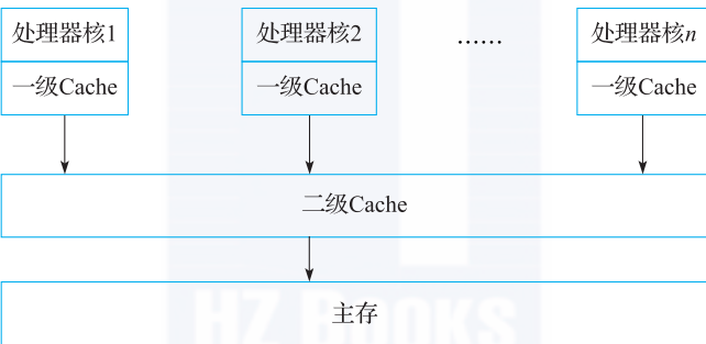
b) 共享Cache结构示意图
