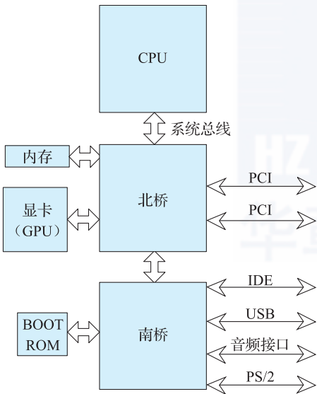
图 5.6 CPU-GPU-北桥-南桥结构
