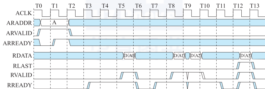
图 6.5 突发读事务
