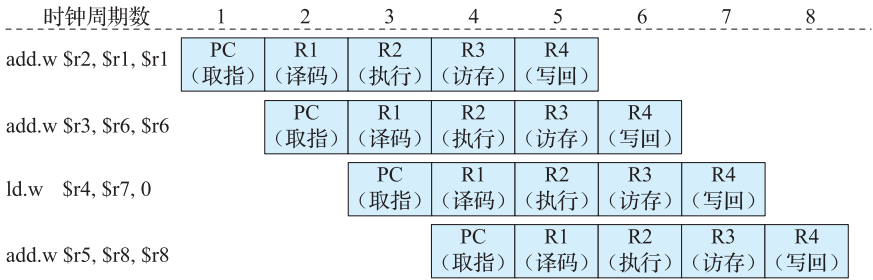
图 9.7 流水线处理器的流水线时空图
