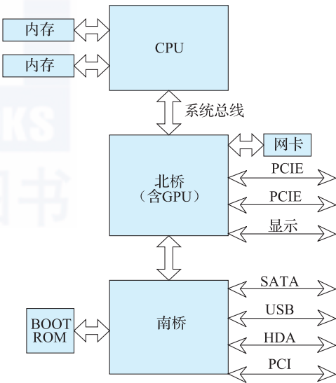
图 6.24 PCIe 接口位置示意图
