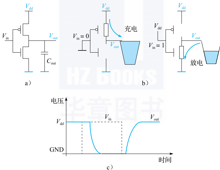
图 8.16 CMOS 反相器的延迟
