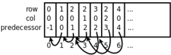
图 26.8. 广度优先搜索的队列数据结构
