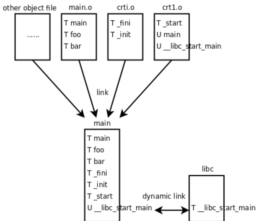
图 19.3. C程序的链接过程
