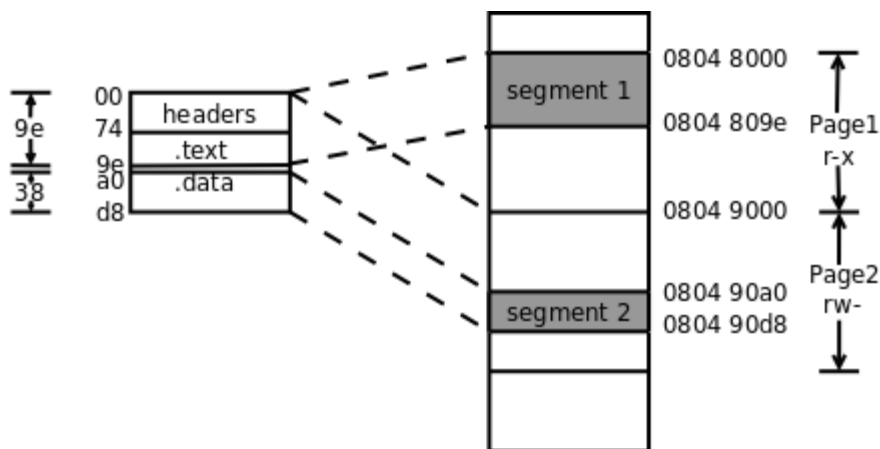
图 18.2. 文件和加载地址的对应关系
