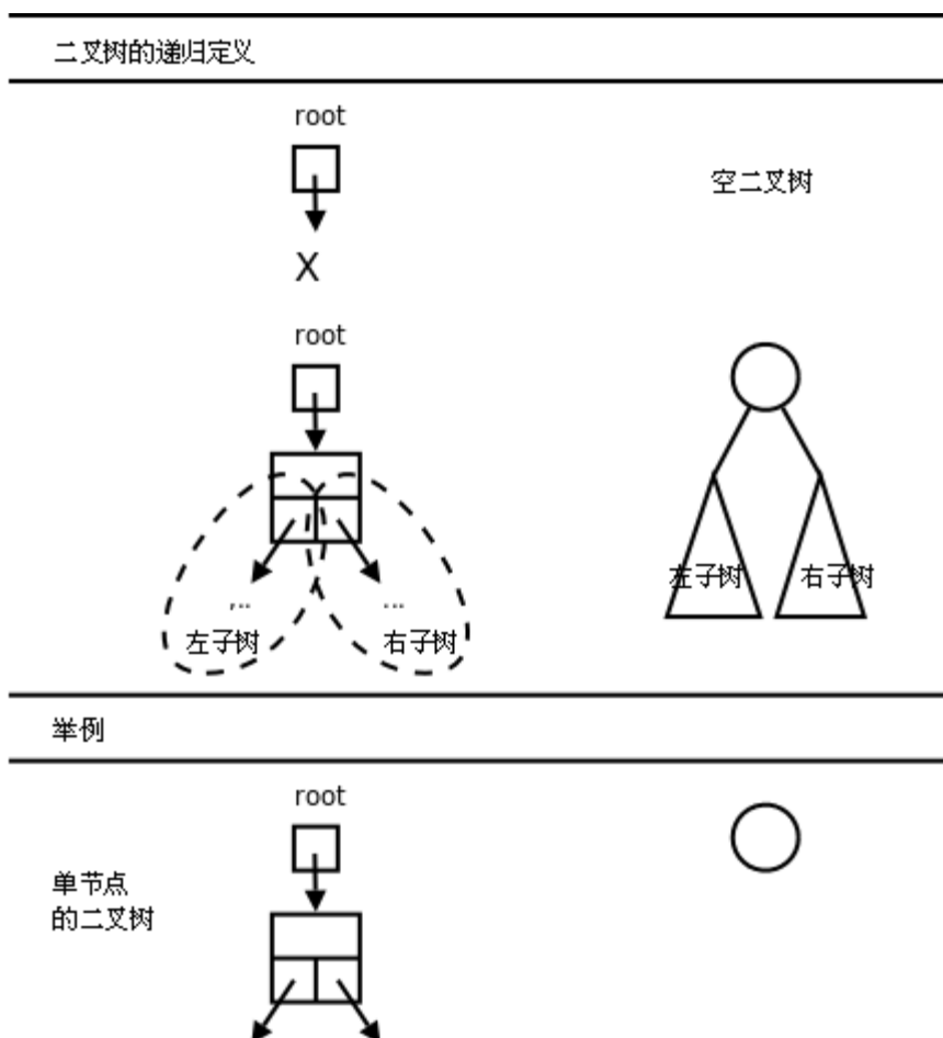
图 26.9. 二叉树的定义和举例
