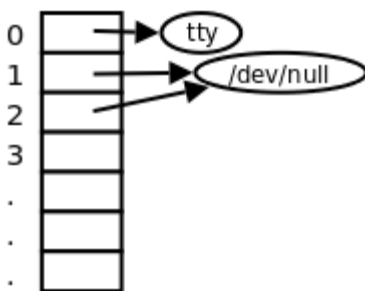
图 28.3. 重定向之后的文件描述符表
