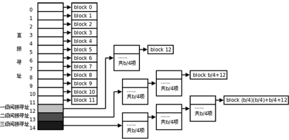
图 29.7. 数据块的寻址
