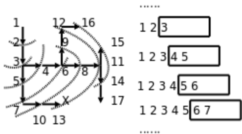
图 12.4. 广度优先搜索
