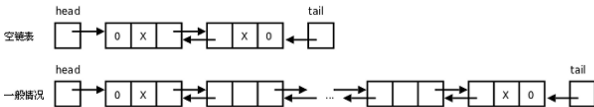
图 26.6. 带Sentinel的双向链表
