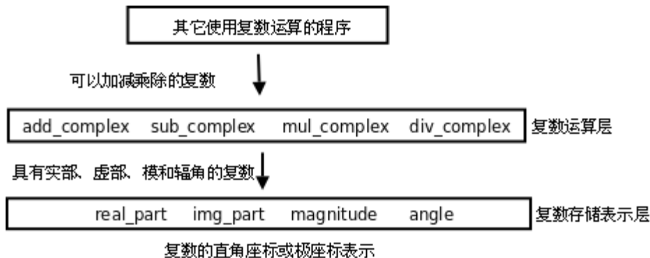
图 7.3. 数据抽象
