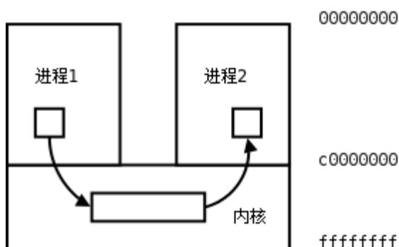
图 30.6. 进程间通信
