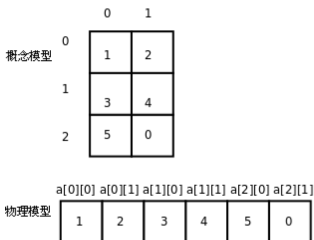
图 8.3. 多维数组
