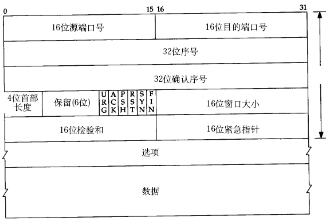
图 36.12. TCP段格式
