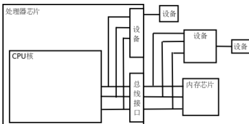
图 17.4. 设备
