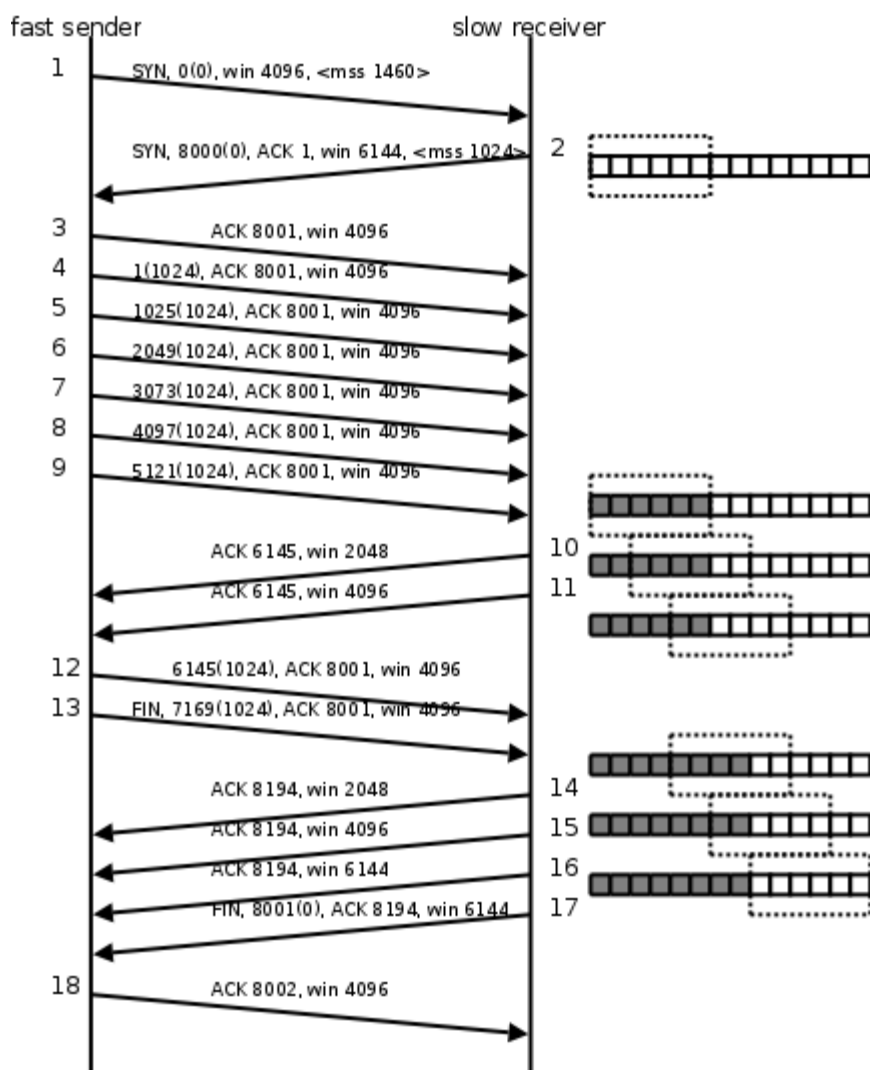
图 36.14. 滑动窗口
