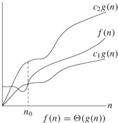
图 11.2. \Theta -notation
