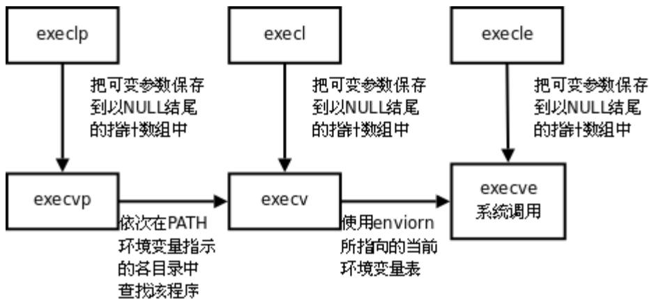
图 30.5. exec函数族
