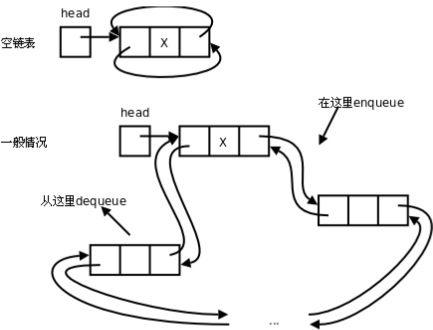
图 26.7. 环形链表
