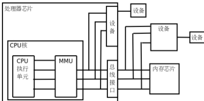
图 17.6. 虚拟地址
