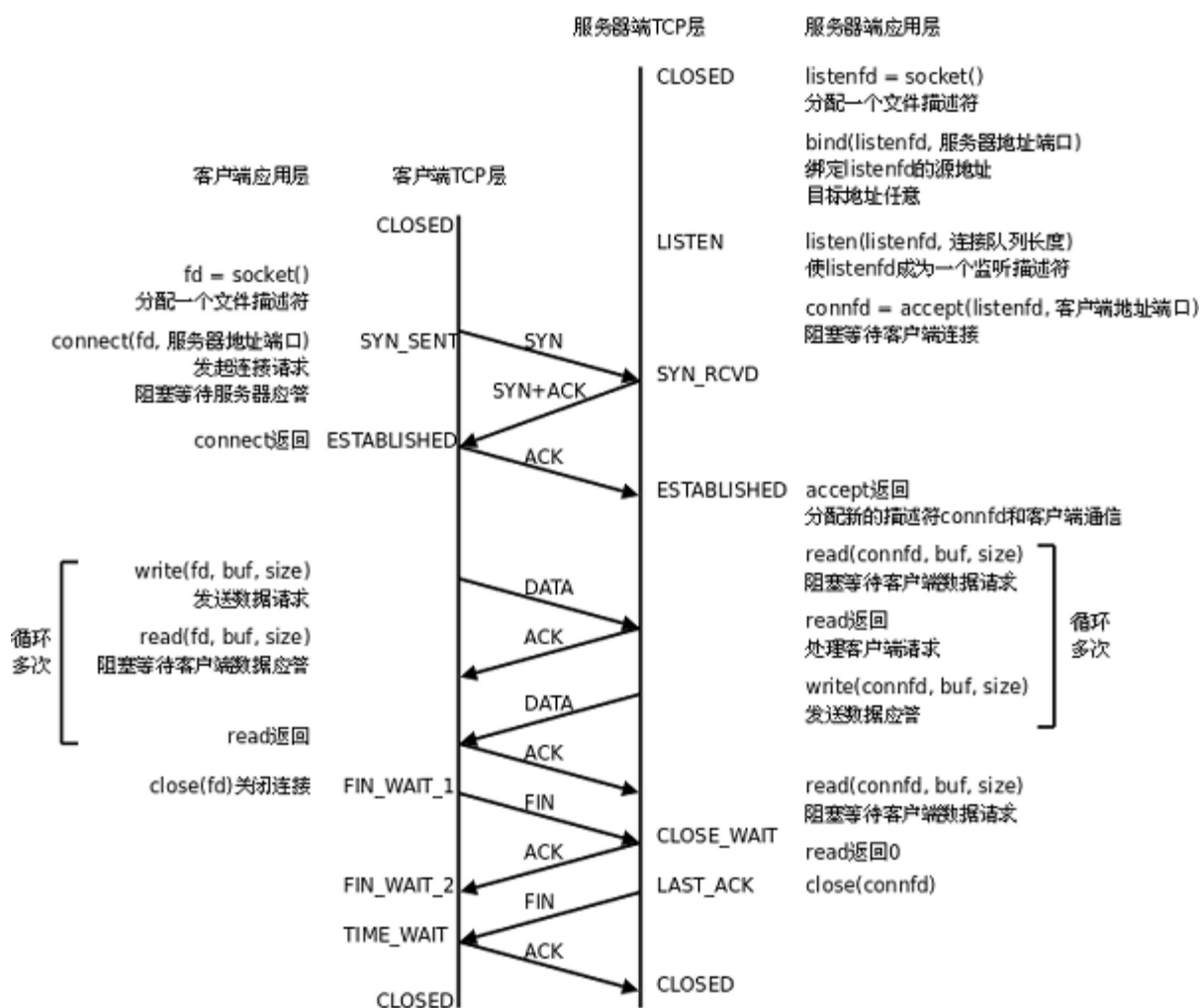
图 37.2. TCP协议通讯流程
