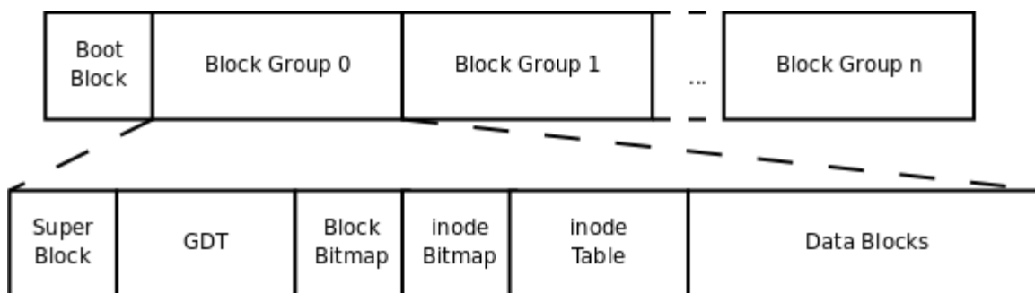
图 29.2. ext2文件系统的总体存储布局
