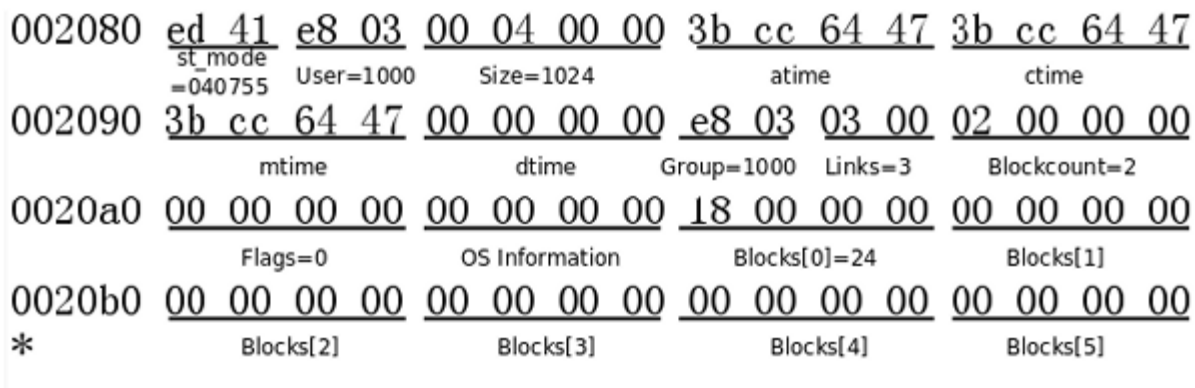
图 29.5. 根目录的inode
