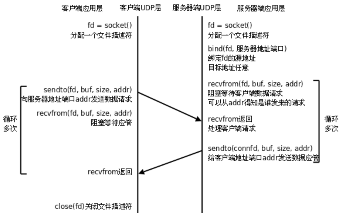
图 37.3. UDP通讯流程
