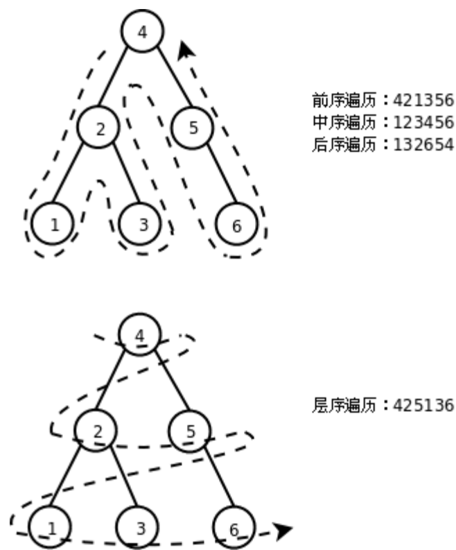
图 26.10. 二叉树的遍历
