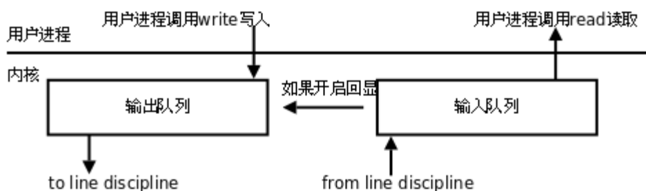
图 34.2. 终端缓冲
