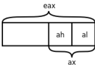
图 19.7. eax寄存器
