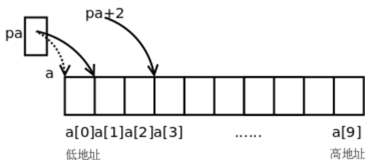
图 23.3. 指针与数组
