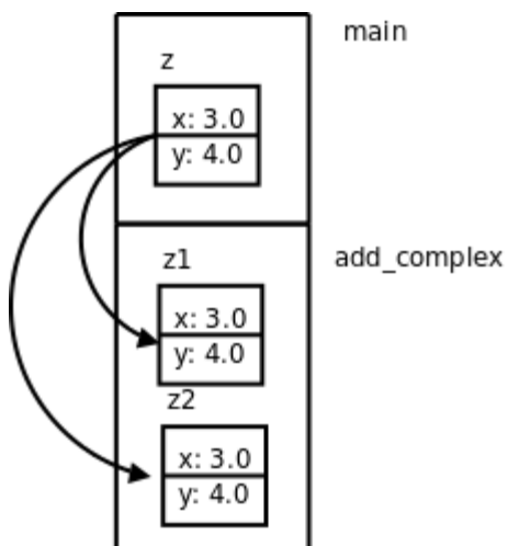
图 7.2. 结构体传参
