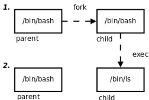
图 30.1. fork/exec
