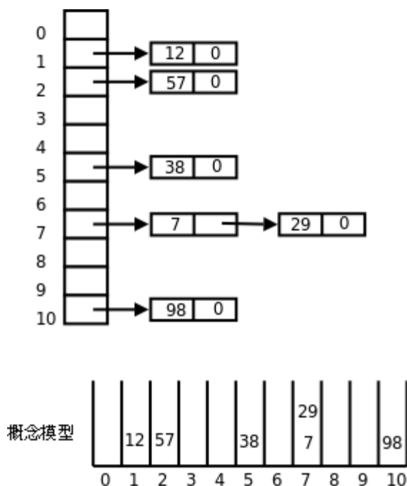
图 26.12. 哈希表
