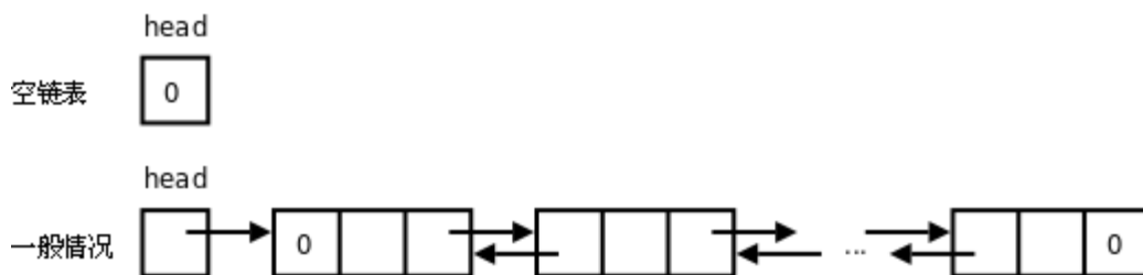
图 26.5. 双向链表
