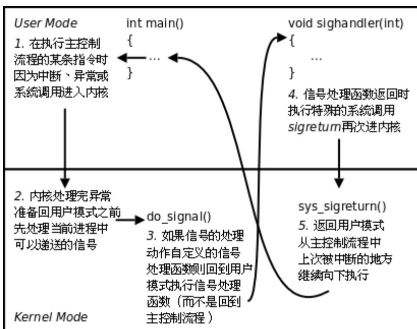
图 33.2. 信号的捕捉
