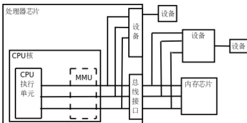
图 17.5. 物理地址
