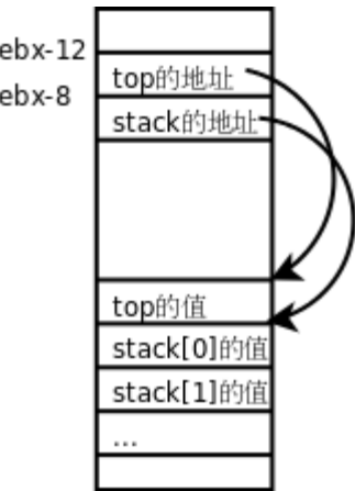
图 20.3. 间接寻址
