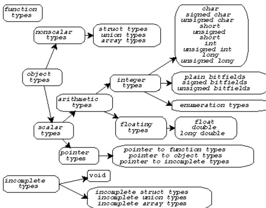
图 23.5. C语言类型总结
