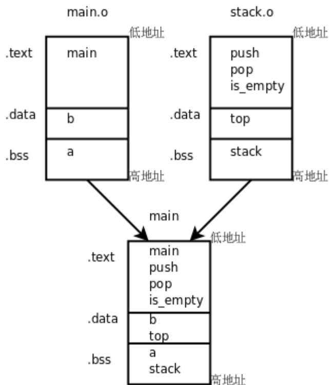
图 20.1. 多目标文件的链接
