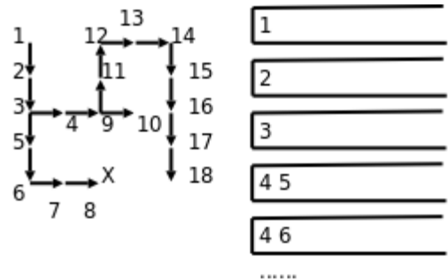
图 12.2. 深度优先搜索
