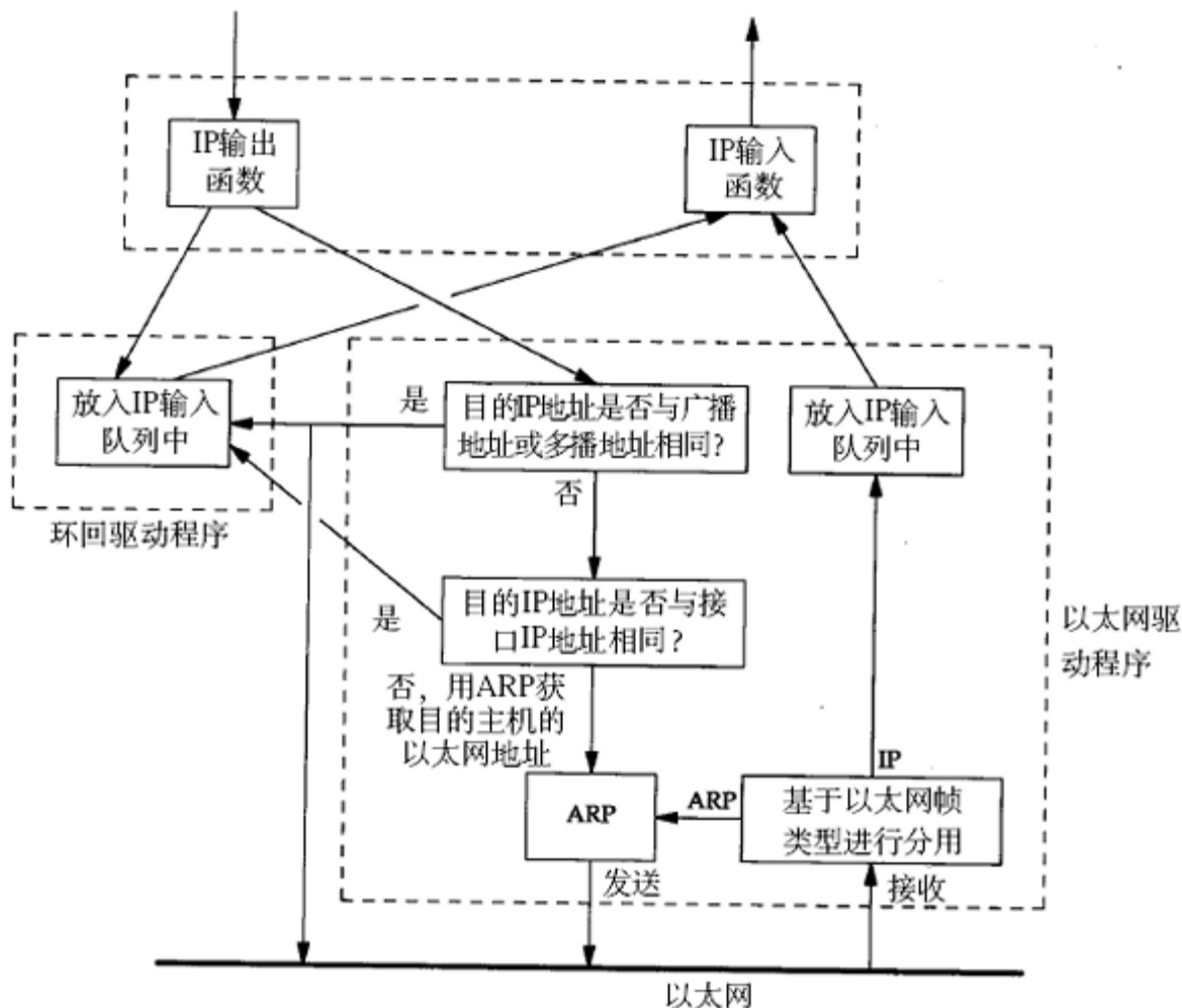
图 36.10. loopback设备
