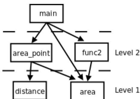
图 5.1. 函数的分层设计
