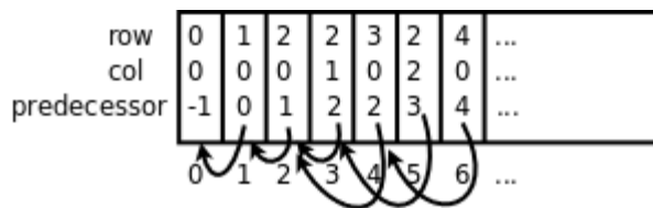
图 12.3. 广度优先搜索的队列数据结构
