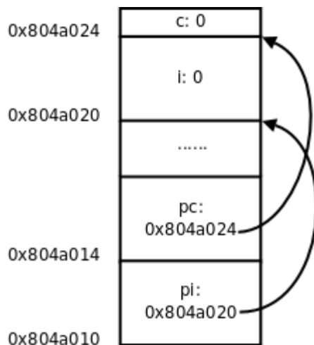
图 23.1. 指针的基本概念
