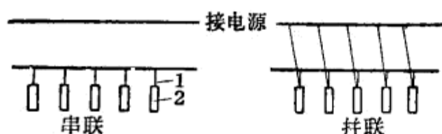
图135 串联和并联
