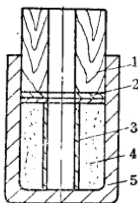
圖94 試驗彈體
