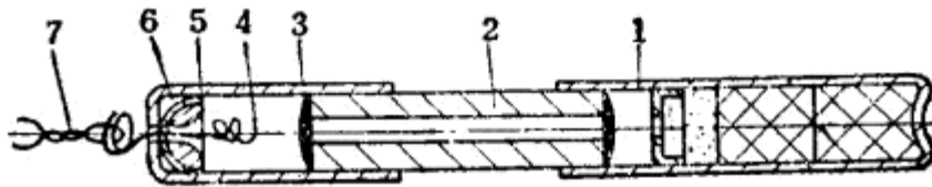
图77 拉火裝置
