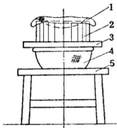
图8 雷汞洗涤装置
