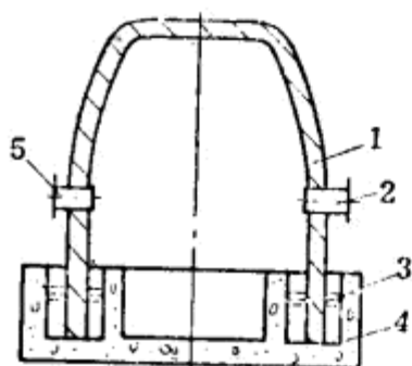
图153 气包
