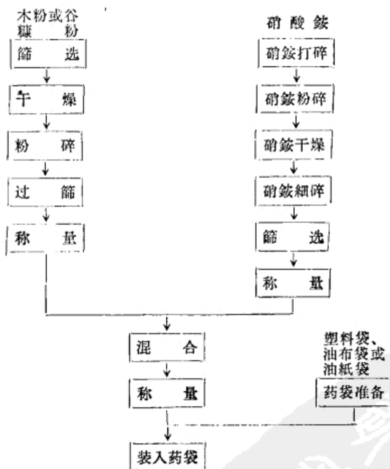
流程11 “第三类型”不含敏感剂的硝酸铵炸药生产工艺流程
