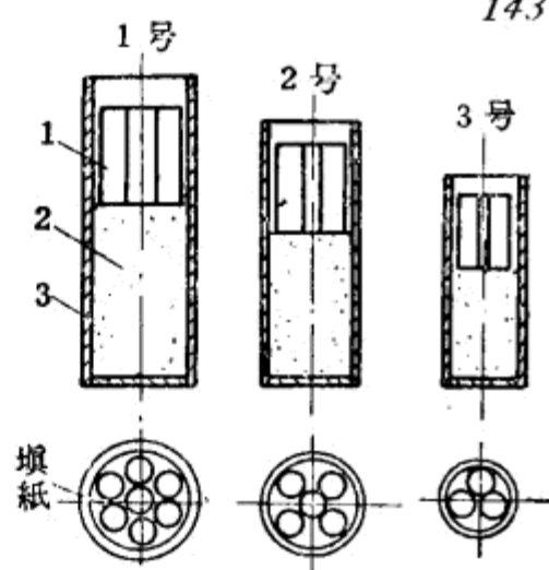
图116 导爆管
