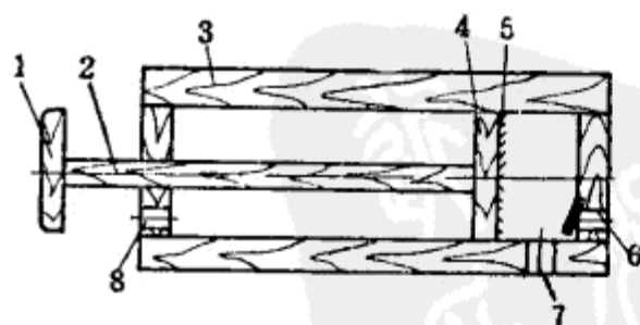
图152 風箱
