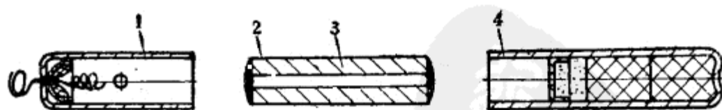
图87 拉火装置合装
