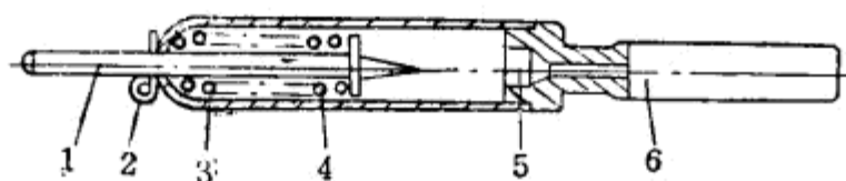
图113 击发式拉火
