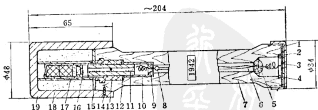
圖69 木柄手榴彈
