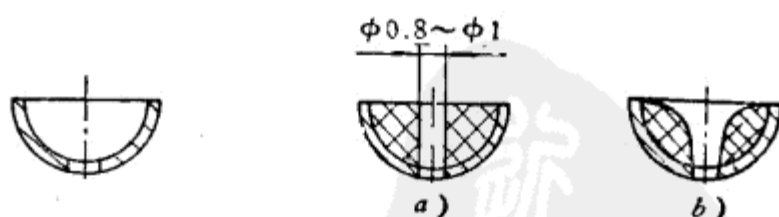
图81 拉火帽壳
