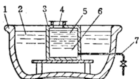
图128 熔磷槽
