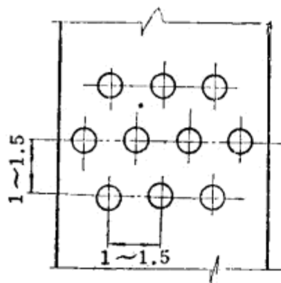
图117 公路布雷
