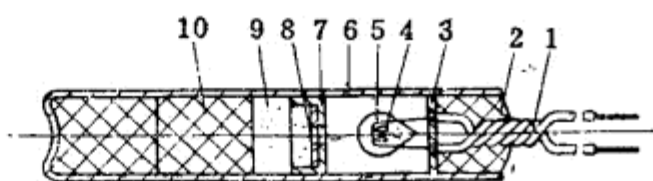
图51 电雷管
