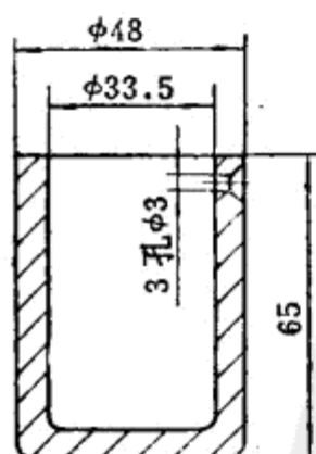
图74 弹壳
