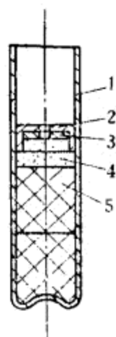
图35 火雷管 1—壳体； 2—加强帽； 3—綢垫； 4—起爆药； 5—烈性炸药。
