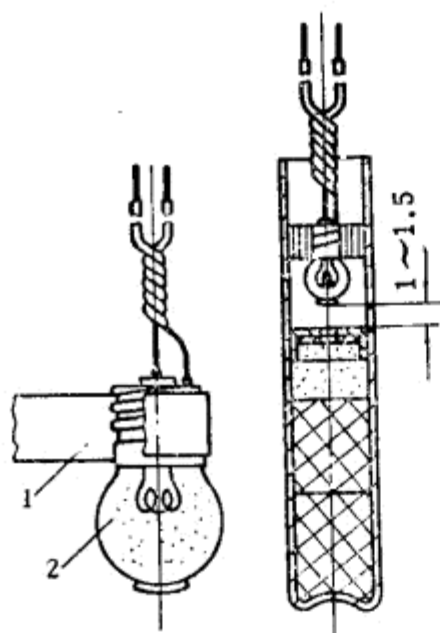
图61 纏紙条 图62 电发 1—紙条; 2—灯泡。 火装配
