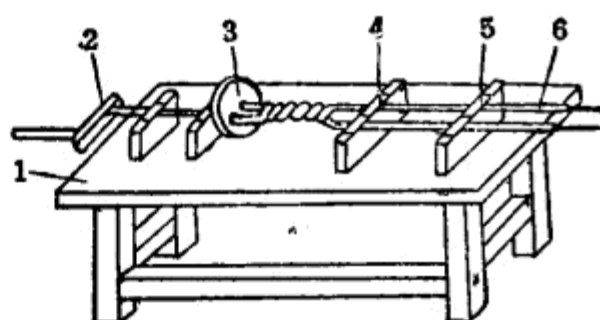
图56 擰紧工具
