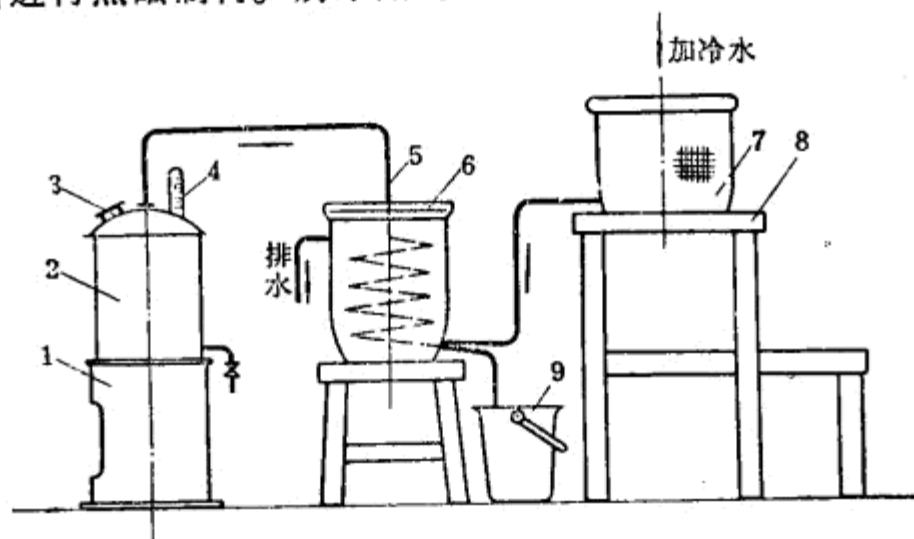
图3 酒精蒸餾装置
