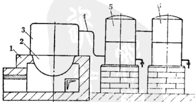
图160 缸法制造硝酸的装置
