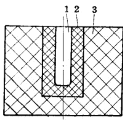
图115 扩爆药柱
