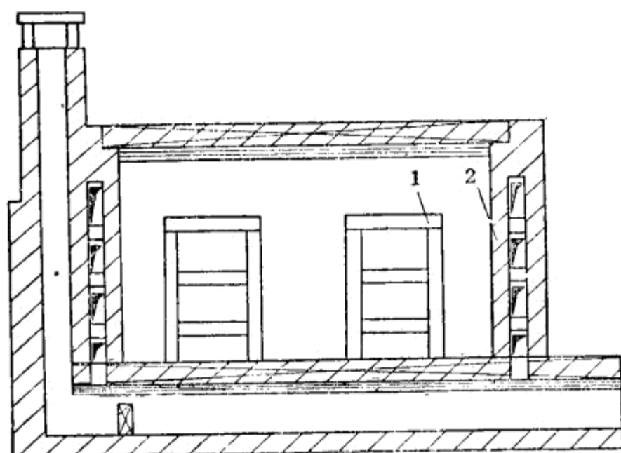
图10 火墙干燥室
