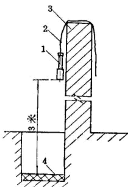
图96 成品安全性試驗
