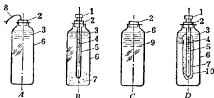
图126 燃燒瓶
