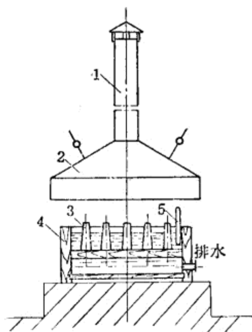
图 5 硝酸汞預溫槽
