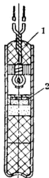
图64 灌硫磺封口 1—硫磺；2—雷管。
