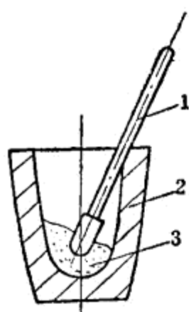
图30 人工捣碎工具
