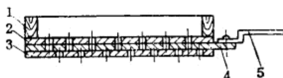
图41 装药板
