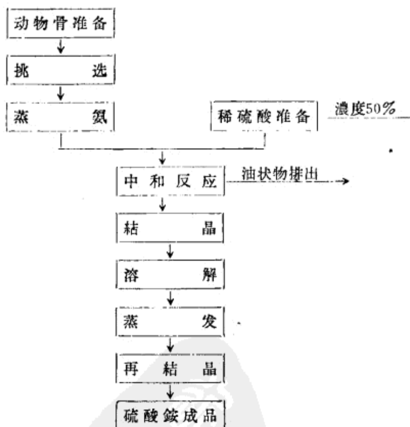
流程 7 用动物骨干錙制造硫酸銨的工艺流程
