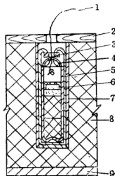
图114 拉发式拉火
