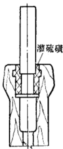
图92 灌硫磺
