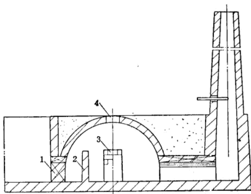
图33 燒炭窑
