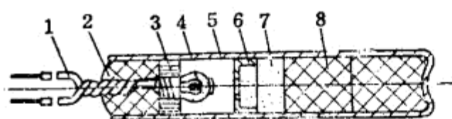
图52 纸壳电雷管
