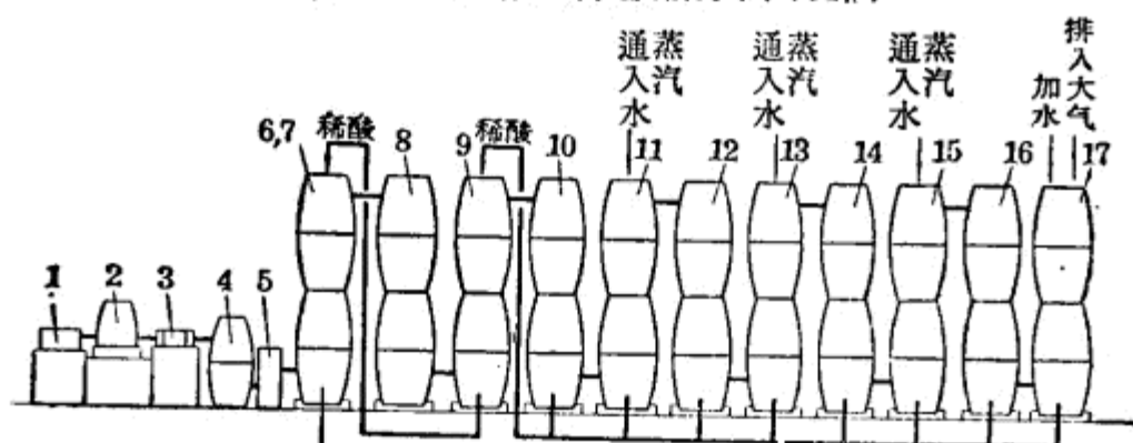
图151 缸塔法制造硫酸的立面视图
