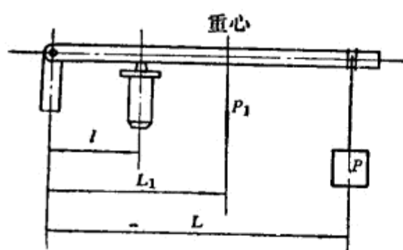
图43 杠杆原理
