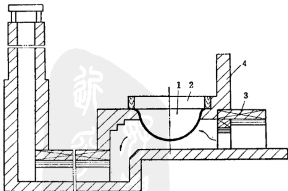
圖16 油脂皂化鍋
