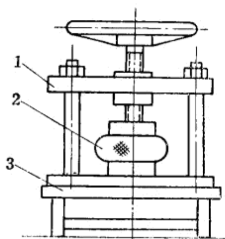
图 9 手扳压力机除水
