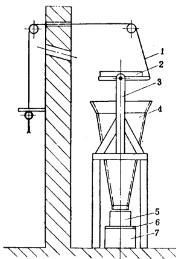
图12 倒药装置
