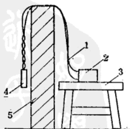
图65 起爆試驗 1—母綫；2—干電池或手搖發電機； 3—工作台；4—電雷管；5—牆。
