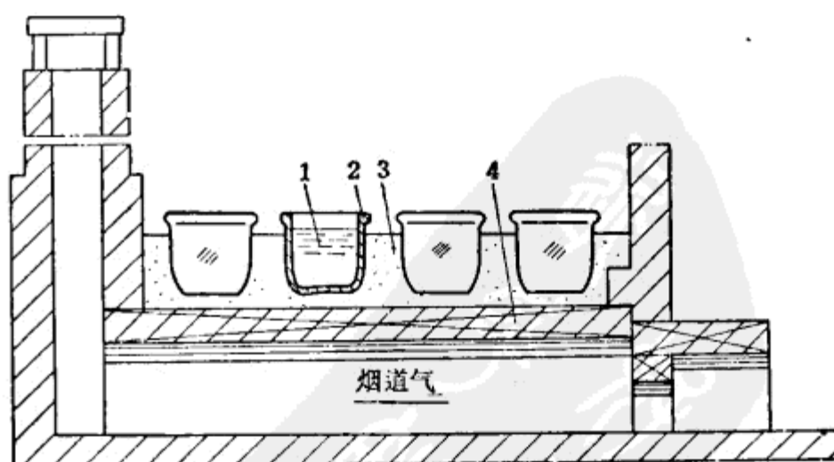
图27 火炕砂盘干燥装置
