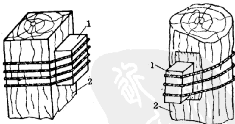
图149 炸毀木柱时药包的敷設方法
