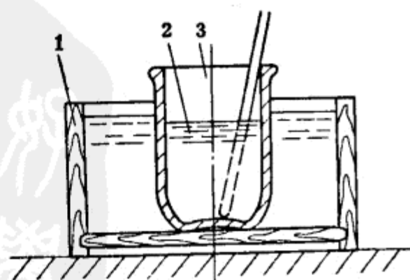
图19 配酸装置
