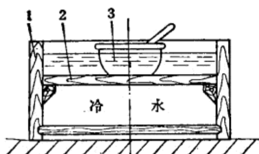
图20 硝化槽
