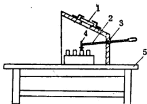
图47 擦管内壁浮药装置
