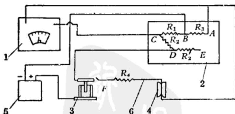
圖 66 接綫圖
