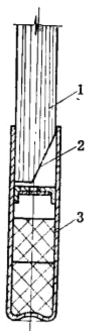
图133 导火綫插入火雷管。
