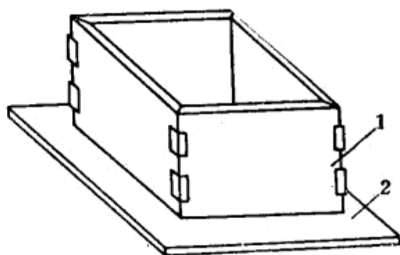
图17 装配槽 1—槽体；2—底板。
