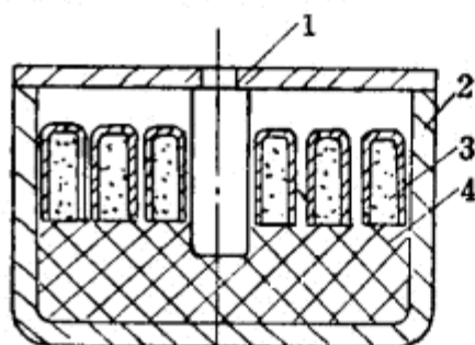
图107 子母雷
