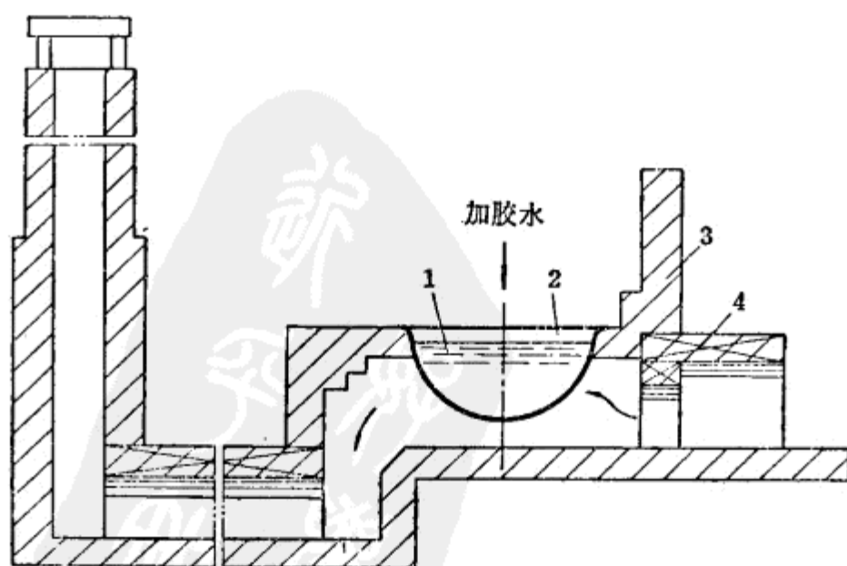
图21 熬硝
