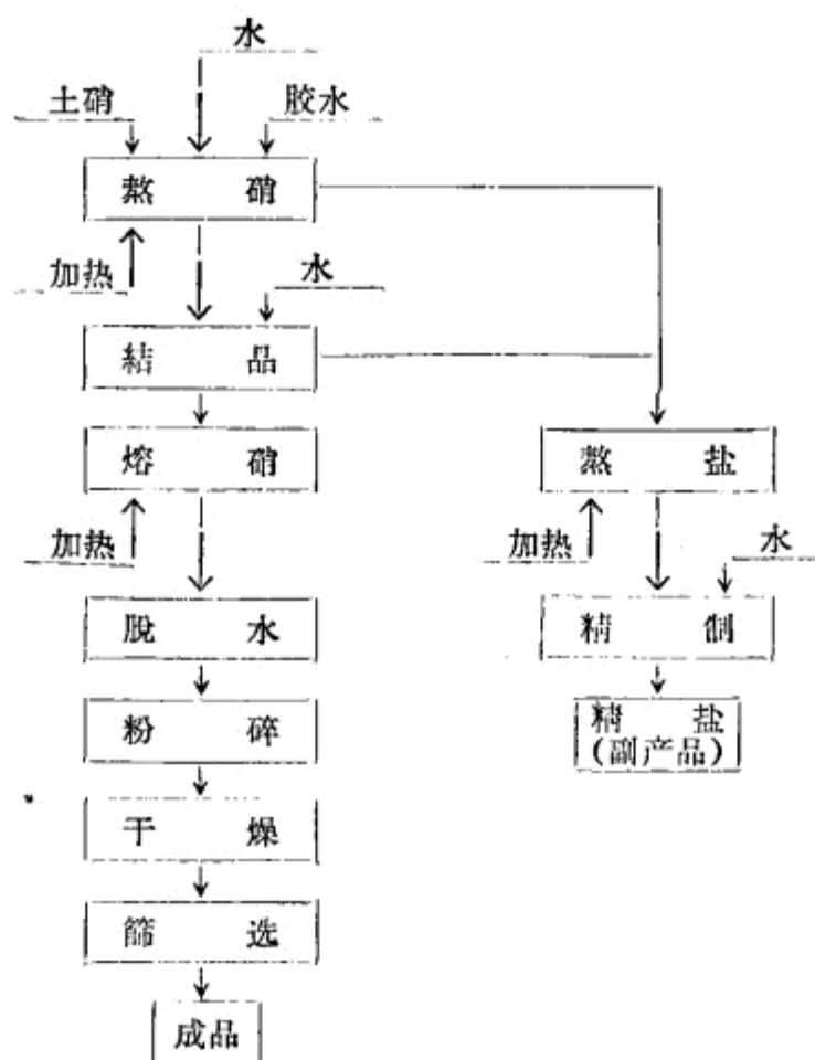
流程 4 火硝精制提纯工艺流程
