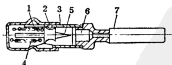
图112 压发机构
