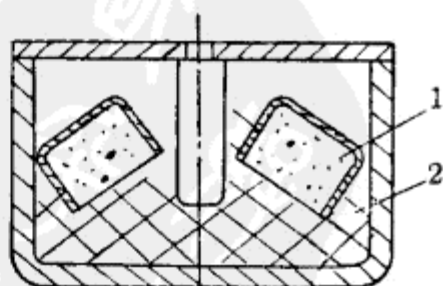
图109 子母雷
