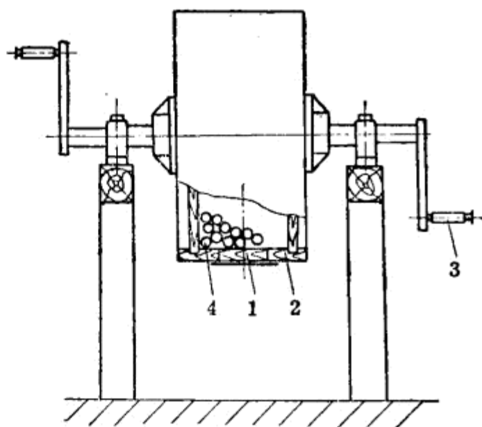
图24 人工球磨机
