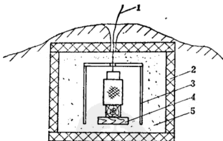
圖95 破片試驗
