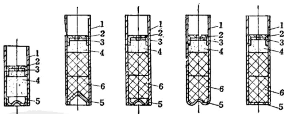
图37 纸壳火雷管
