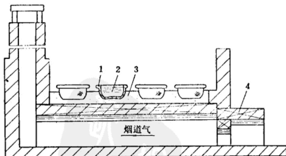
图18 甘油蒸濃沙盘
