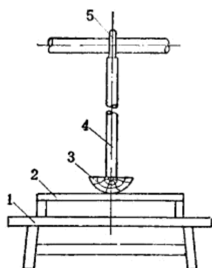
图38 搓管工具
