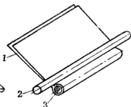
图138 捻芯子 1—紙；2—金屬棒； 3—黑火药。
