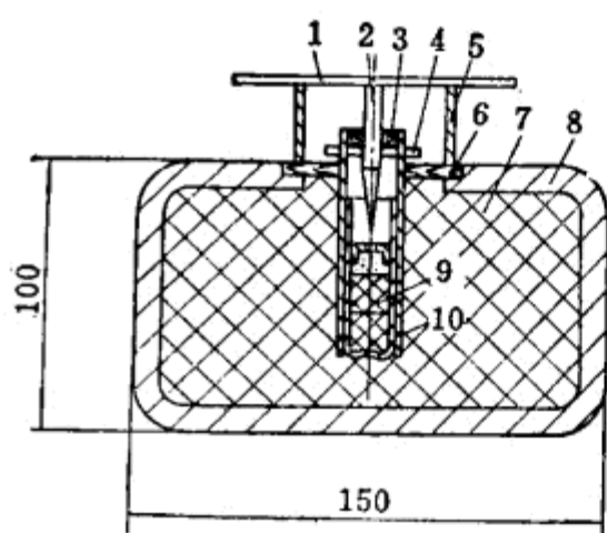
图97 压发地雷
