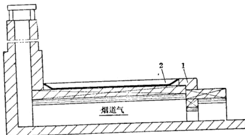
图31 烟道气干燥法
