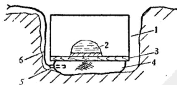
图131 燃燒地雷
