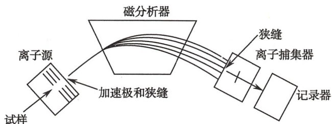
图 3-22 单聚焦质谱仪工作示意图
