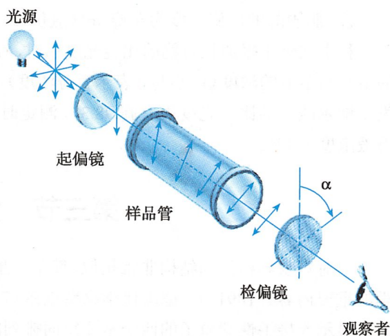
图 2-6 旋光仪的简图
