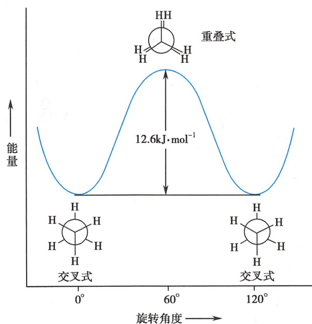
图 4-5 乙烷分子构象的能量曲线
