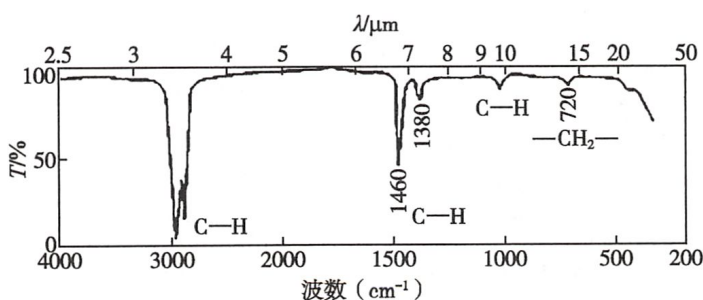
图 3-6 正己烷的红外光谱
