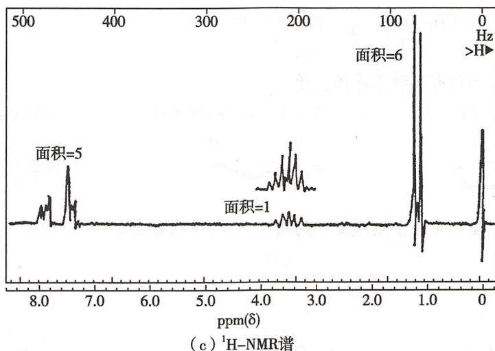
图 3-25 未知物的 UV、IR 和 ^1\text{H} -NMR 谱(续)
