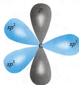
图1-6 sp^2 杂化碳的构型
