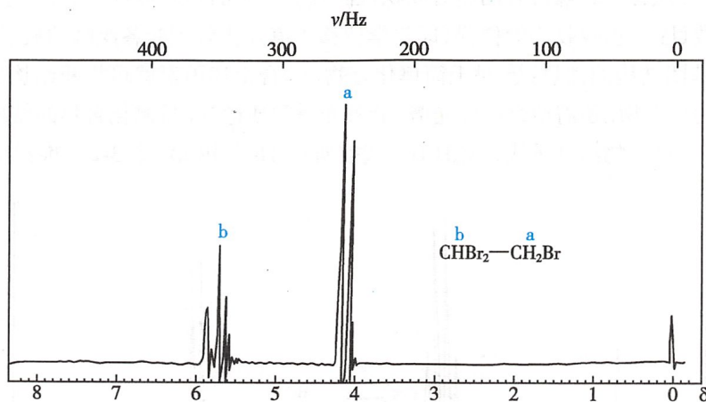
图 3-20 1,1,2-三溴乙烷的 ^1\text{H-NMR} 谱
