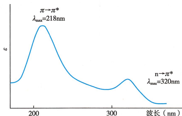
图 3-3 丙烯醛的紫外光谱
