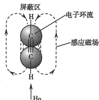
图 3-18 乙炔质子的屏蔽效应
