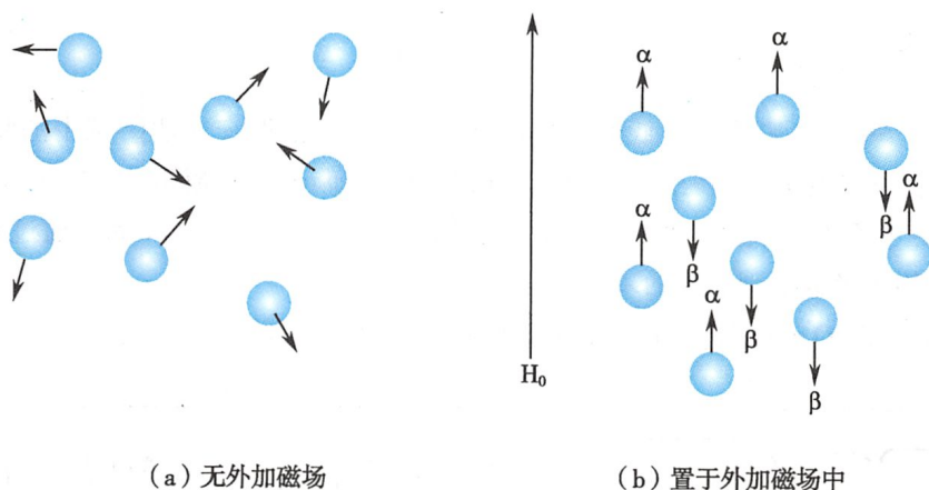
图 3-14 氢核的自旋取向
