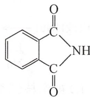
邻苯二甲酰亚胺 phthalimide
