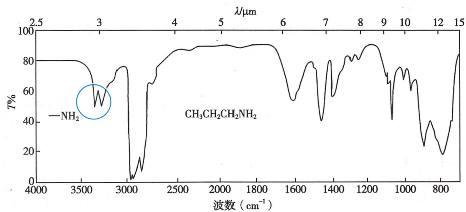
(a) 伯胺的红外光谱
