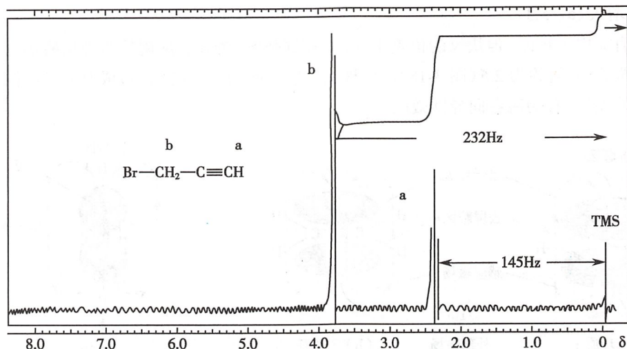
图 3-16 3-溴丙炔的 ^1\text{H} -NMR 谱图
