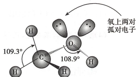
图 8-1 甲醇的结构
