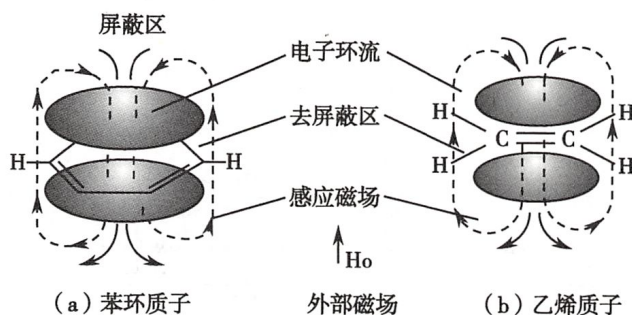
图 3-17 苯环和乙烯质子的去屏蔽效应示意图
