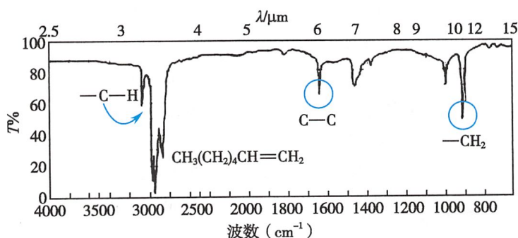
图 3-7 1-庚烯的红外光谱
