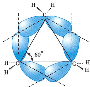
图 4-11 环丙烷分子中的“弯曲键”
