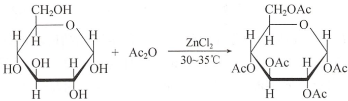
1,2,3,4,6-五乙酰基- \alpha -D-吡喃葡萄糖
