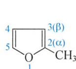
2-甲基呋喃 ( \alpha -甲基呋喃) 2-methylfuran
