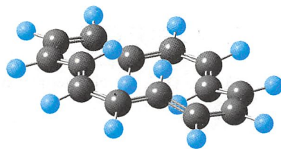
[14]-轮烯的球棒模型
