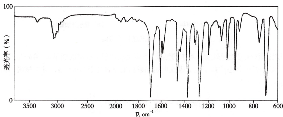
图 3-13 化合物 C_8H_8O 的红外光谱
