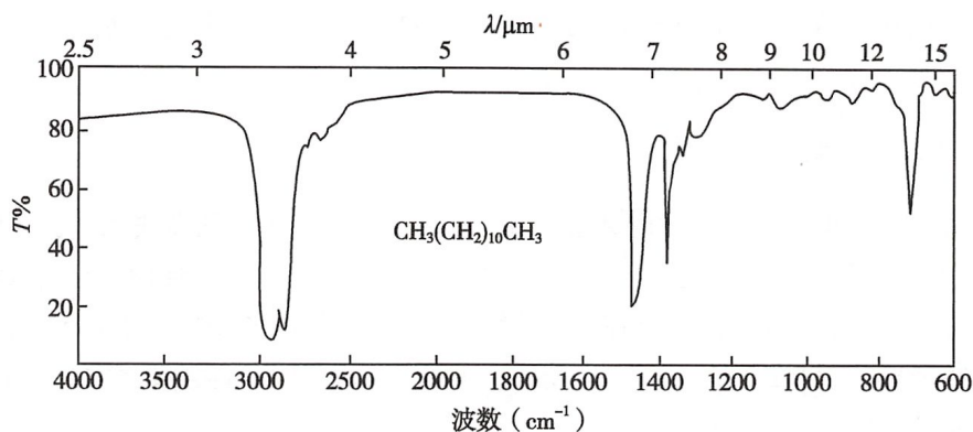
图 3-5 十二烷红外光谱
