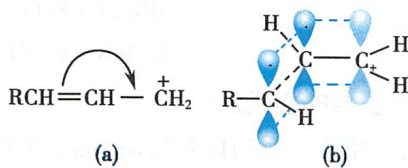
图 7-3 烯丙基正碳离子及其电子离域示意图
