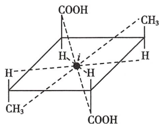
图2-5 对称中心
