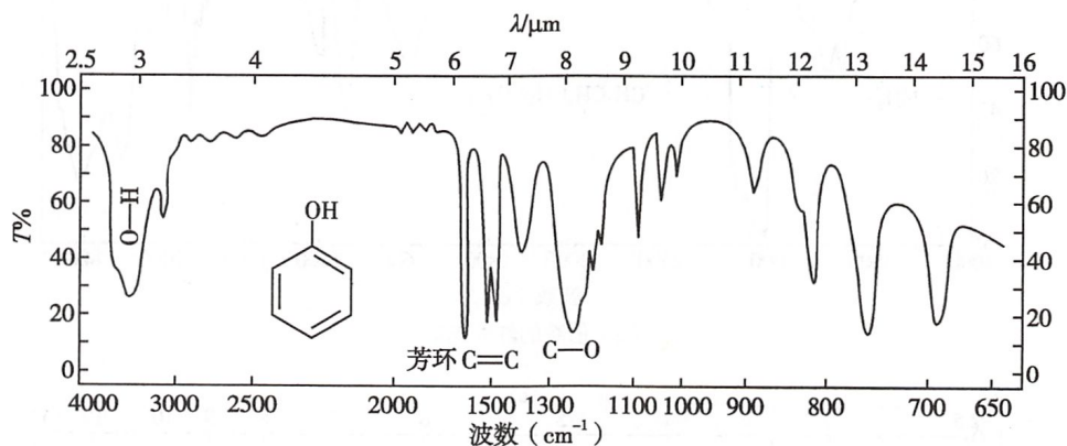
图 3-9 苯酚的红外光谱
