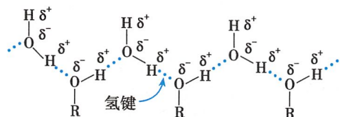
图 8-2 醇羟基与水之间形成的氢键
