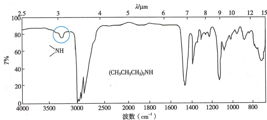
(b) 仲胺的红外光谱
