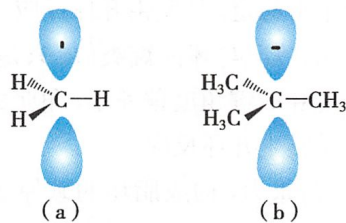
图 4-10 甲基自由基 (a) 及叔丁基自由基 (b) 的结构
