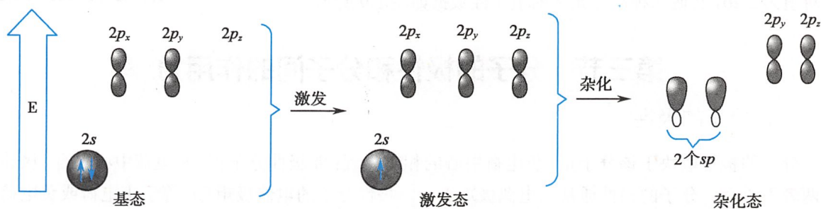
图1-7 碳的 sp 杂化过程
