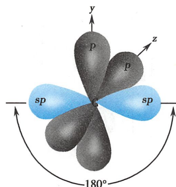
图 1-8 sp 杂化碳的构型
