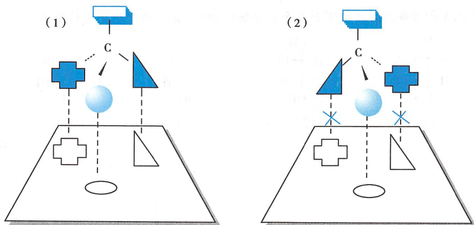
图 2-11 一对对映体与同一种受体之间的结合情况
