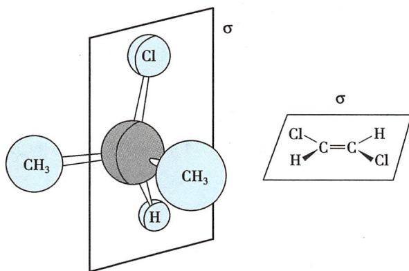
图2-4 2-氯丙烷和1,2-二氯乙烯的对称面
