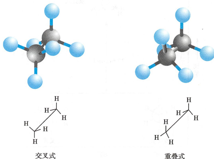
图 4-3 乙烷的锯架式结构图
