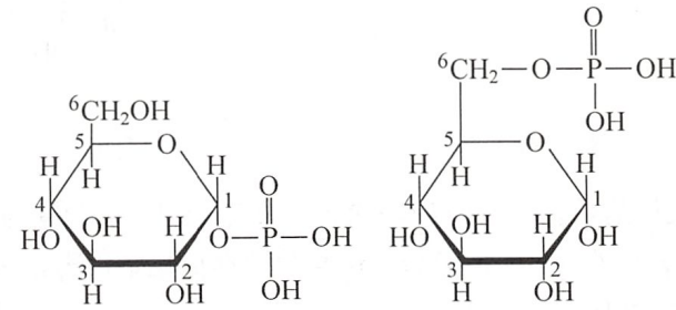
\alpha -1-磷酸吡喃葡萄糖
