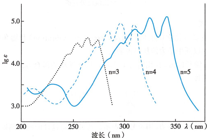
图 3-4 \text{H}-(\text{CH}=\text{CH})_n-\text{H} 的紫外光谱
