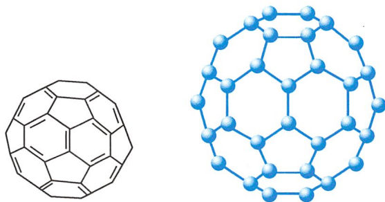
图 6-3 \text{C}_{60} 分子结构示意图
