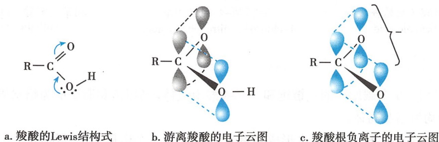
图 11-1 羧酸的结构
