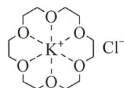
18-冠-6与KCl的络合物
