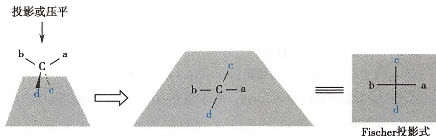
图 2-7 Fischer 投影式示意图
