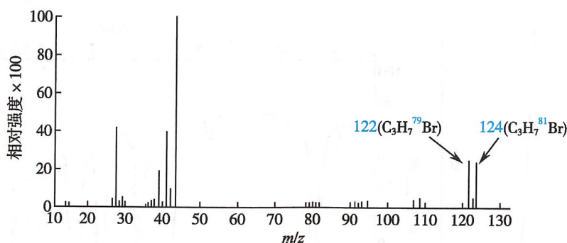
图 3-24 1-溴丙烷的质谱图
