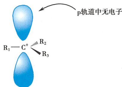
图5-2 正碳离子
