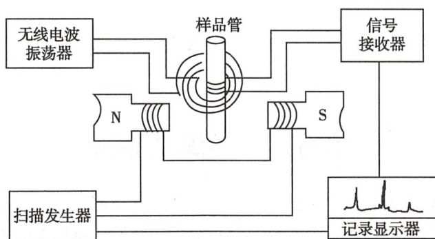
图 3-15 核磁共振仪示意图
