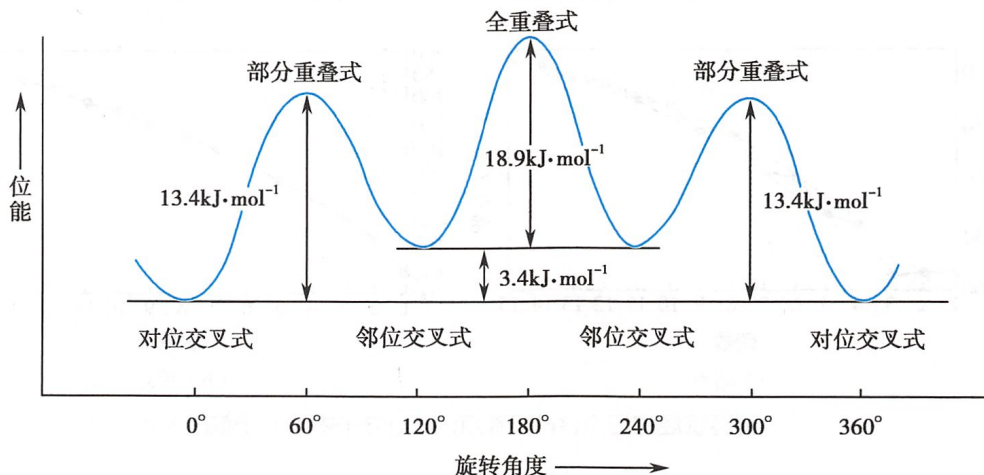
图 4-6 正丁烷 \text{C}_2-\text{C}_3 旋转时各种构象的能量曲线
