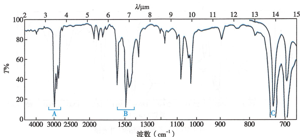
图 3-8 甲苯的红外光谱
