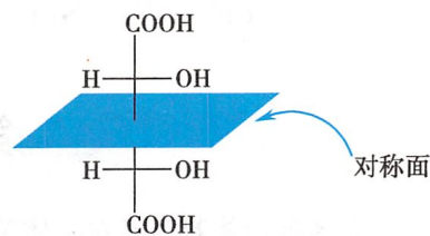
图 2-9 内消旋酒石酸
