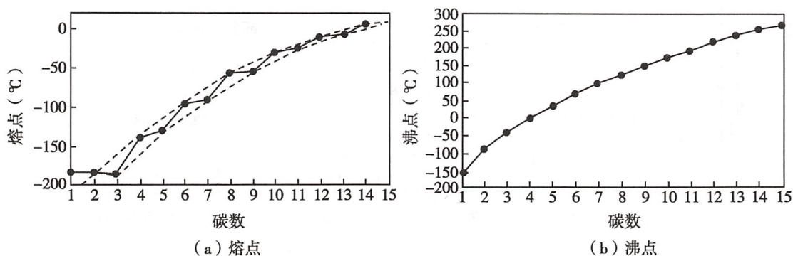
图 4-8 直链烷烃的熔点(a)和沸点(b)与分子中碳原子数的关系
