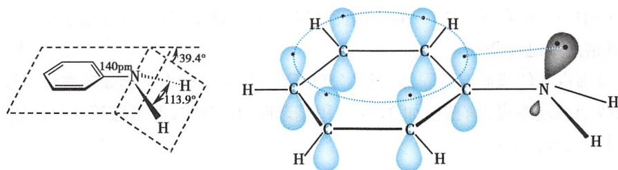
图 13-2 苯胺的结构
