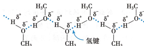
图 8-3 液态甲醇分子之间缔合的氢键
