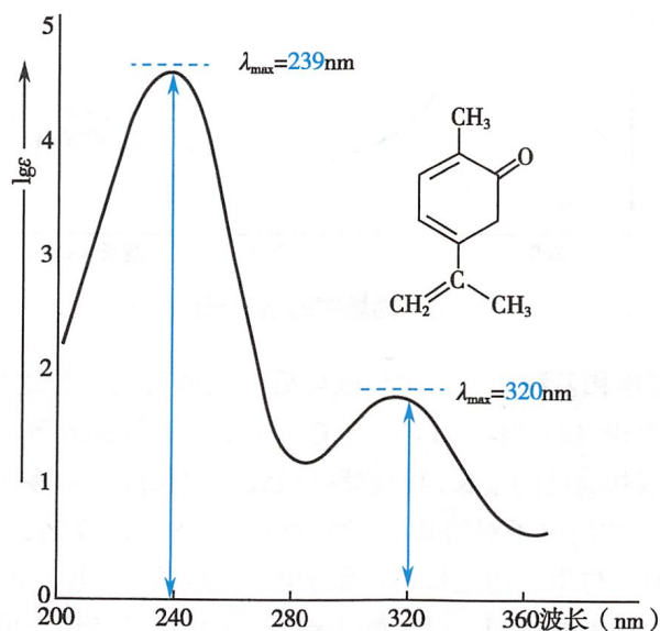
图 3-1 香芹酮的紫外光谱图
