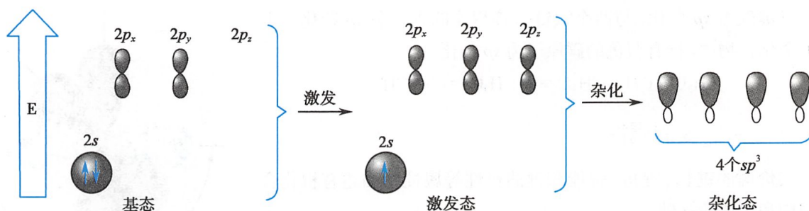
图1-4 碳的 sp^3 杂化过程
