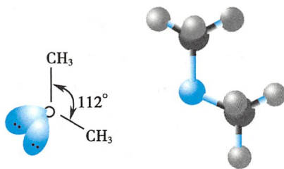
图 9-1 甲醚分子的结构
