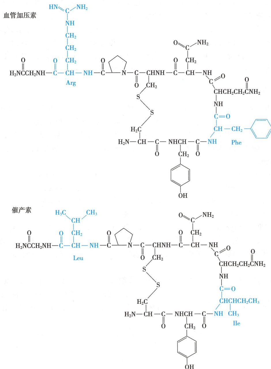
图 17-3 催产素和血管加压素的结构
