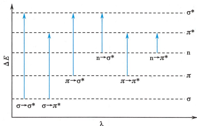
图 3-2 分子轨道能级及主要的电子跃迁类型
