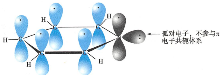
图 14-1 吡啶结构的电子云图
