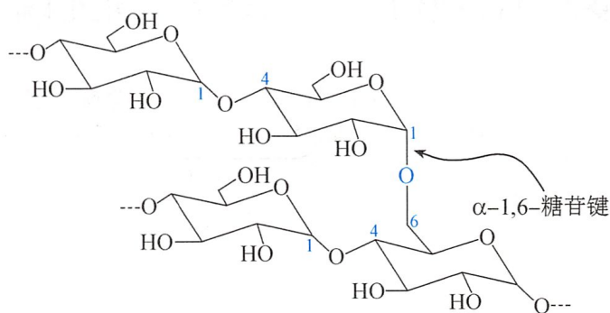
支链淀粉结构
