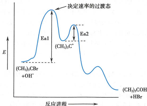
图 7-1 叔丁基溴水解反应( \text{S}_{\text{N}}1 )的能量曲线
