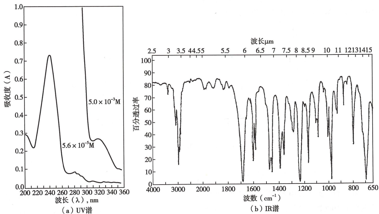
图 3-25 未知物的 UV、IR 和 ^1\text{H-NMR} 谱
