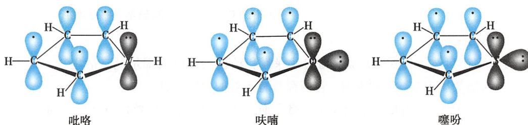
图 14-2 吡咯、呋喃和噻吩的结构
