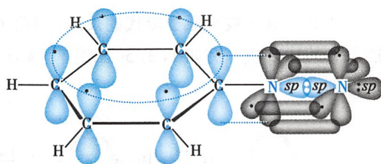
图 13-4 苯重氮正离子的结构
