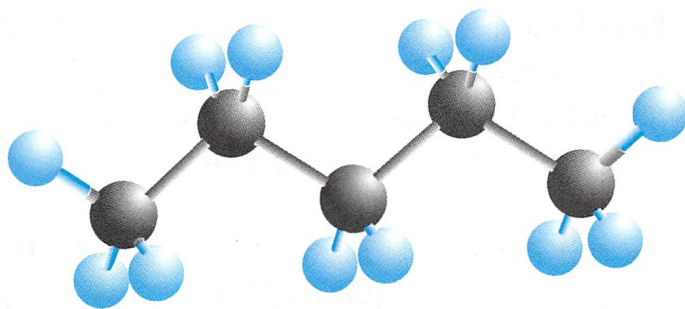
图 4-7 戊烷分子结构球棍模型
