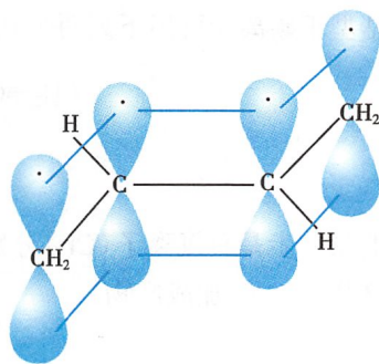
图 5-3 1, 3-丁二烯分子的大 \pi 键示意图
