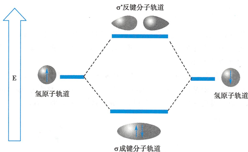
图 1-10 氢的原子轨道和分子轨道
