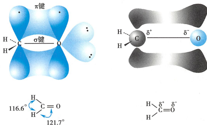
图 10-1 甲醛的结构
