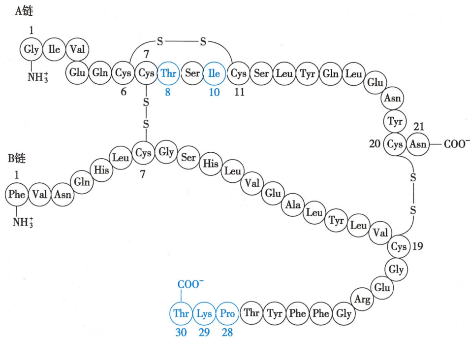
图 17-4 人胰岛素分子的一级结构
