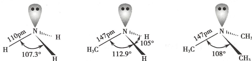
图 13-1 氨、甲胺和三甲胺的结构
