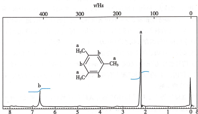
图 3-19 均三甲苯的 ^1\text{H-NMR} 谱
