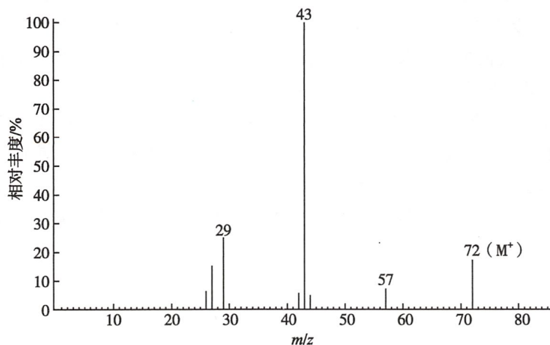
图 3-23 丁酮的质谱图
