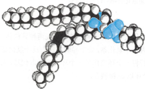
图 15-1 甘油磷脂的分子模型
