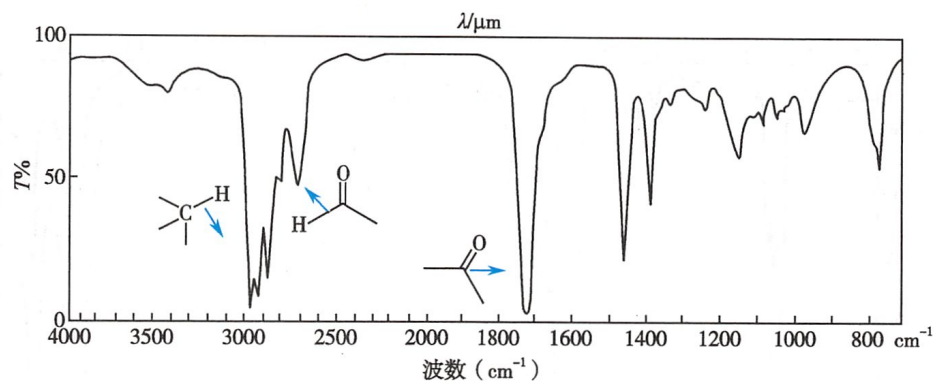
图 3-10 2-乙基丁醛的红外光谱
