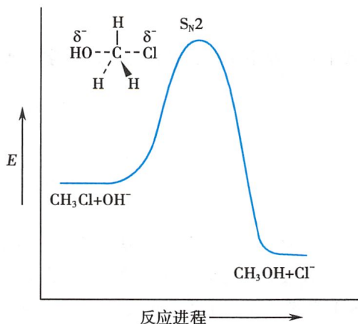
图 7-2 氯甲烷水解反应 ( S_N2 ) 的能量曲线
