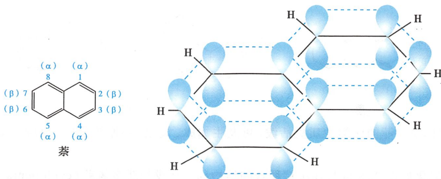
图 6-2 萘的 p 轨道组成的大 \pi 键
