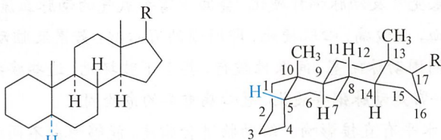
5 \beta -系甾族化合物
