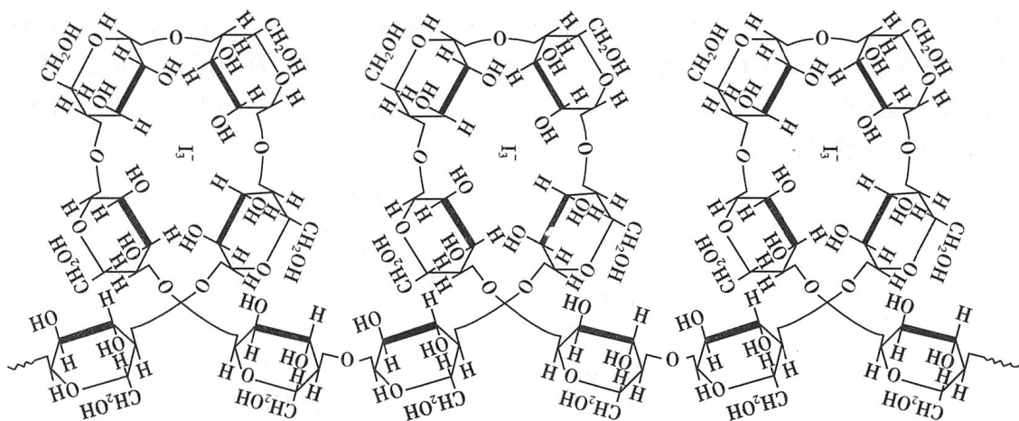
图 16-2 淀粉分子与碘作用示意图
