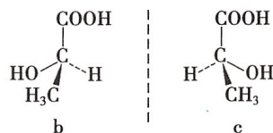
图 2-2 乳酸分子的两种立体结构
