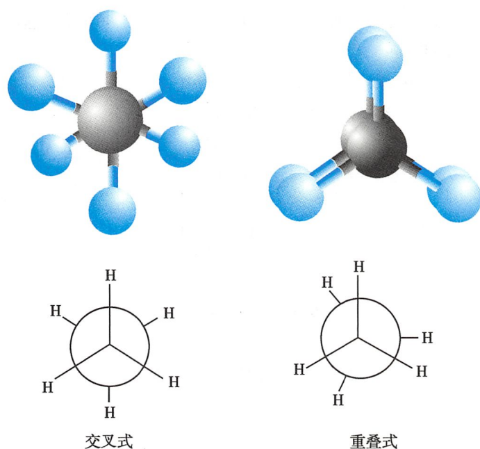
图 4-4 乙烷的纽曼投影式
