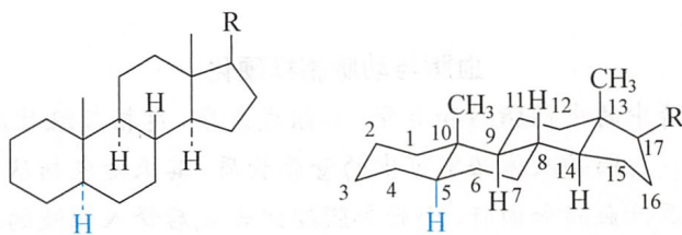
5 \alpha -系甾族化合物
