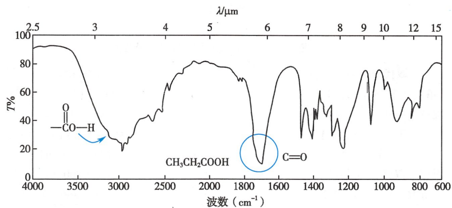
图 3-11 丙酸的红外光谱
