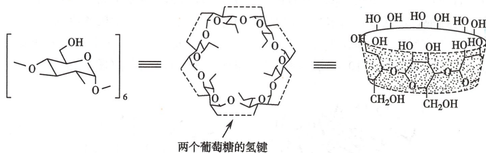
图 16-4 \alpha -环糊精
