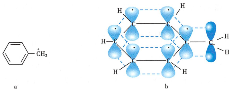
图 7-4 苄基正碳离子及其电子离域示意图
