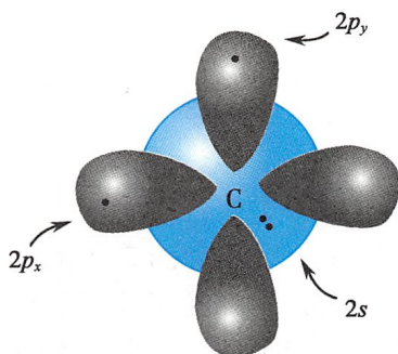
图1-2 基态碳原子的外层电子构型
