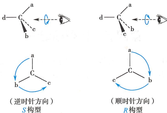
图 2-8 R/S 标记方法示意图
