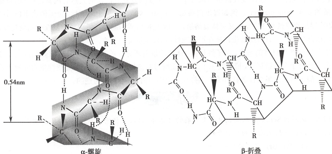
图17-5 蛋白质二级结构片段
