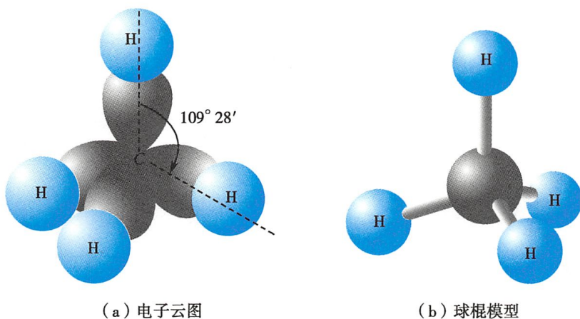
图 4-1 甲烷分子的结构
