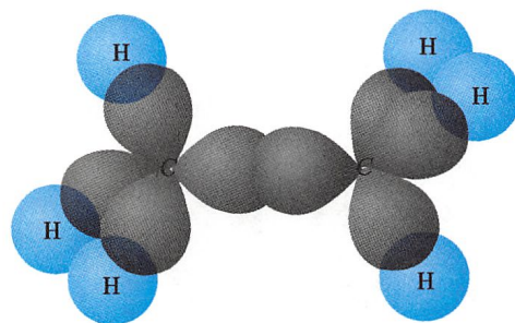
图 4-2 乙烷分子的电子云图
