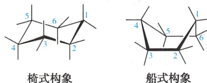
图 4-12 环己烷的两种典型构象
