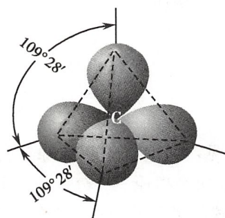
图1-3 sp^3 杂化碳的构型
