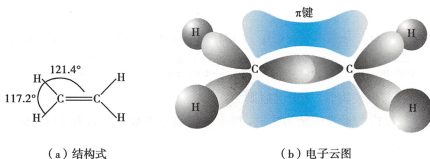
图 5-1 乙烯分子的结构示意图
