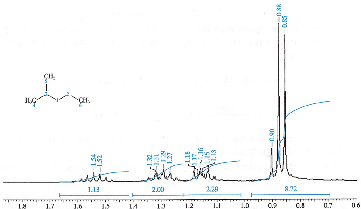
图 4-9 2-甲基戊烷核磁共振图谱
