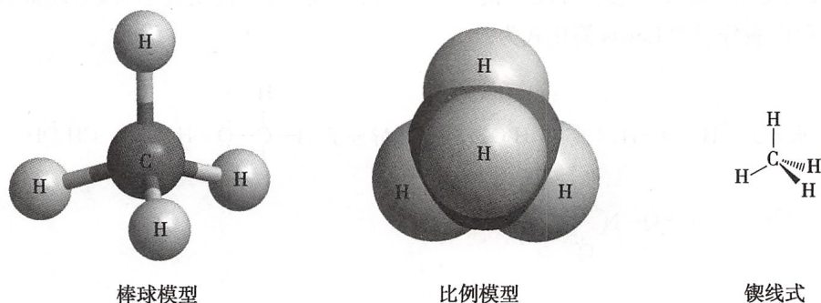
图 1-1 甲烷分子的模型和楔线式
