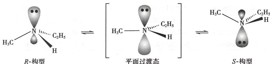
图 13-3 甲乙胺的一对对映体及其通过过渡态相互转化
