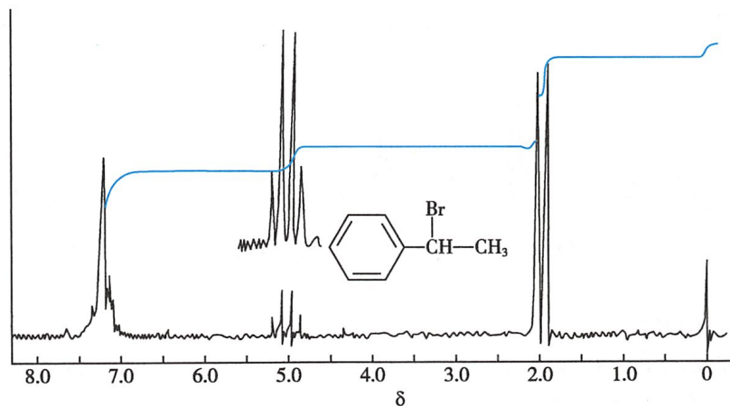
图3-21 C_8H_9Br 的 ^1H -NMR谱
