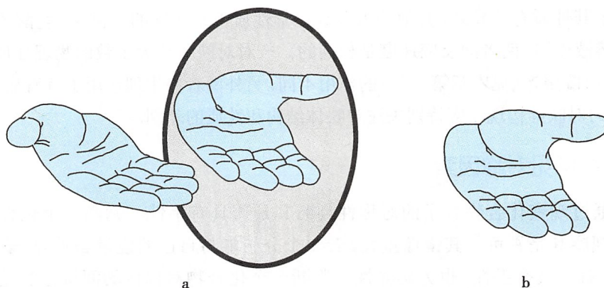
图 2-1 左右手及手性关系
