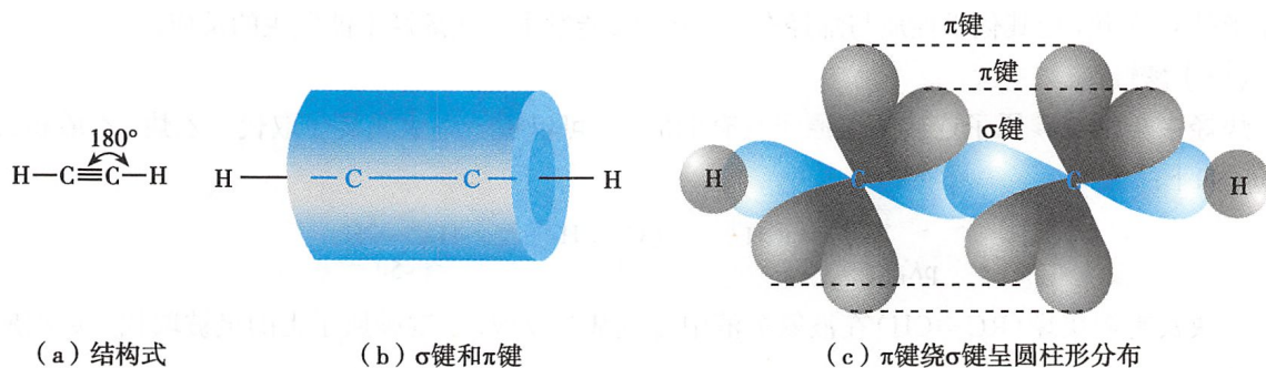
图 5-4 乙炔的结构
