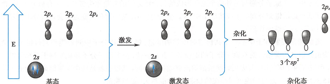
图1-5 碳的 sp^2 杂化过程
