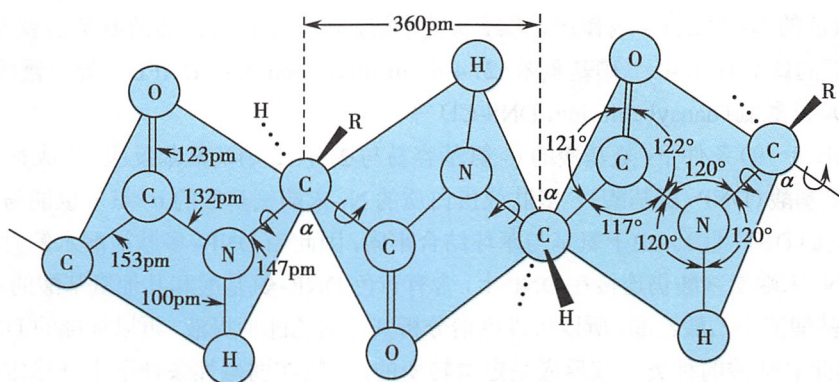
图 17-1 肽键平面
