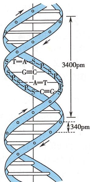
图18-1 DNA的双螺旋结构
