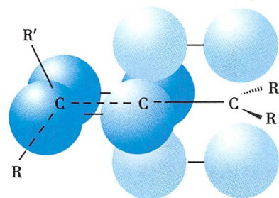
图 2-10 丙二烯型化合物的电子云图
