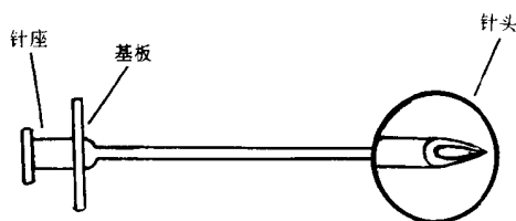
图 4-79 股静脉穿刺针
