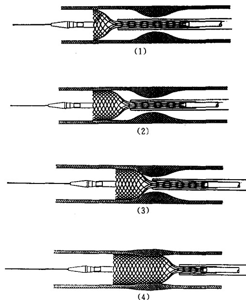
图 7-30 Wallstent 手术操作步骤
