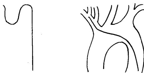
图 4-82 Headhunter 导管，用于锁骨下动脉、颈动脉、椎动脉造影
