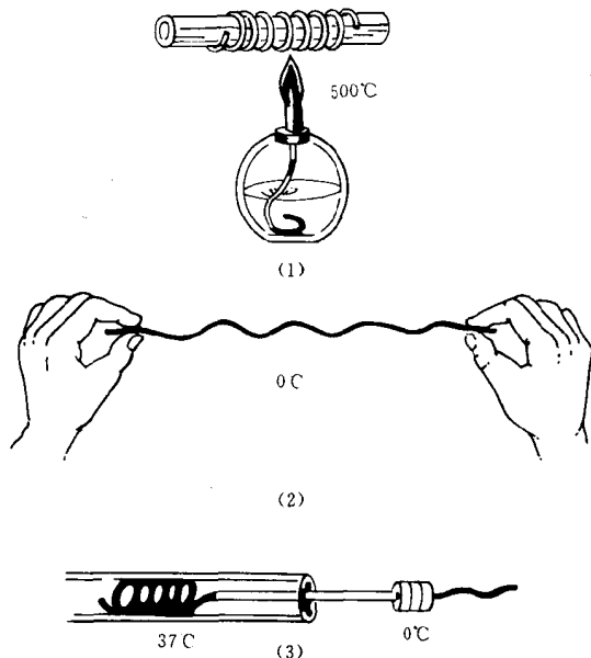
图 7-24 形状记忆合金内支架
