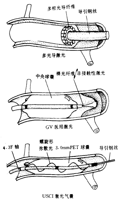
图 7-22 不同类型激光导管示意图
