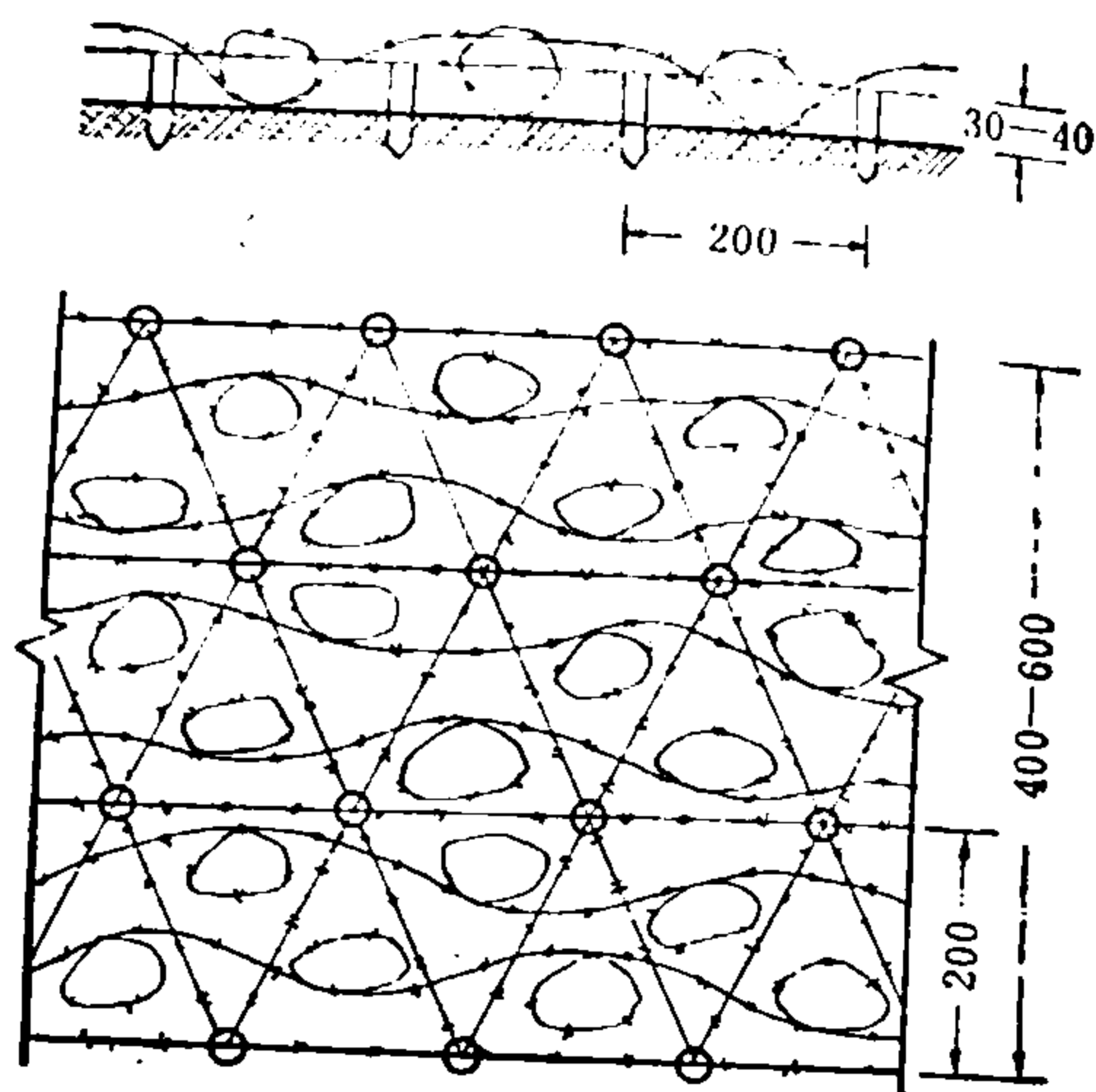
图34 低桩铁丝网（单位为厘米）
