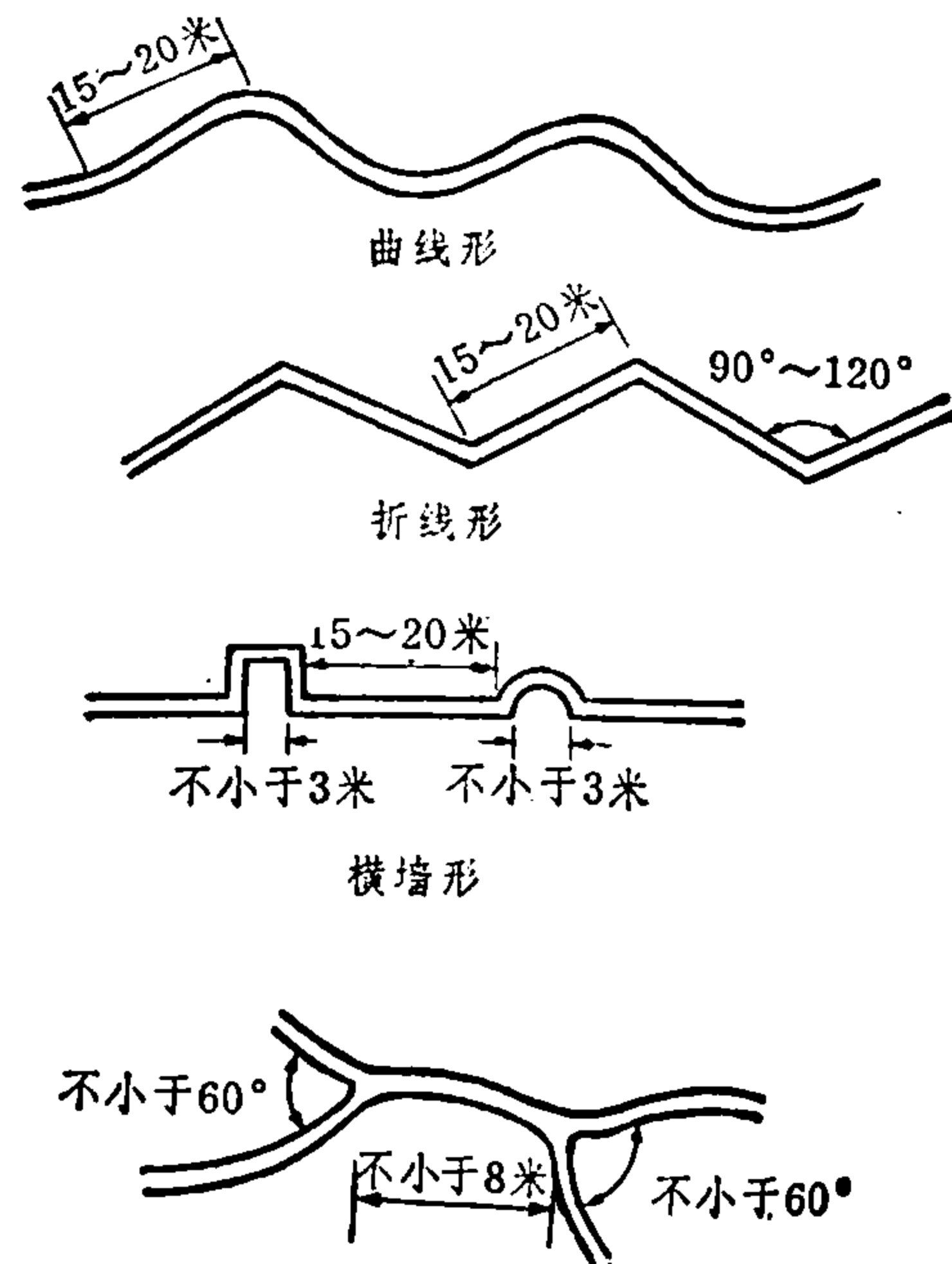
图22 堑壕、交通壕的形状
