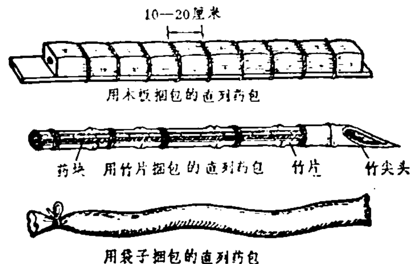
图7 直列药包
