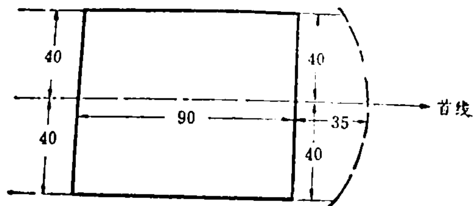
图15 立（跪）射单人掩体经始图 (单位为厘米)
