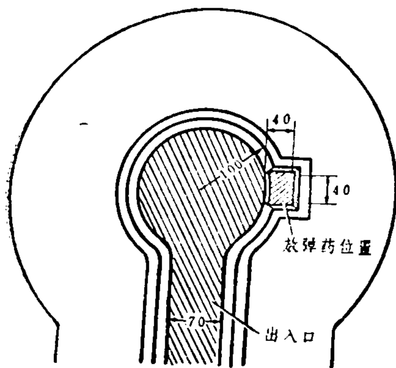
平面图
