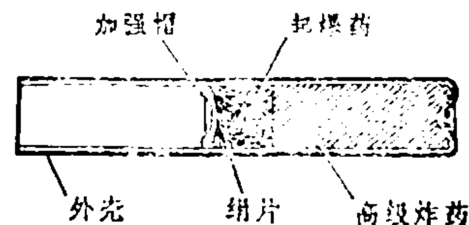
图2 雷管（火雷管）
