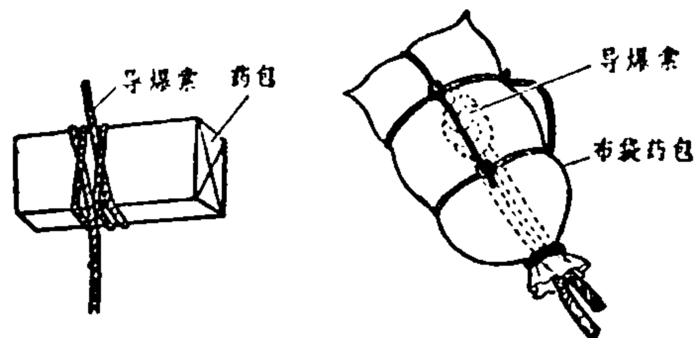
图16 导爆索与药包的连结
