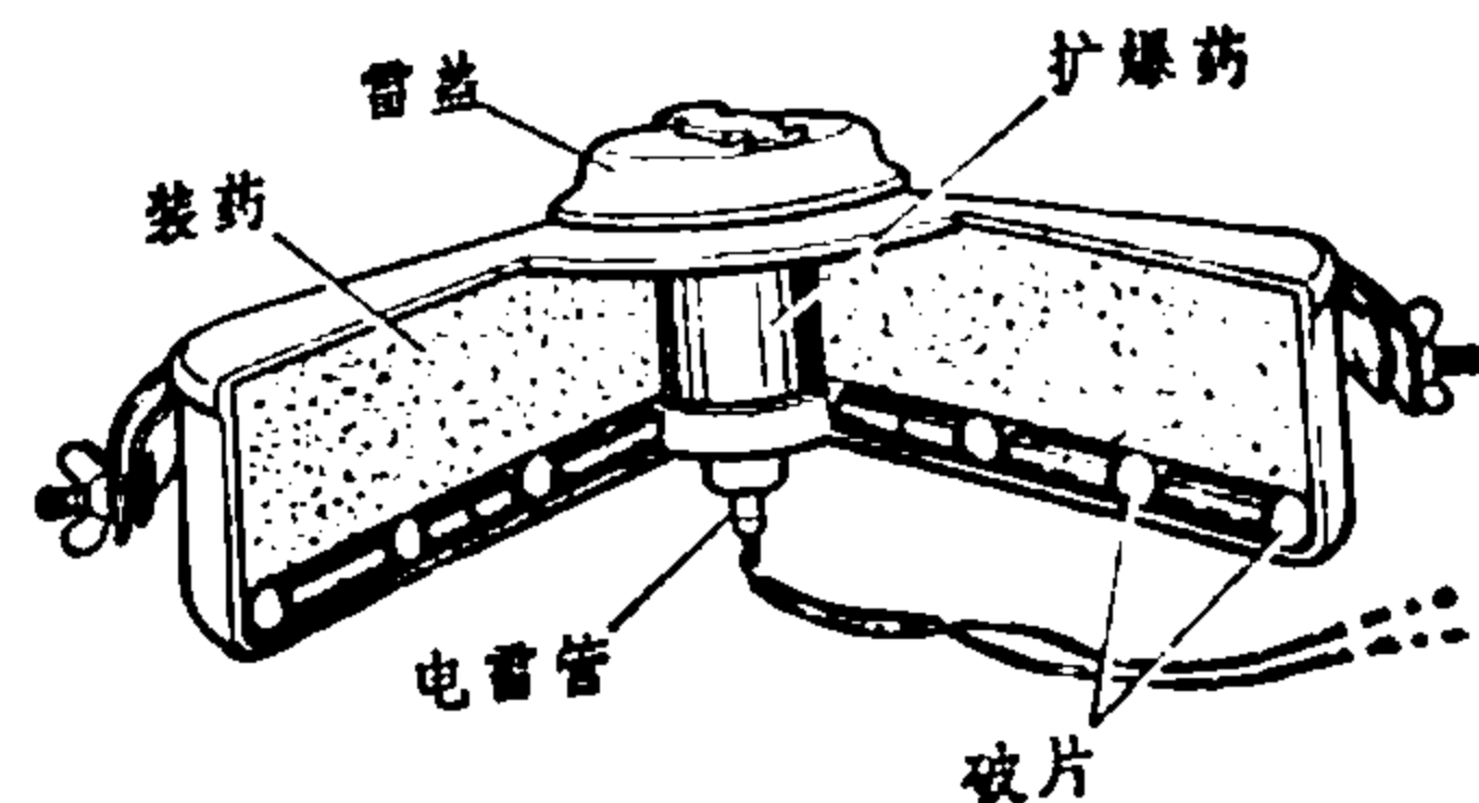
断面图
