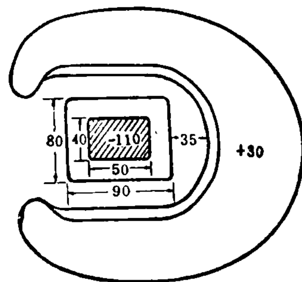
平面图
