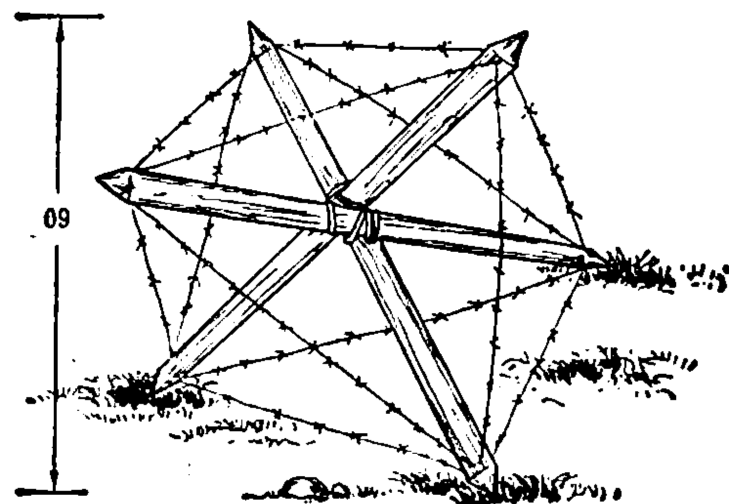
图36 菱形拒马
