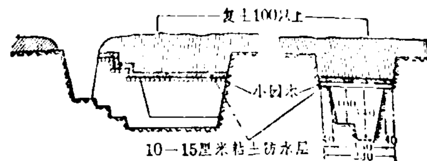
横断面图
