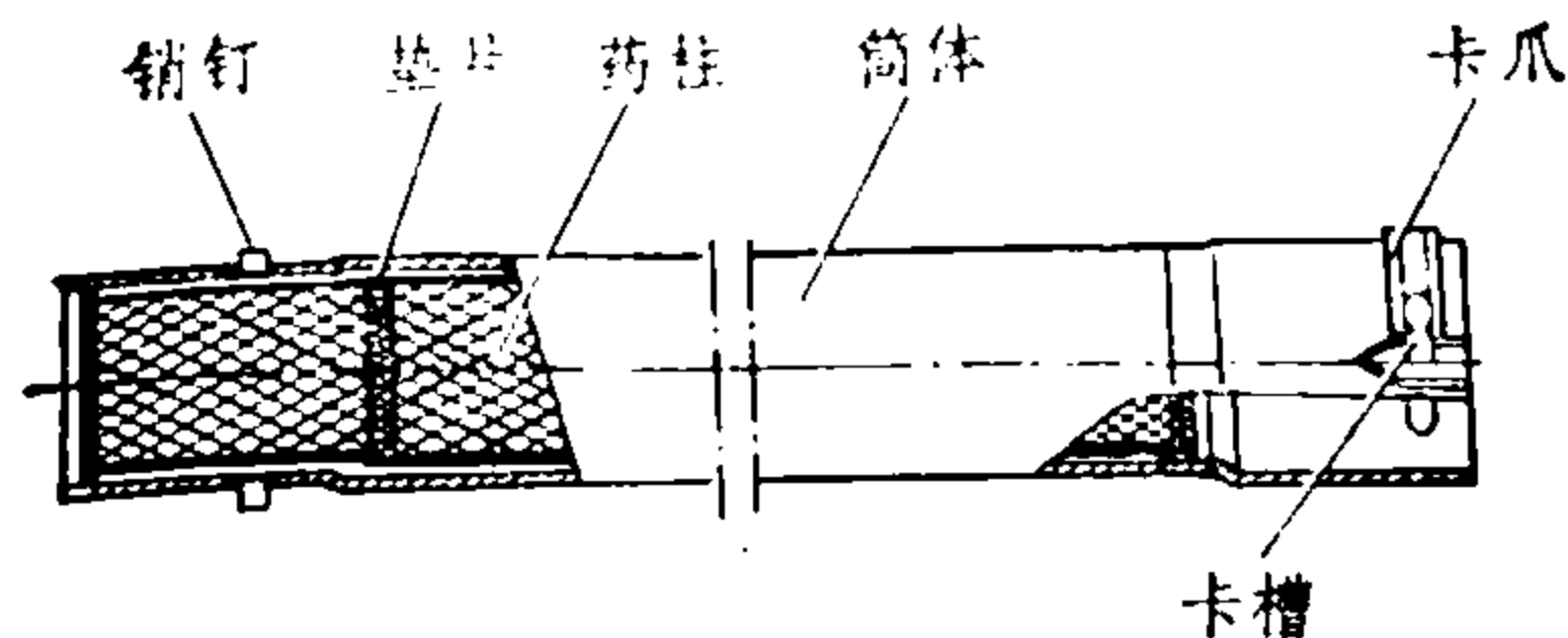
图18 筒身
