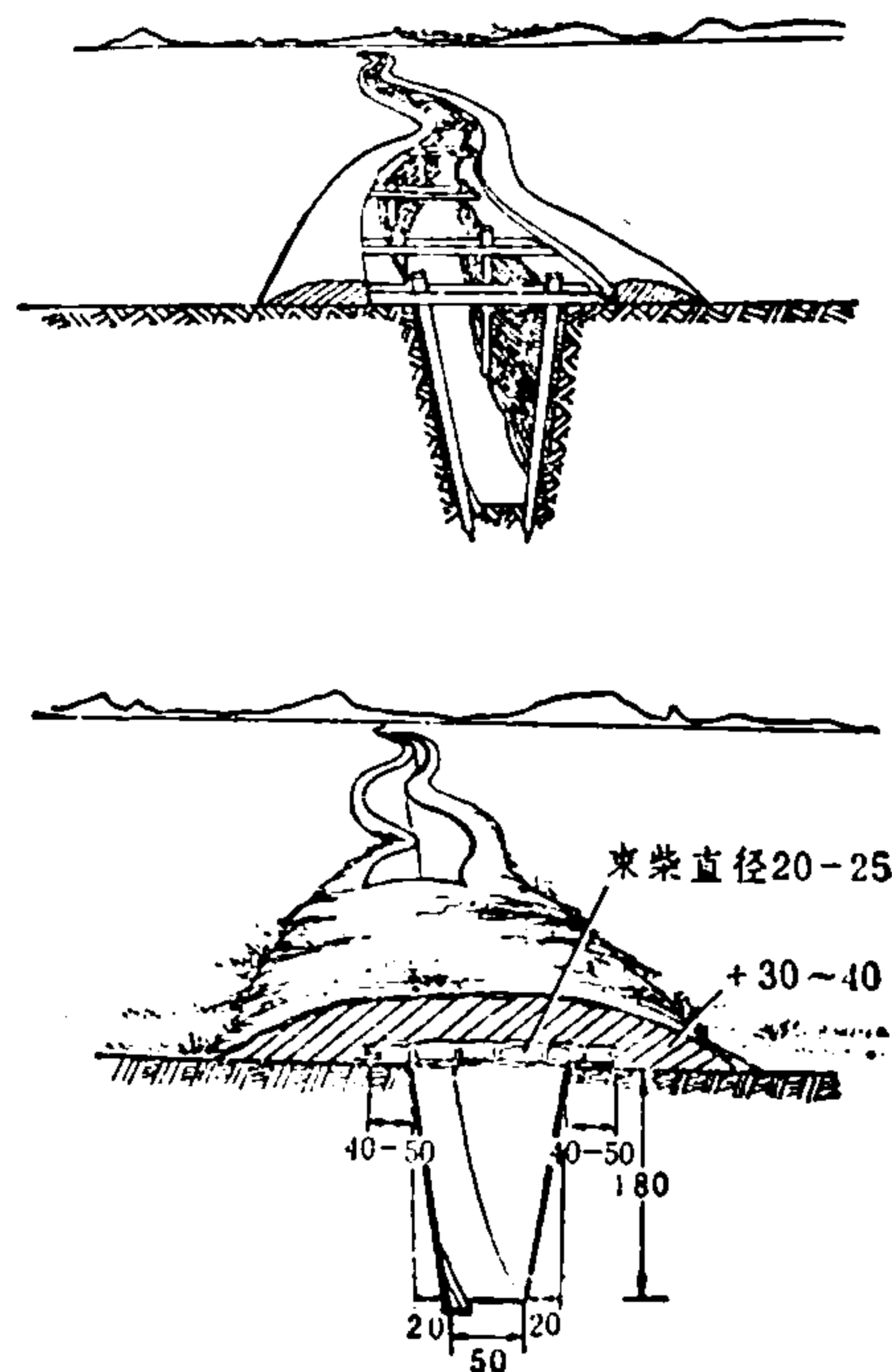
图 23 被复掩盖的堑壕、交通壕
