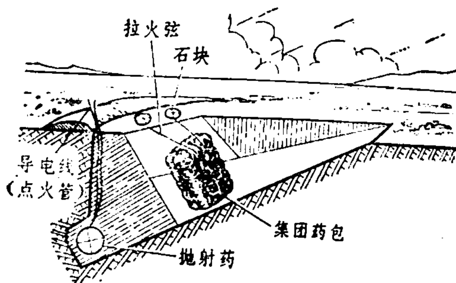
图30 药包设置好的情形
