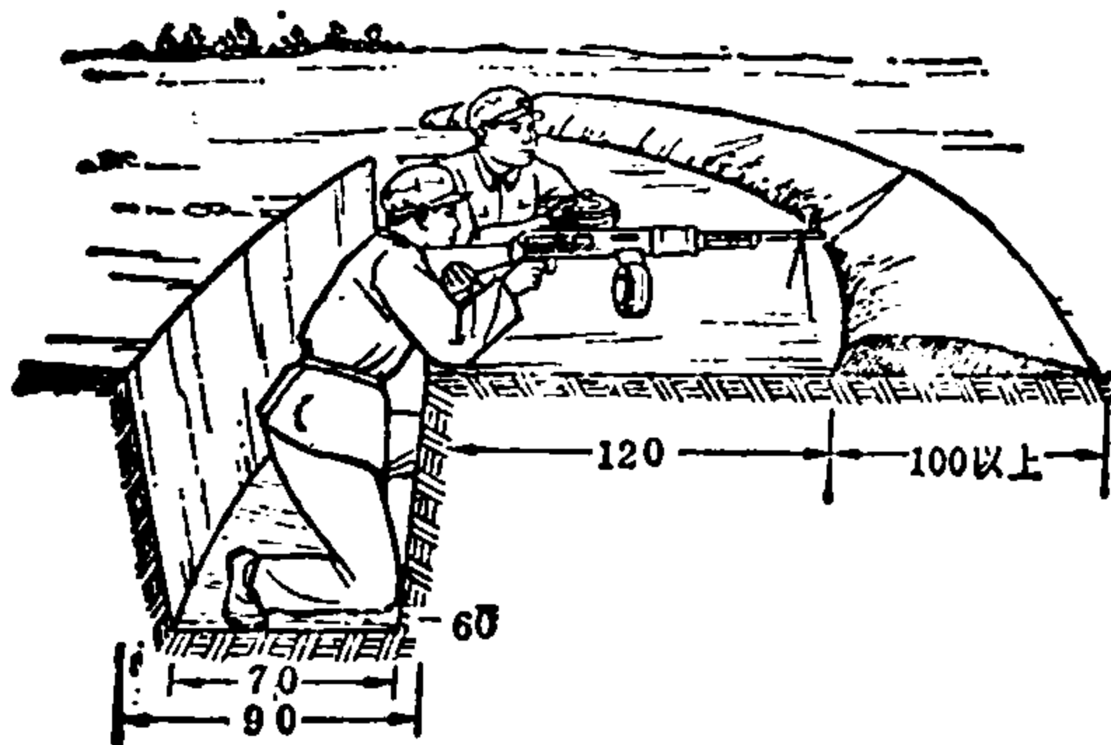
断面图
