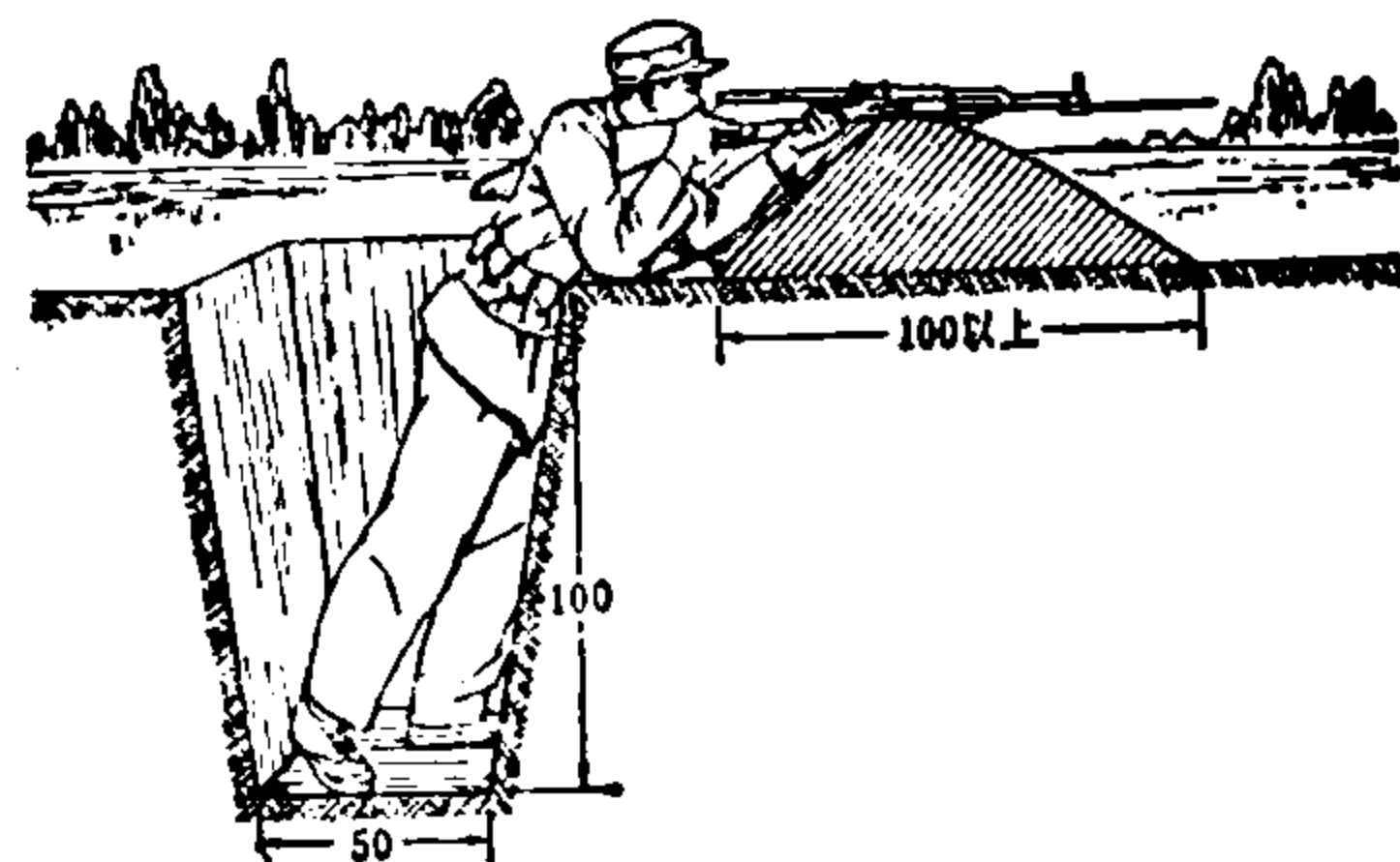
断面图
