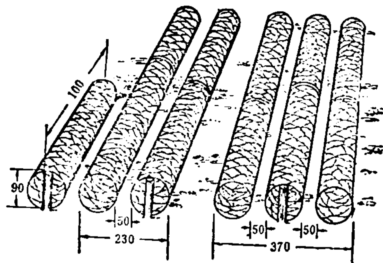
图31 蛇腹形铁丝网的设置(单位为厘米)
