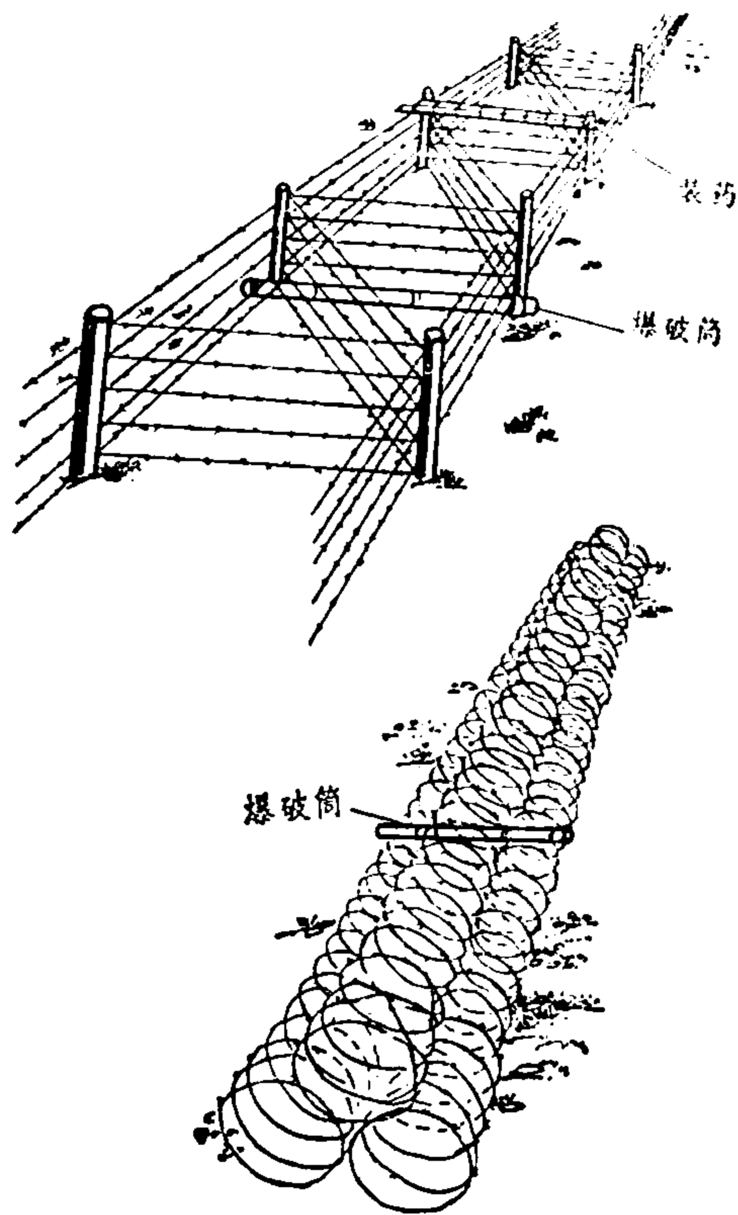
图23 对铁丝网的爆破
