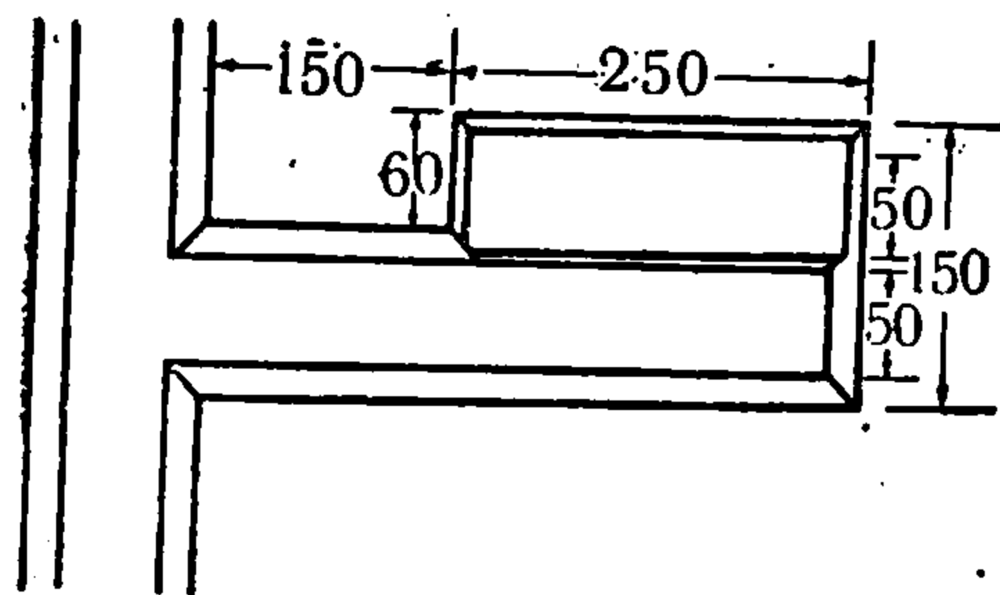
平面图
