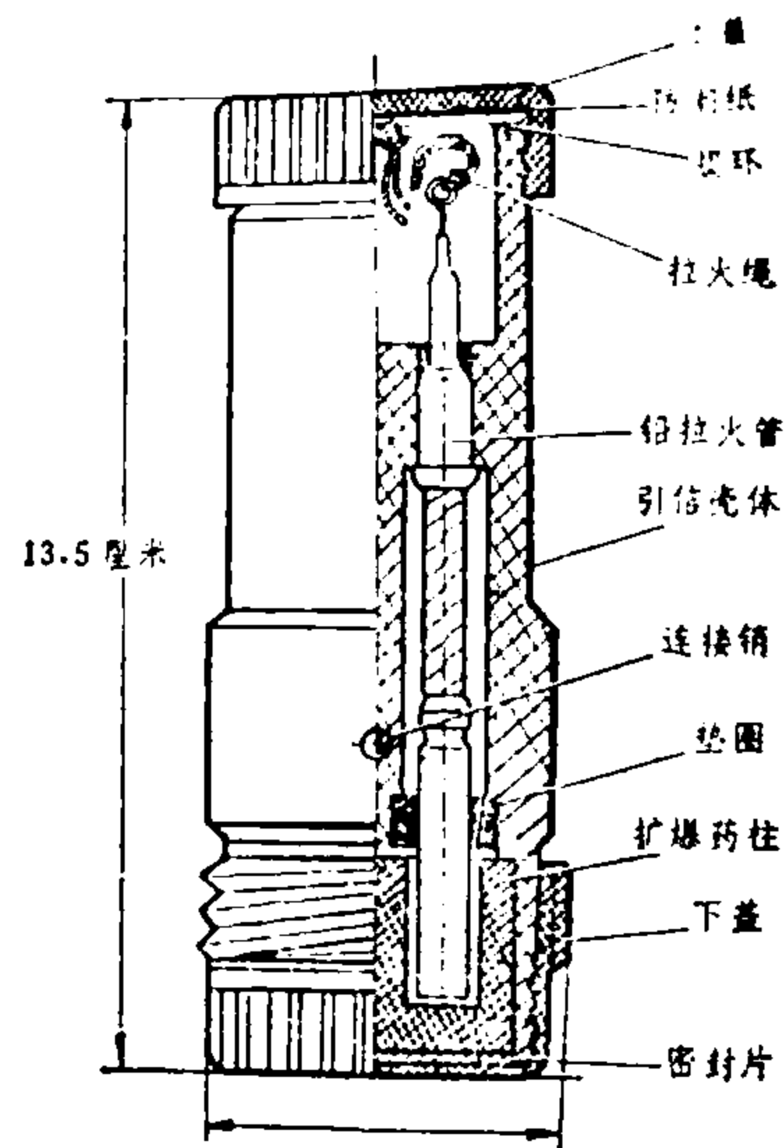
图20 六八一2式引信
