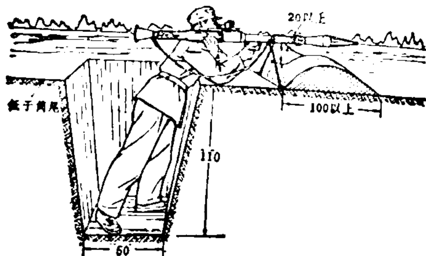
断面图
