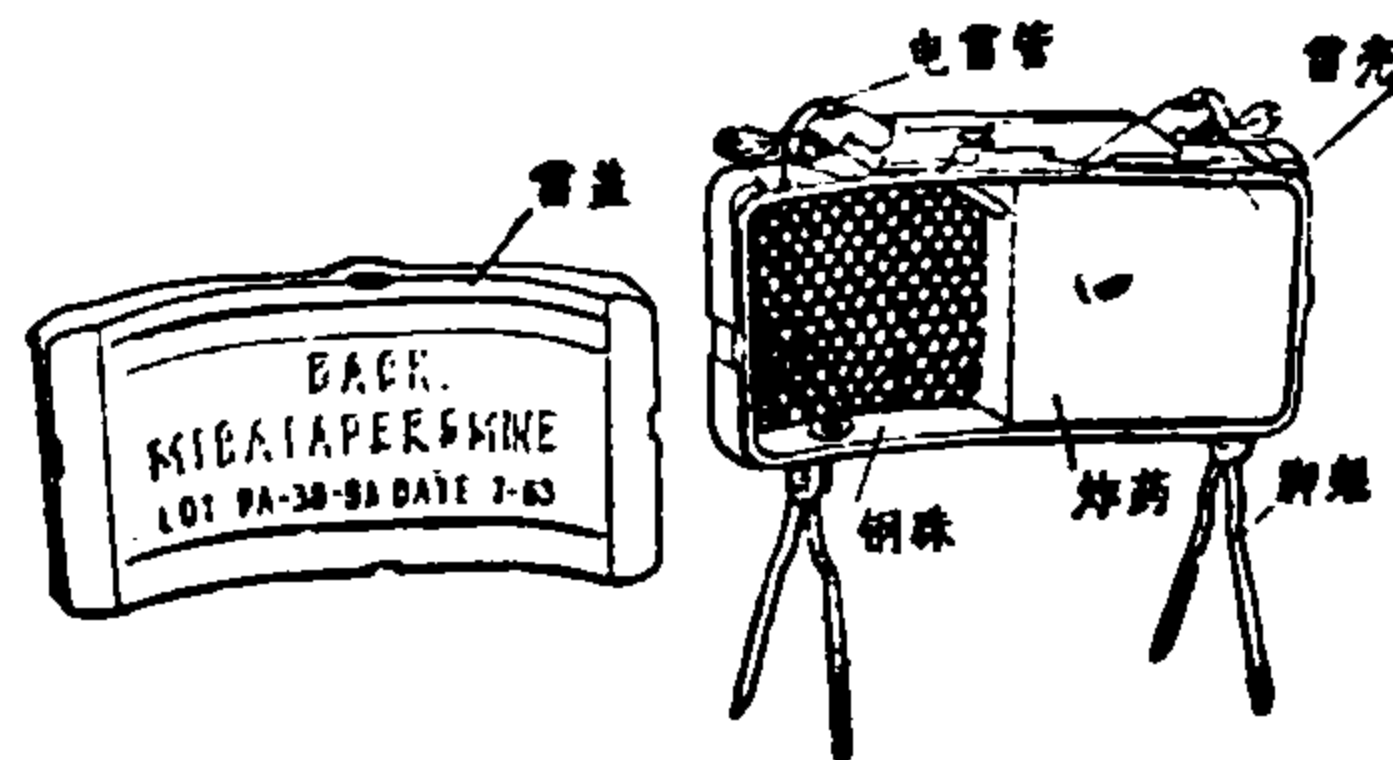
结构图
