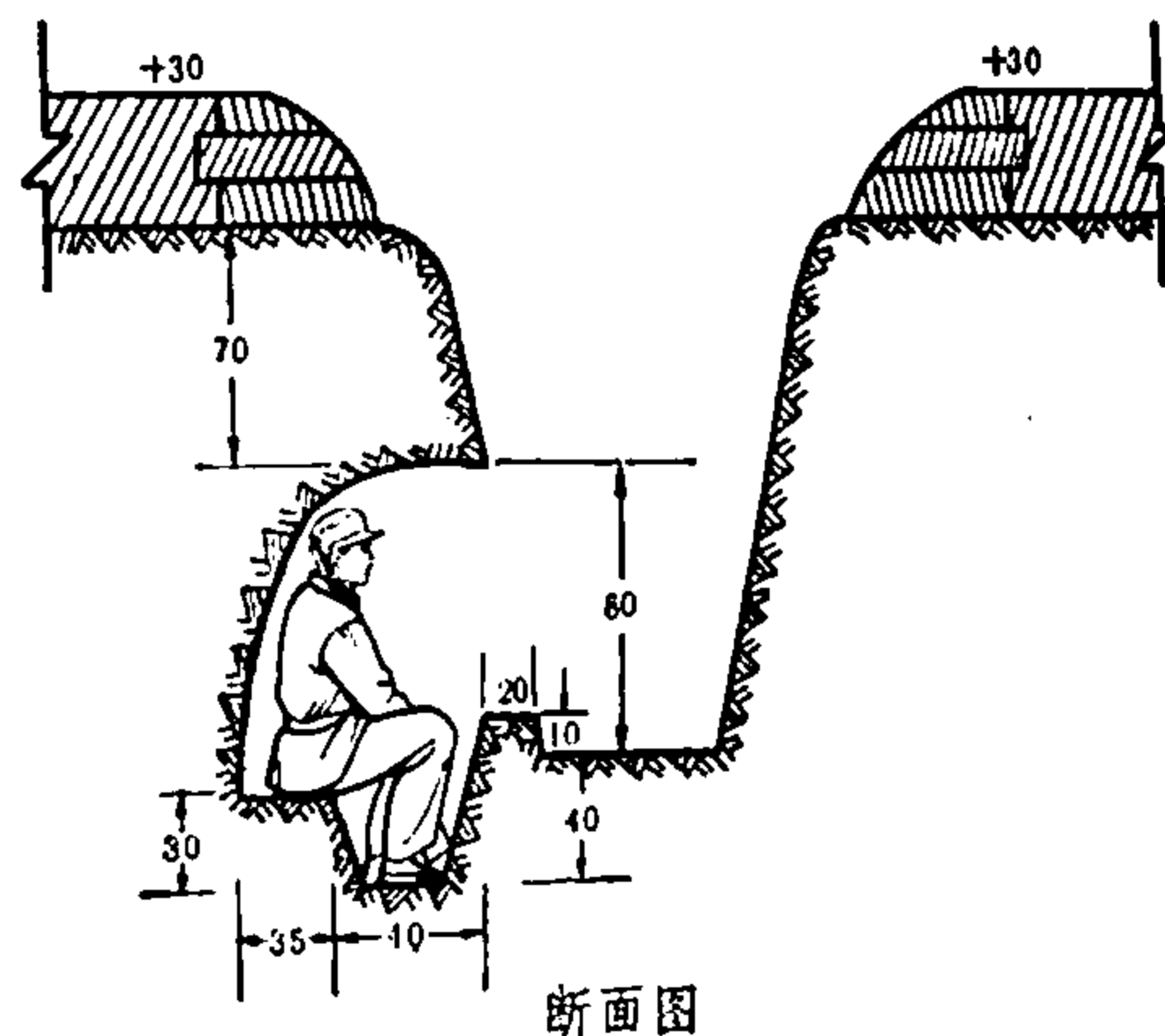
图24 崖孔(单位为厘米)
