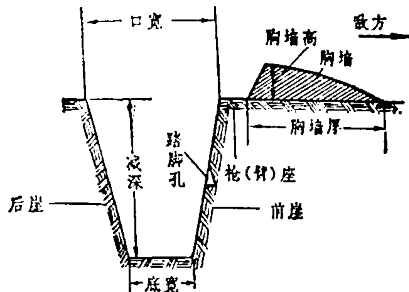
图 1 掩体的各部名称
