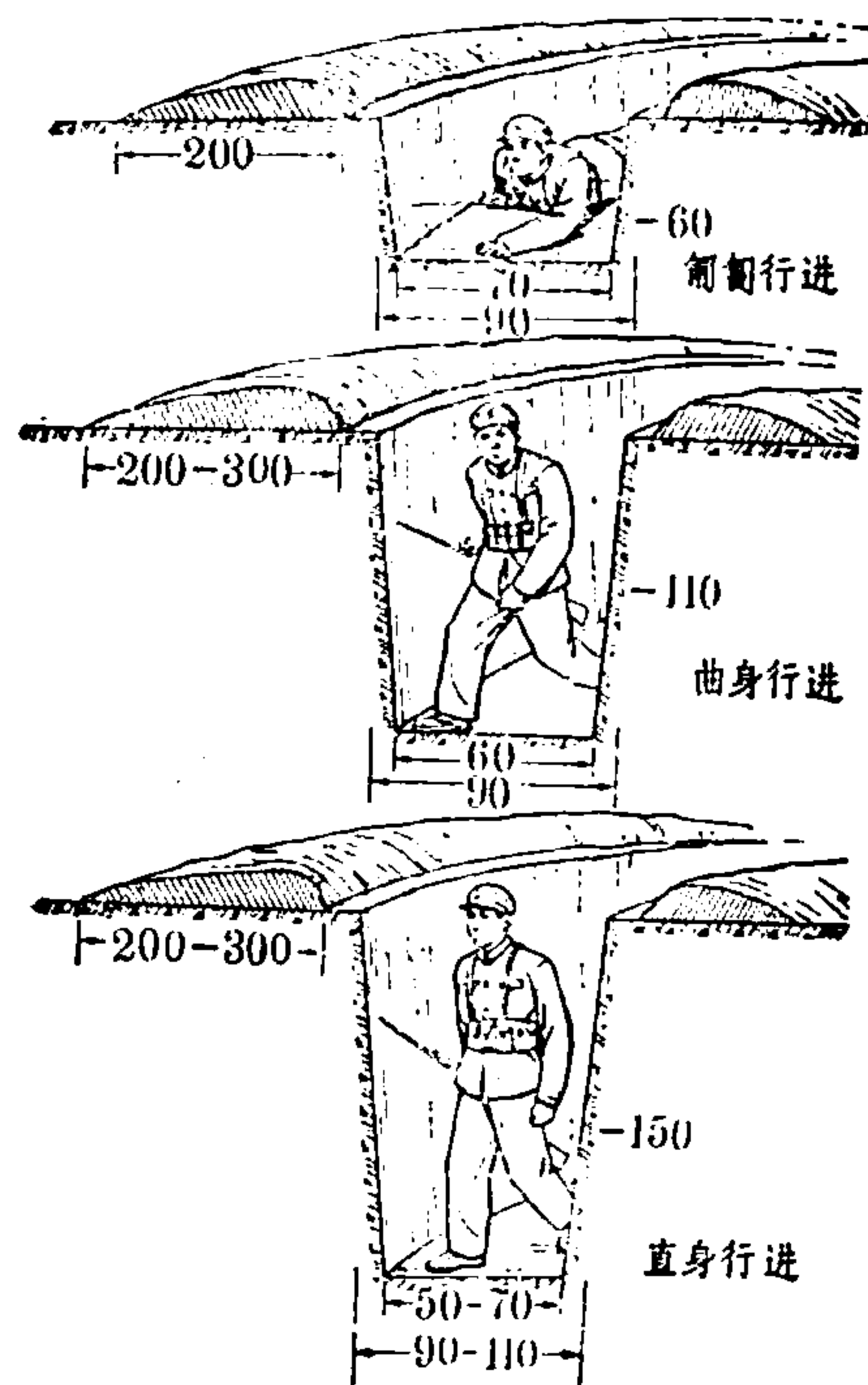
图21 堑壕交通壕的种类
