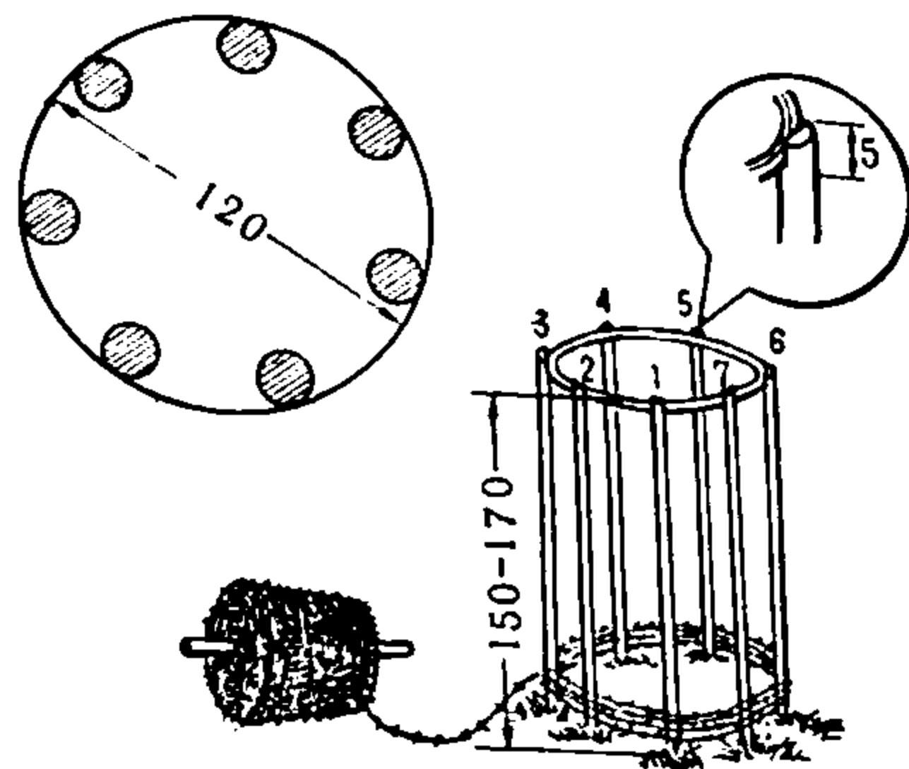
图30 蛇腹形铁丝网的制作
