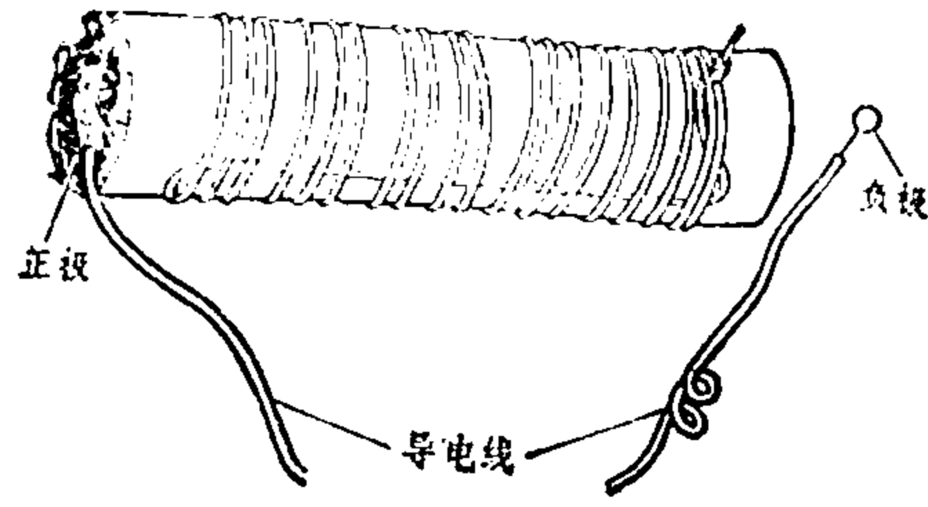
图17 干电池点火法
