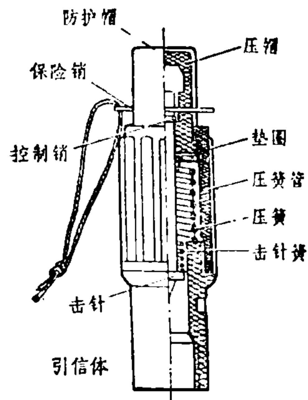
图32 六九式压、拉两用引信
