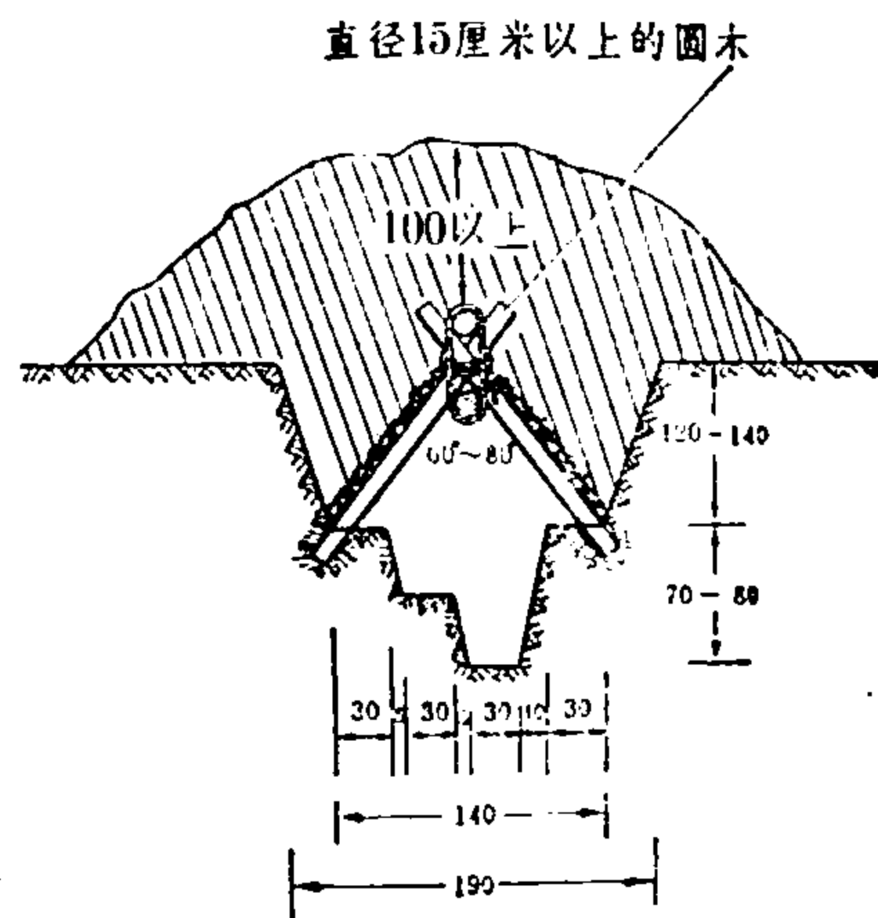
横断面图
