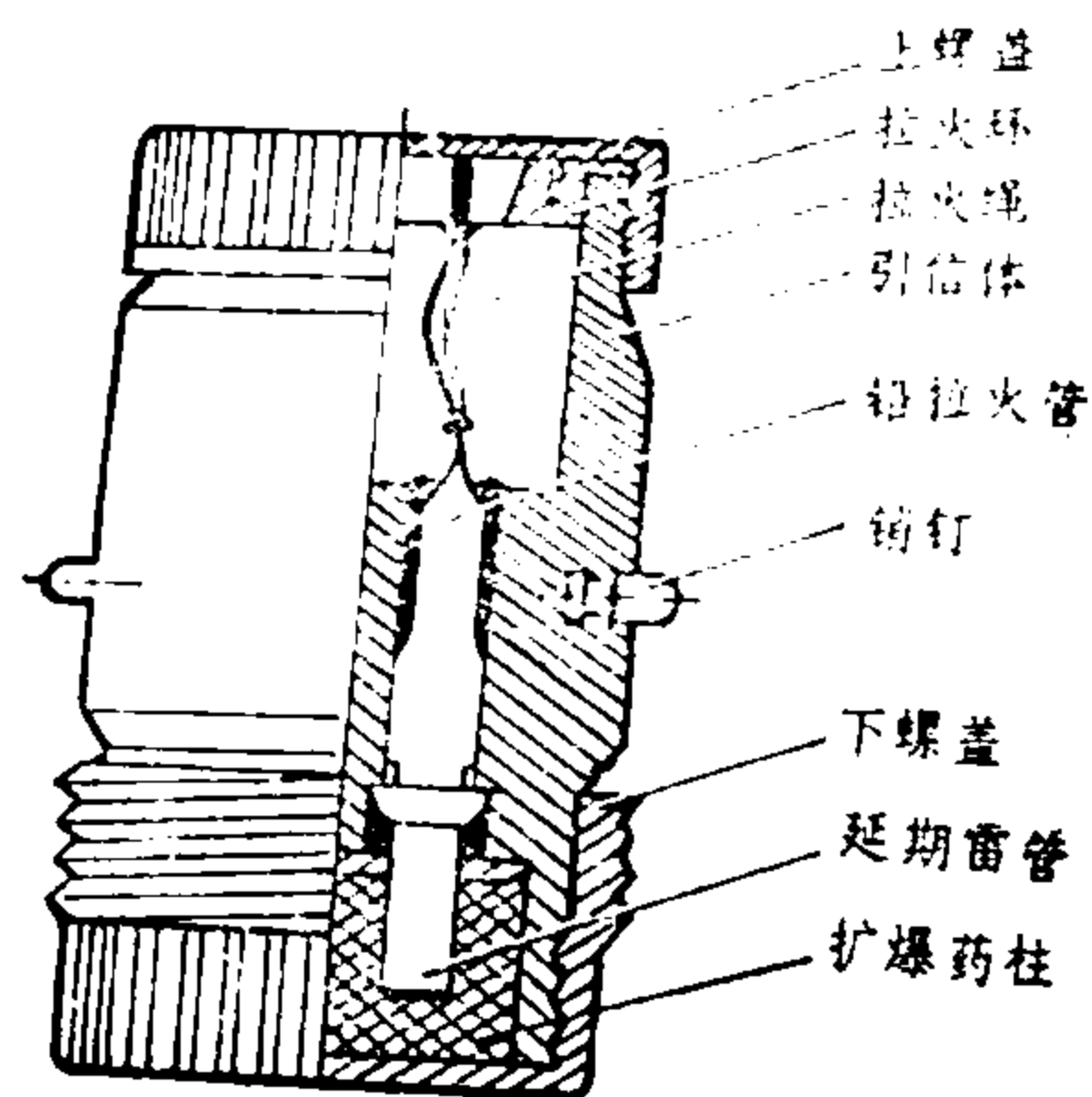
图19 六八一1式引信
