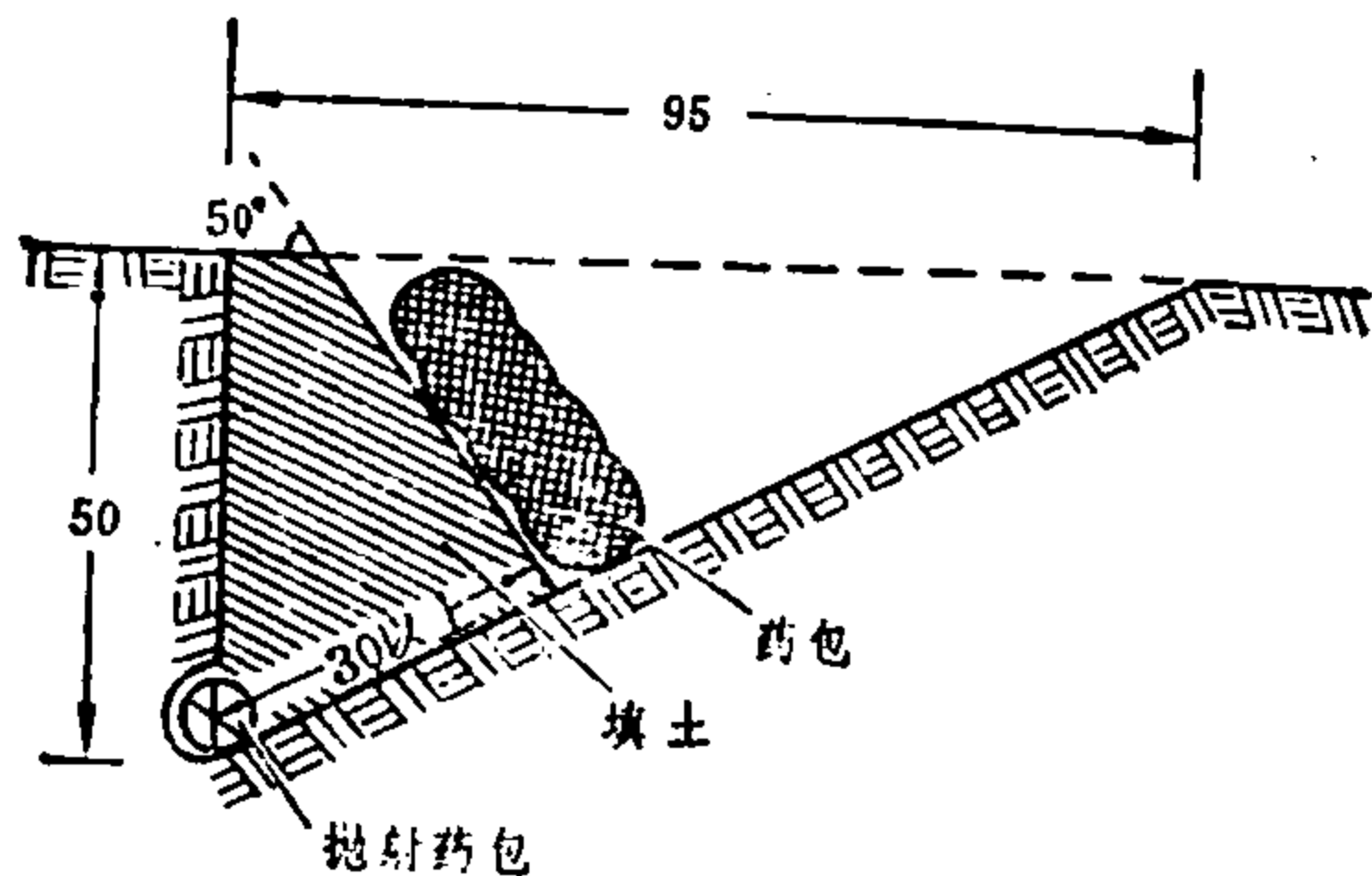
断面图
