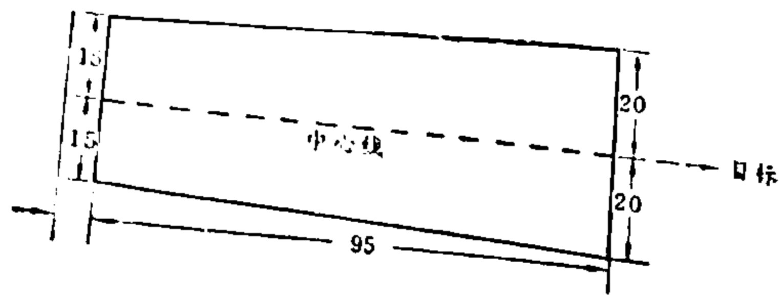
经始图
