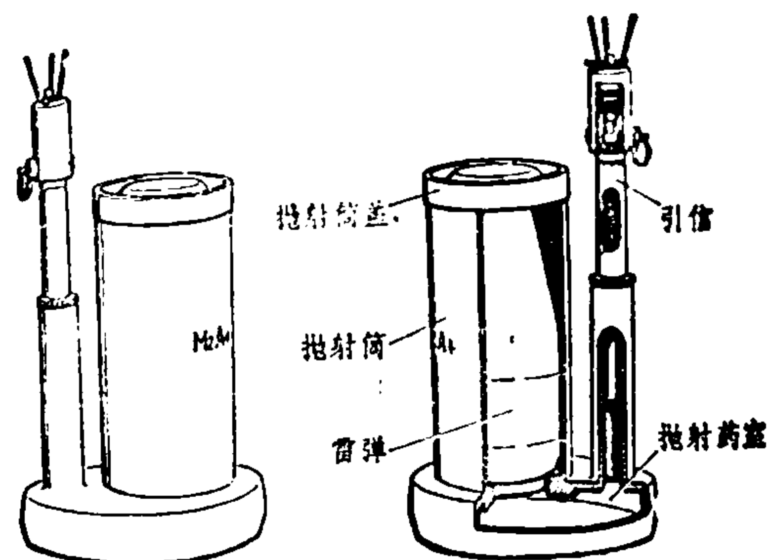
断面图
