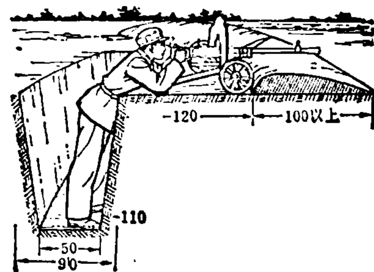
断面图
