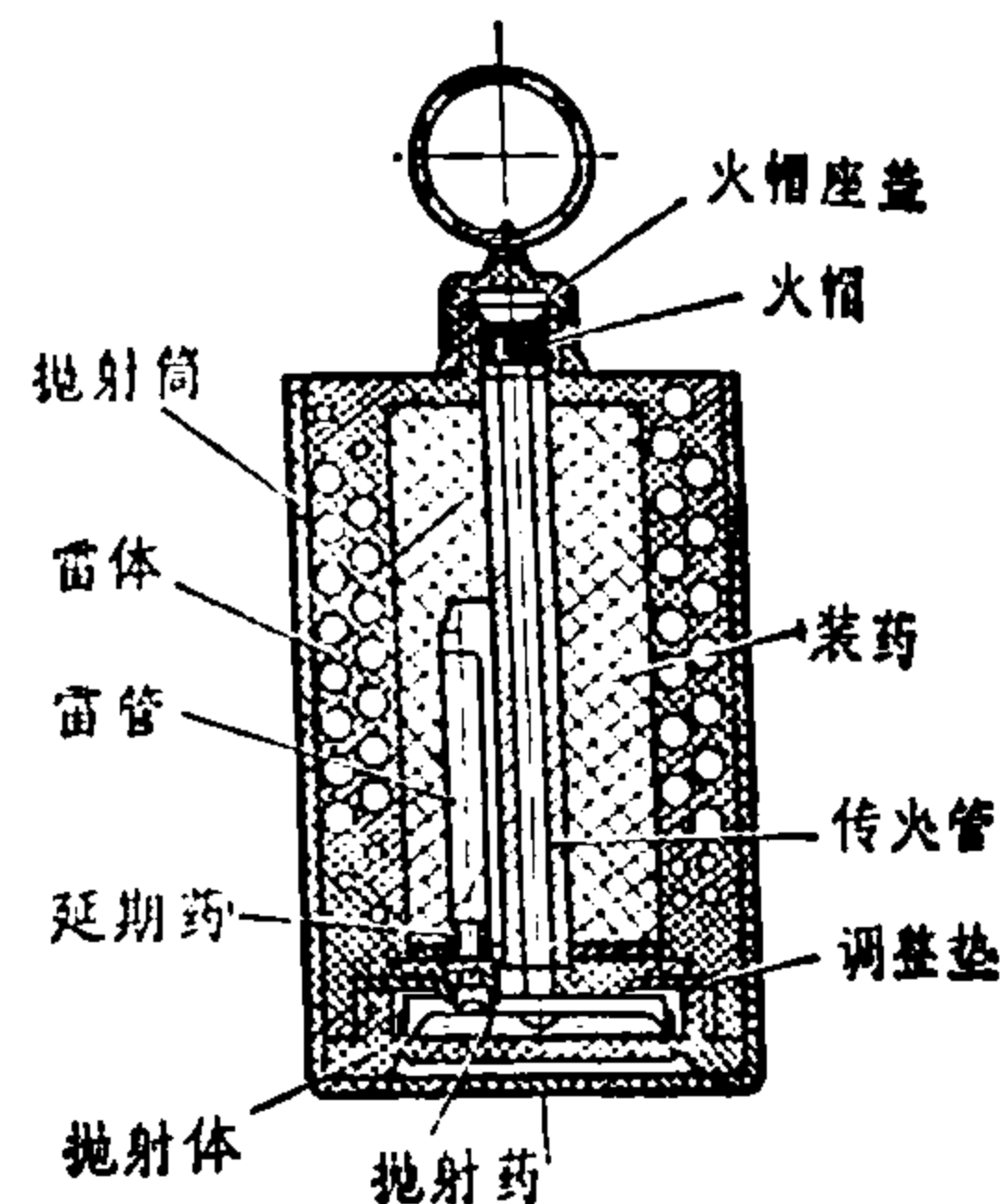
断面图
