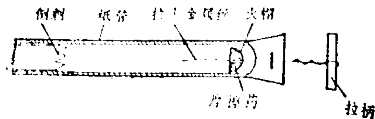
图4 拉火管
