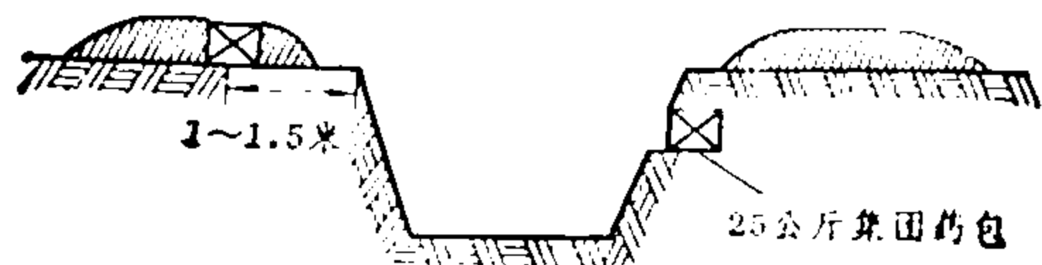
25公斤集团药包放置位置
