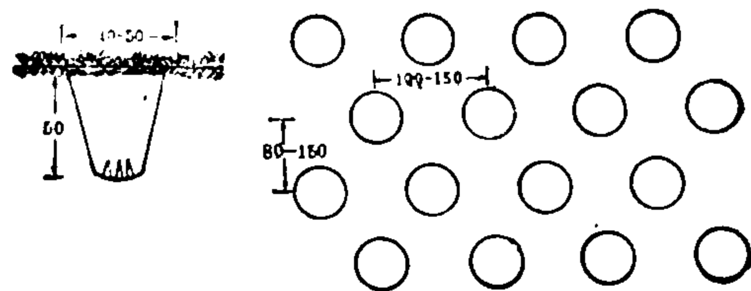
图38 陷阱（单位为厘米）
