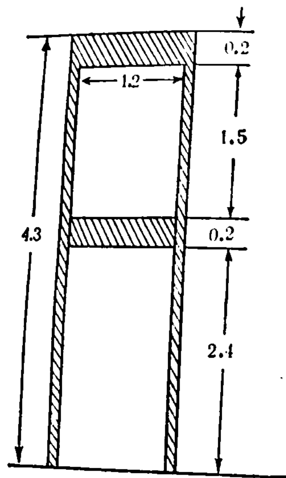
窗口靶 (单位 米)
