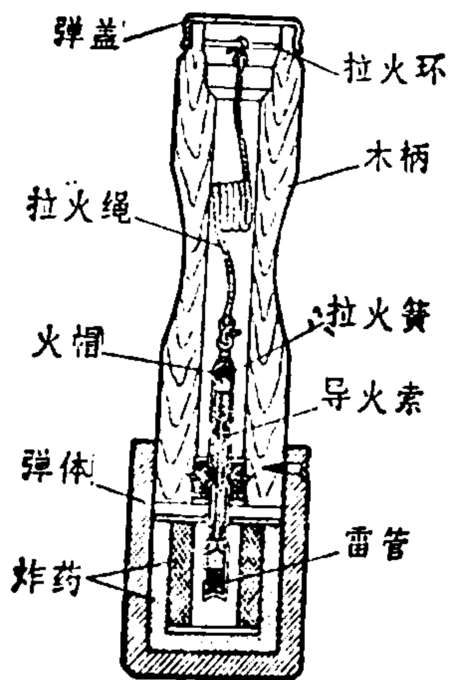
图1 木柄手榴弹剖视图
