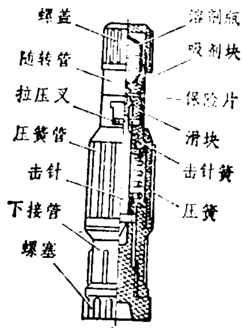
图36 七二式压、拉两用引信
