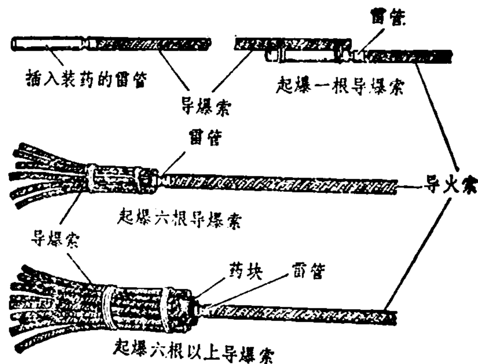
图14 导爆索的起爆
