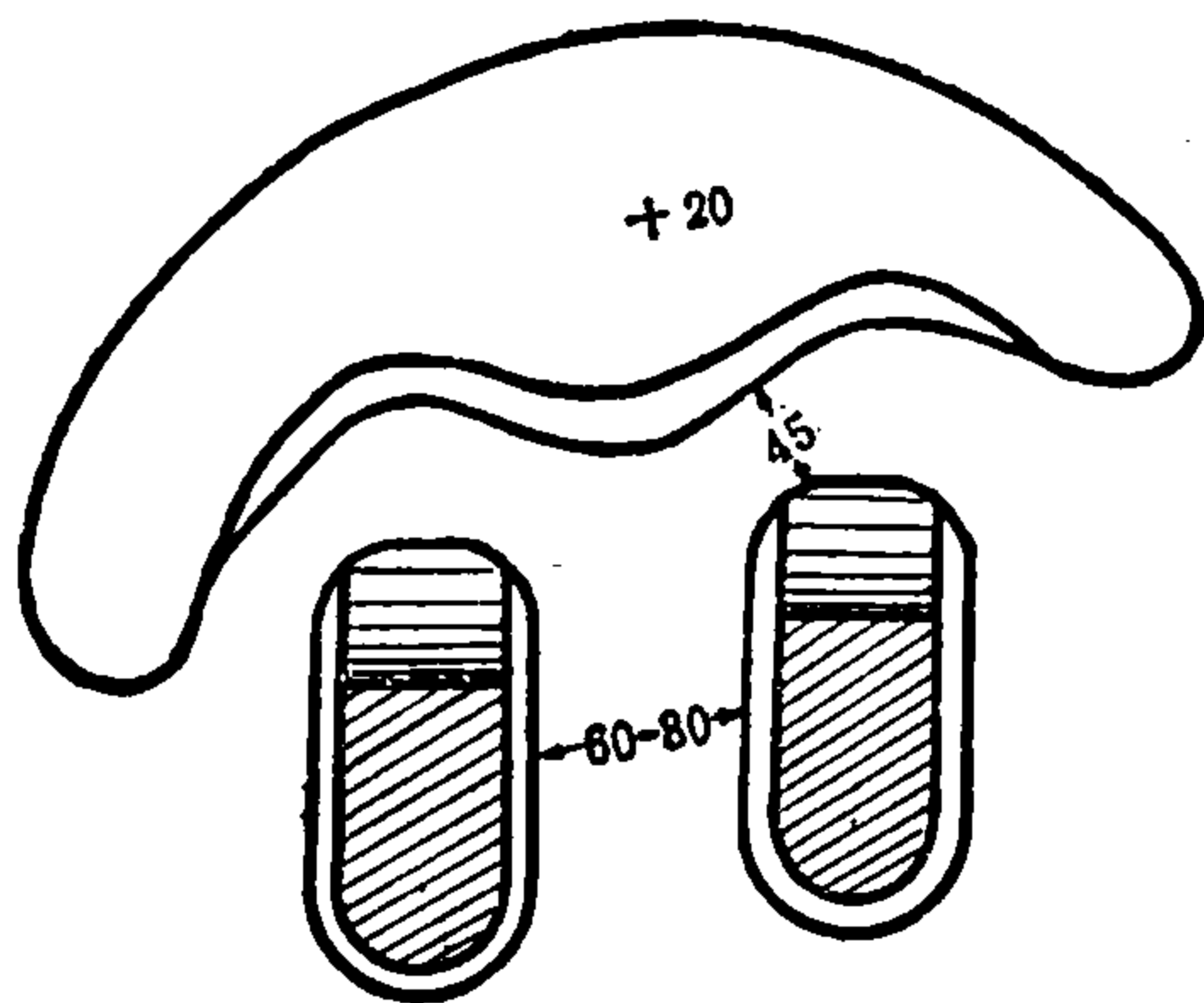
图 7 卧射火箭筒掩体
