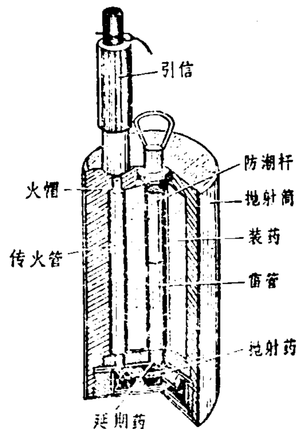
图31 六九式防步兵跳雷
