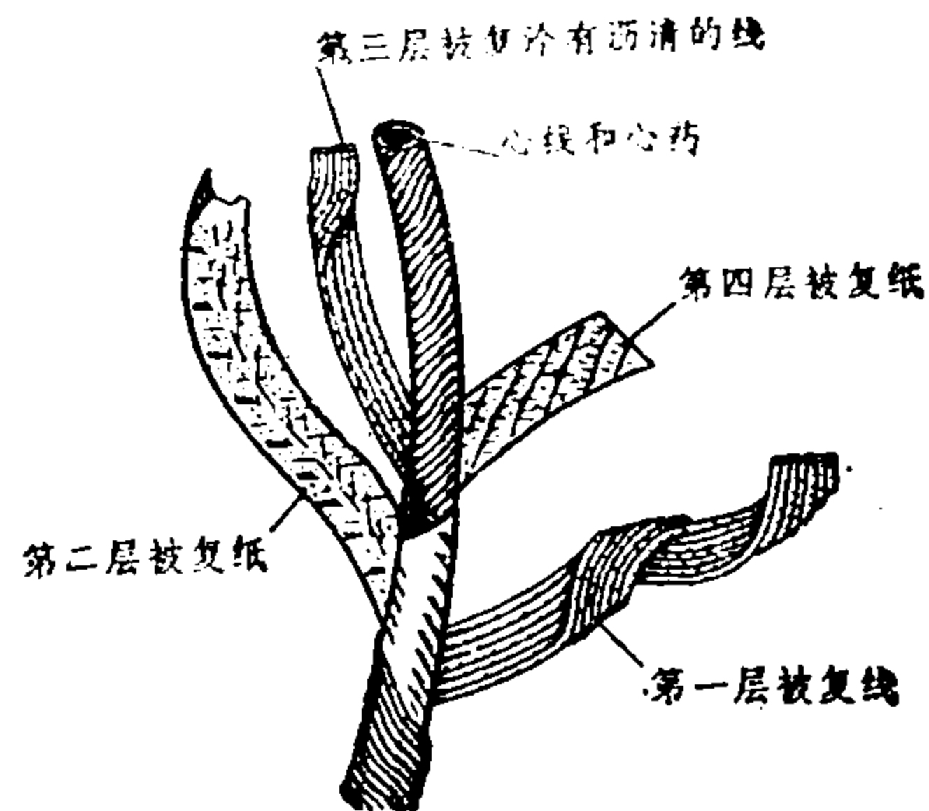
图5 导火索
