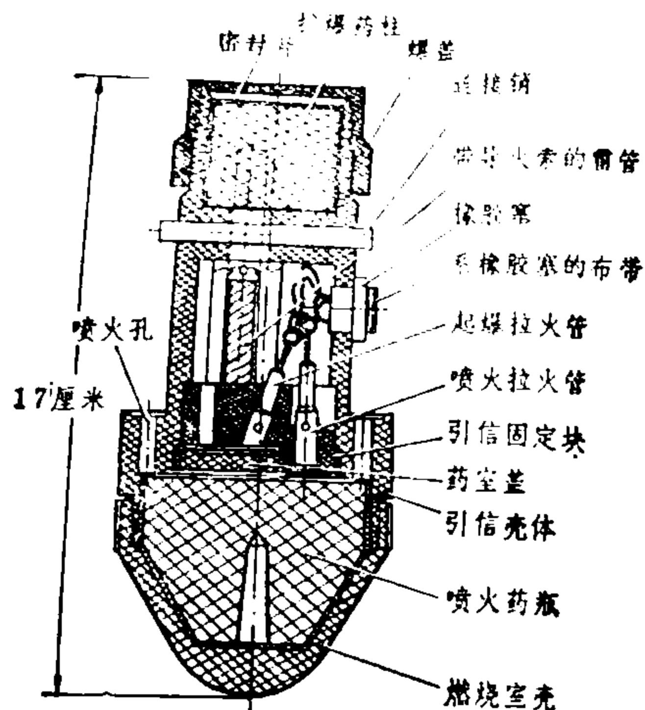
图21 七〇式喷火引信
