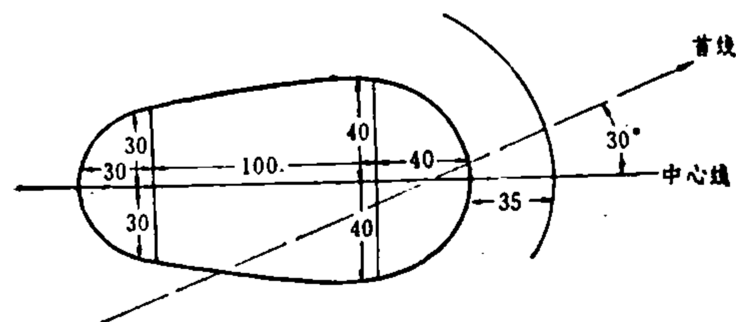
图14 卧射单人掩体经始图（单位为厘米）
