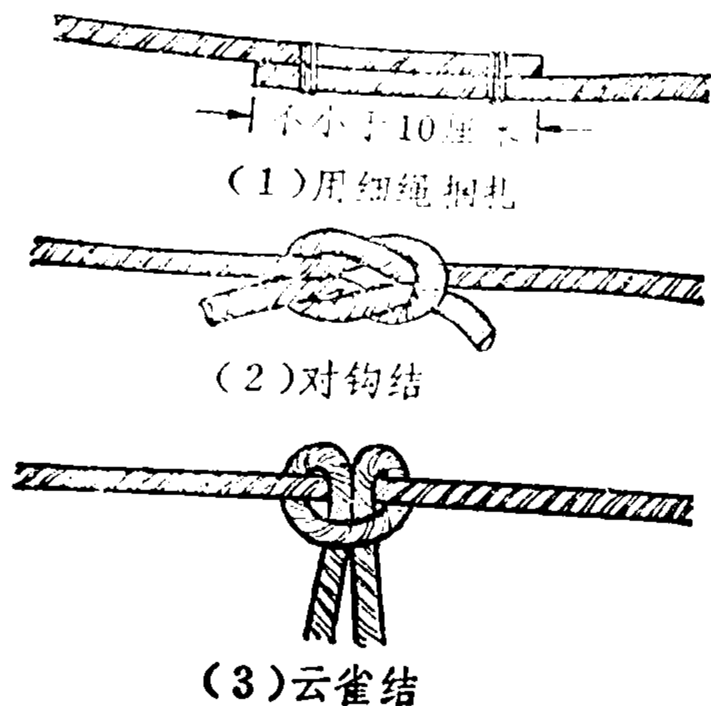
图15 导爆索的接续
