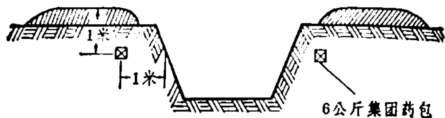
6公斤集团药包放置位置
