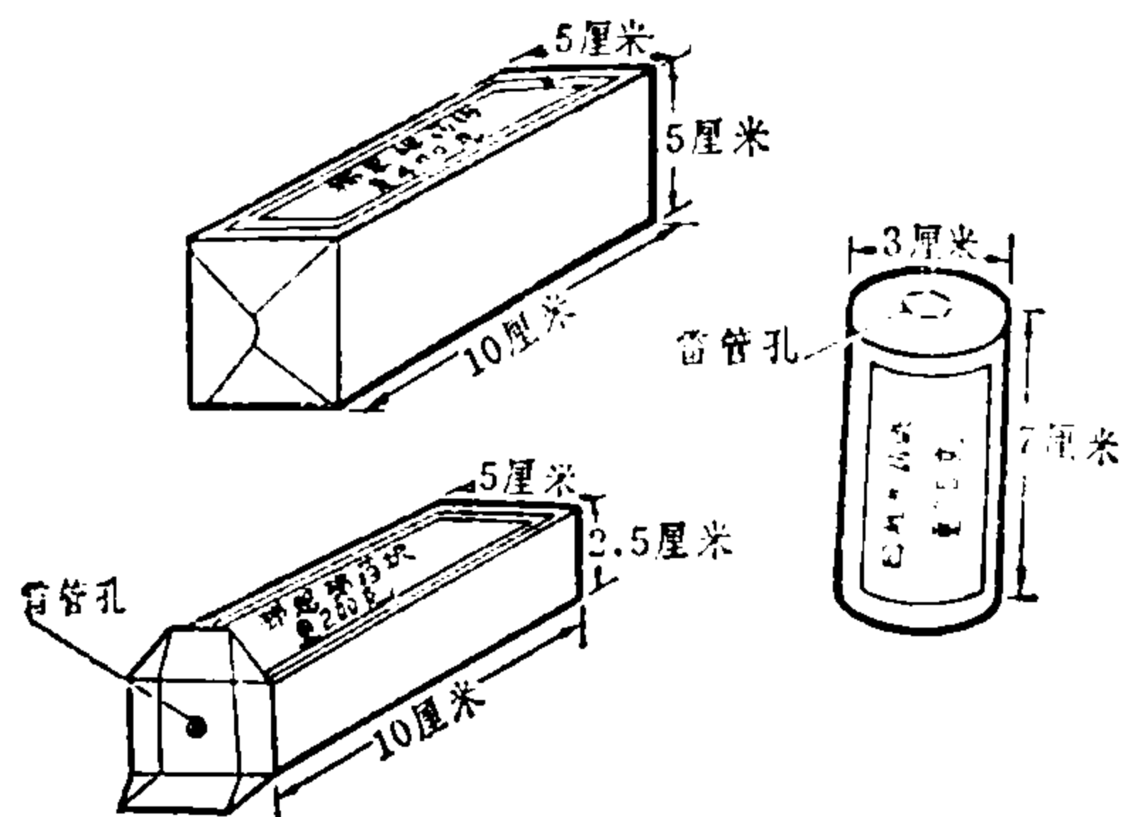
图1 梯恩梯药块
