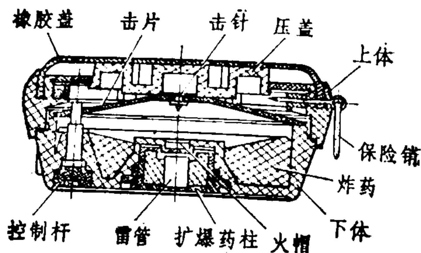
断面图
