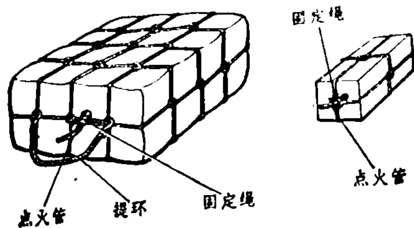
图11 点火管固定在药包上
