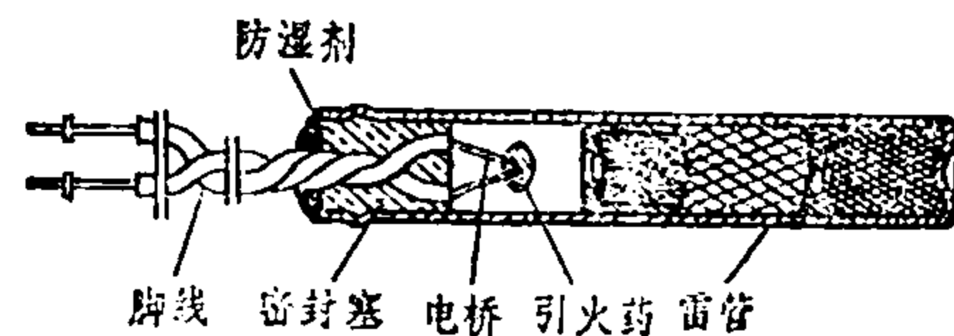
图3 瞬发电雷管
