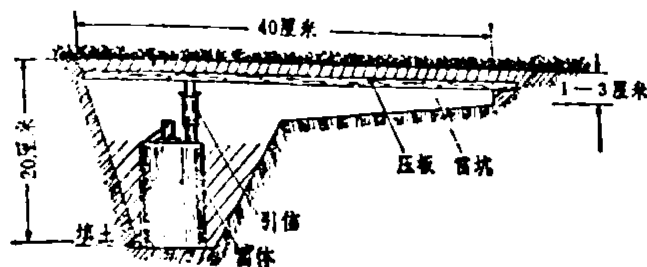
图34 设置成压发状态
