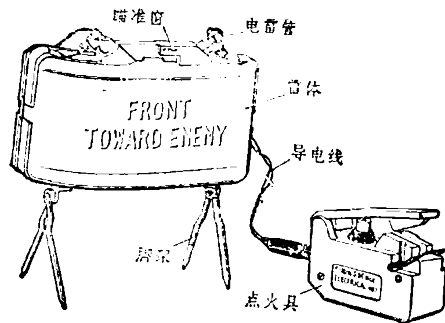
设置图
