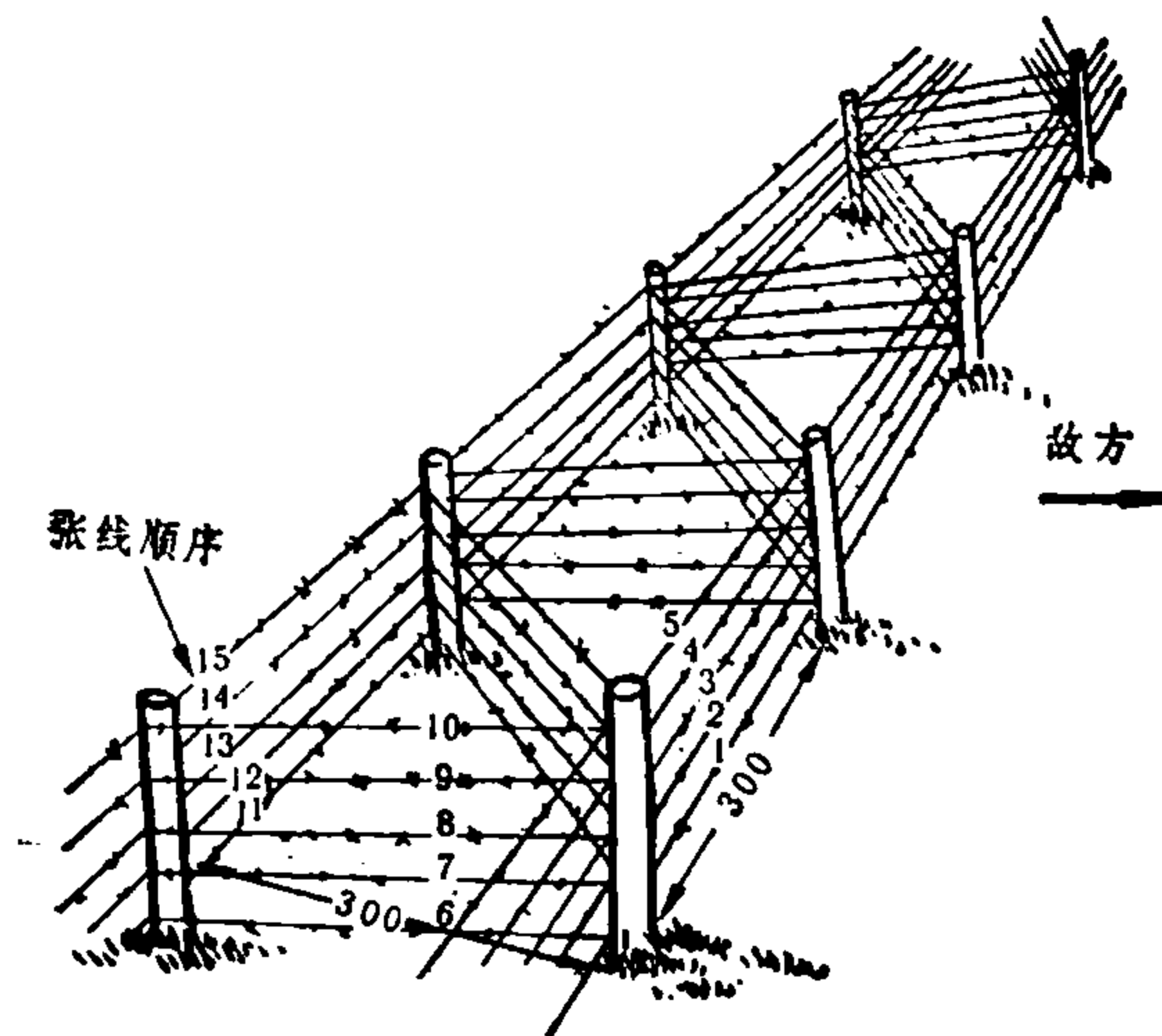
图33 二列桩铁丝网（单位为厘米）
