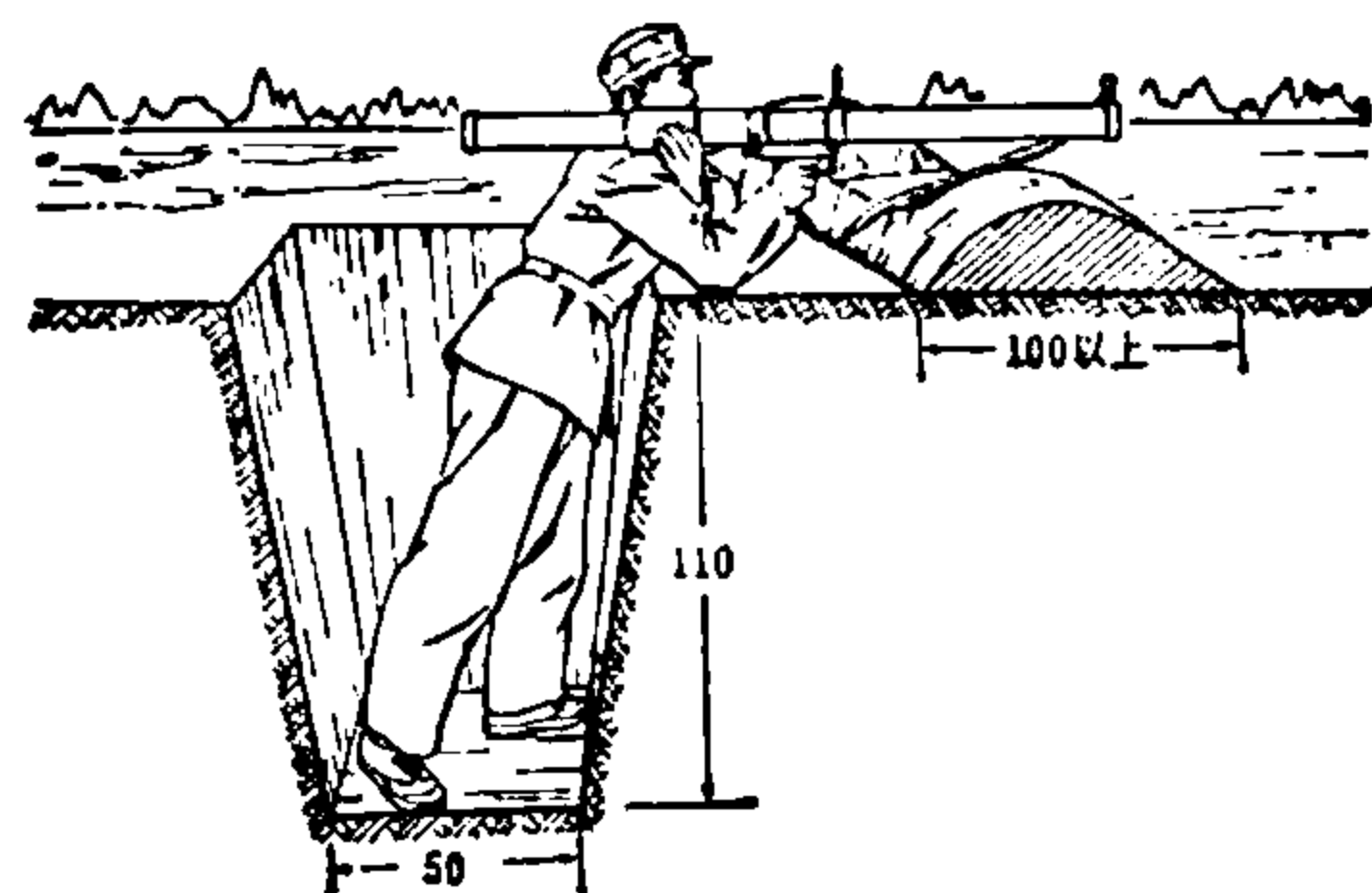
图6 单兵火箭掩体
