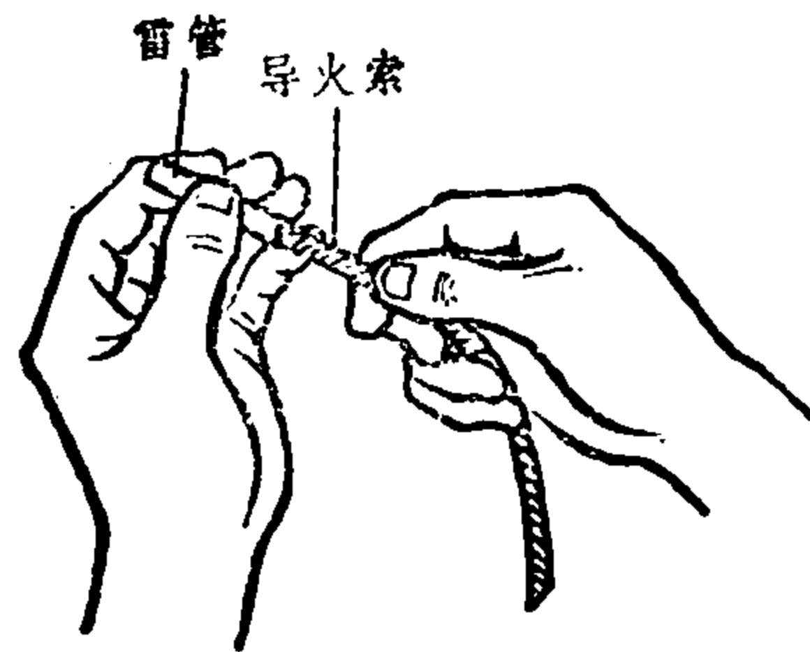
图9 将导火索插入雷管
