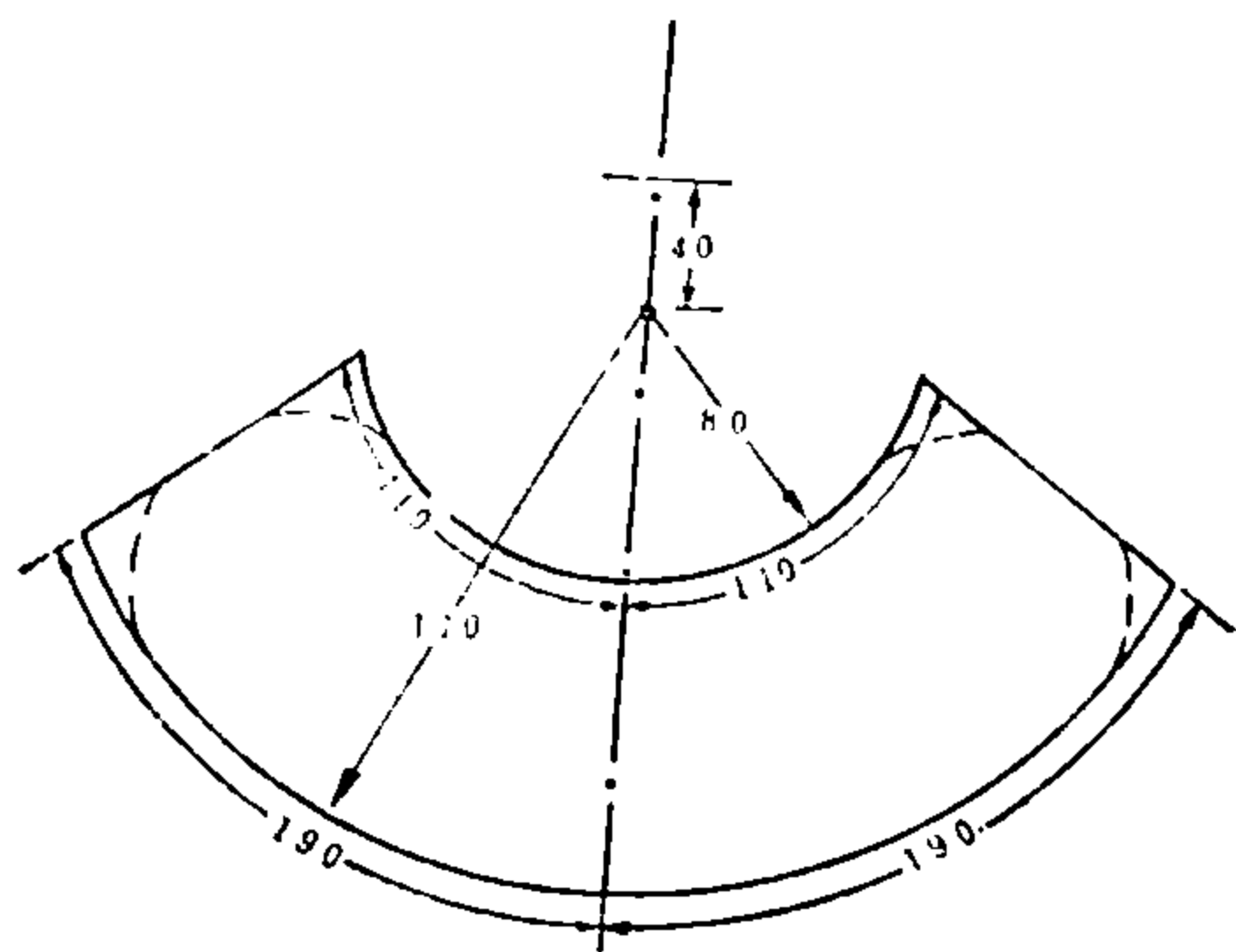
图16 立（跪）射机枪掩体经始图 (单位为厘米)
